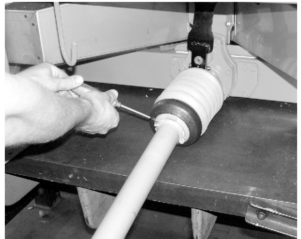
Fig. 14: Bloquer la sécurité de l'arbre de transmission
