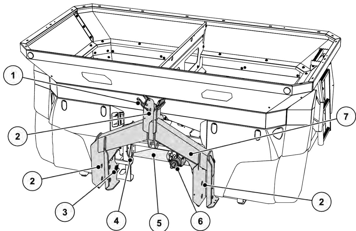
Fig. 6: Aperçu des modules : Face avant
