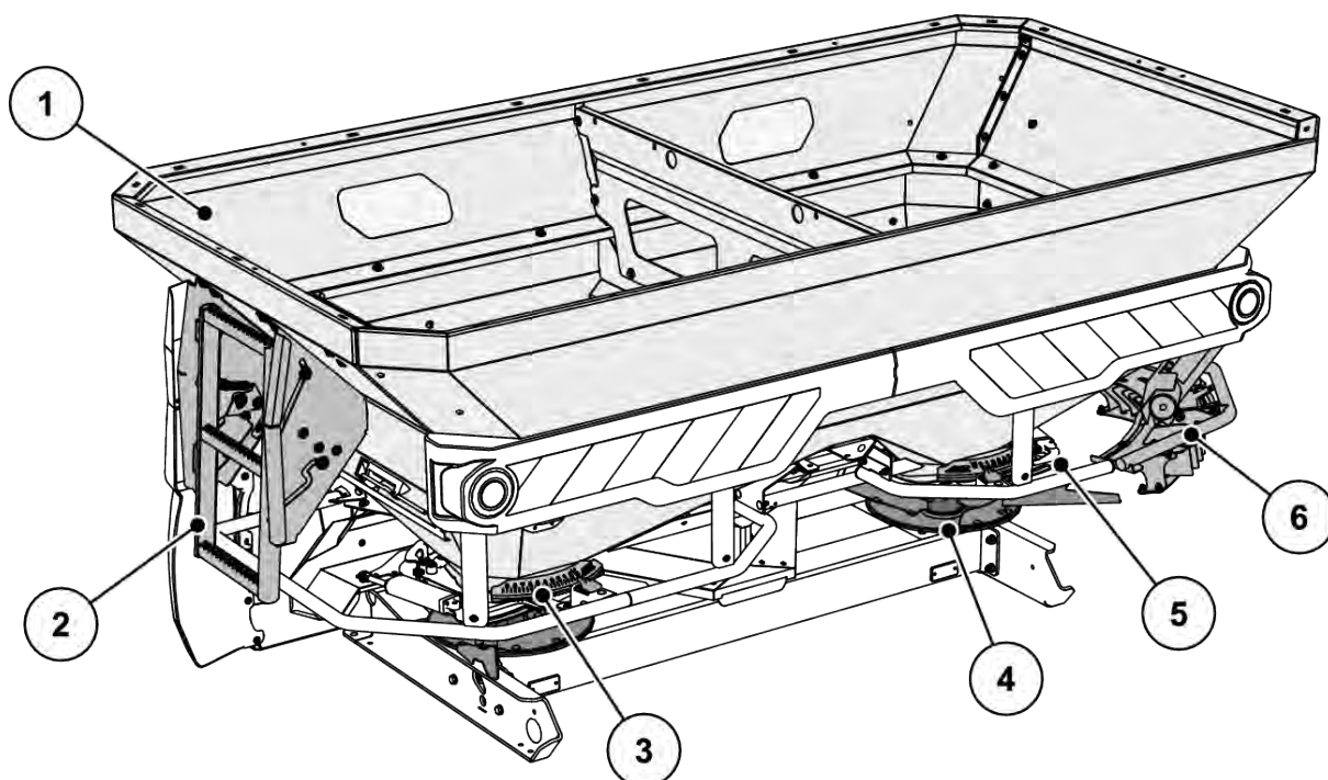
Fig. 5: Aperçu des modules : Face arrière
