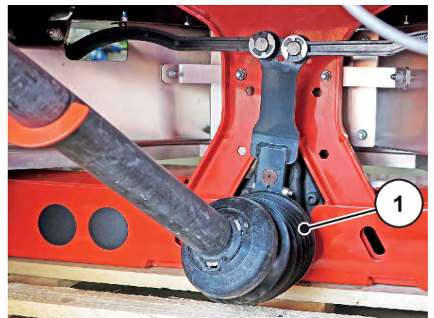
Abb. 4: Gelenkwelle
