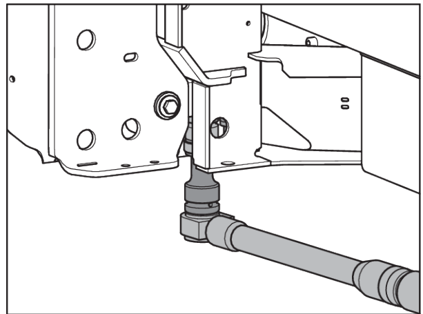
Abb. 47: Befestigung der Wiegezelle (in Fahrtrichtung links)
