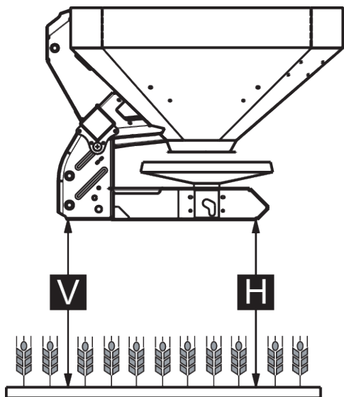
Abb. 19: Maximal zulässige Anbauhöhe in der Normal- und Spätdüngung
