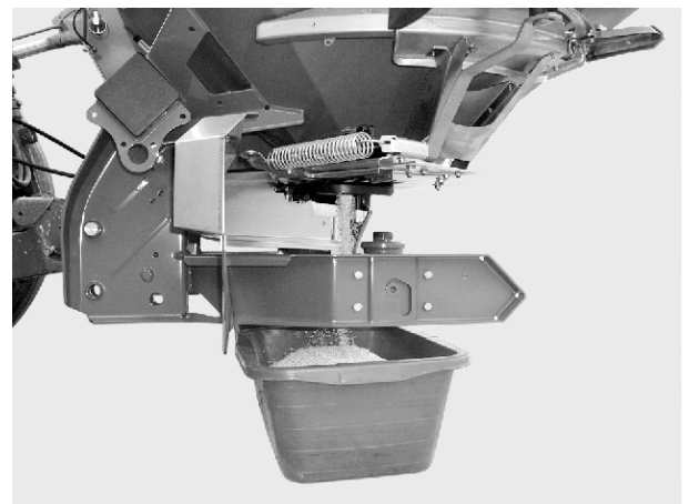
Abb. 40: Abdrehprobe durchführen
