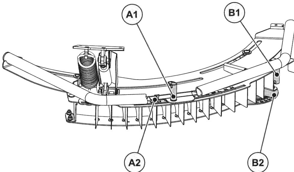
Abb. 24: TELIMAT Einrichtung einstellen
