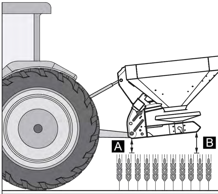
Abb. 22: Anbau der Maschine an den unteren Unterlenkerkuppelpunkt
