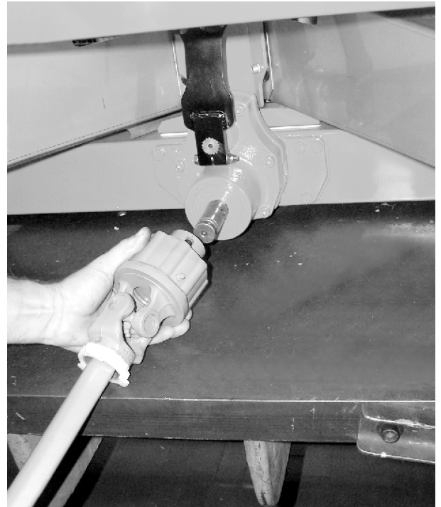
Abb. 12: Gelenkwelle auf Getriebezapfen aufstecken
