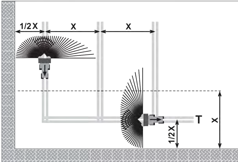
Abb. 32: Grenzstreuen
