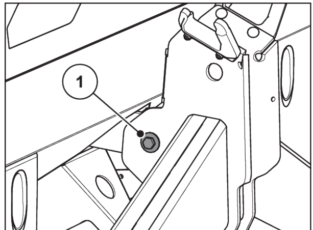
Abb. 48: Befestigung des Zugstabes am Wiegerahmen
