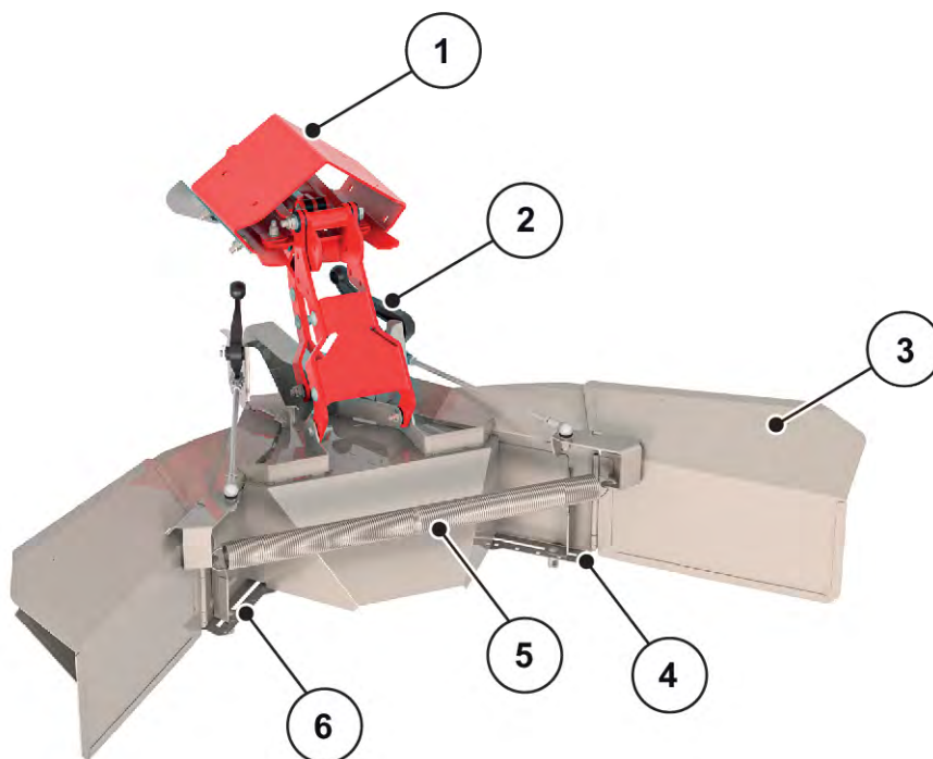
Рис. 29: Налаштування обмежувача ширини розкидання
