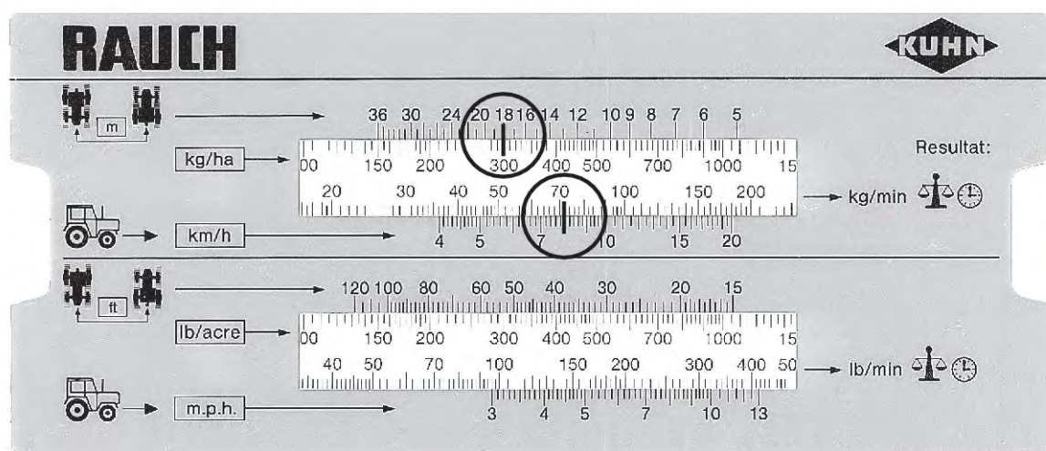
Рис. 41: Шкала для визначення заданої норми виходу добрива за хвилину
