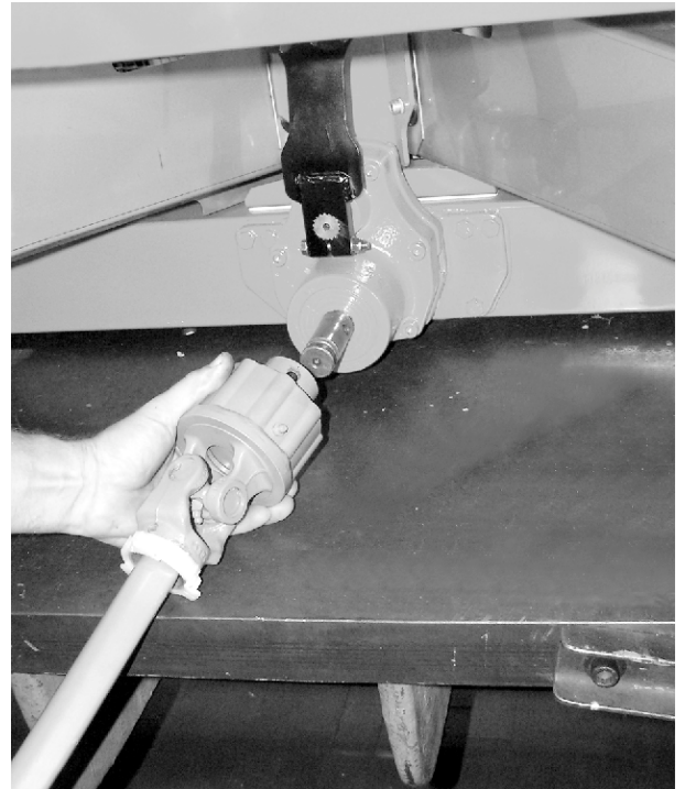
Рис. 12: Встановлення карданного вала на цапфу редуктора
