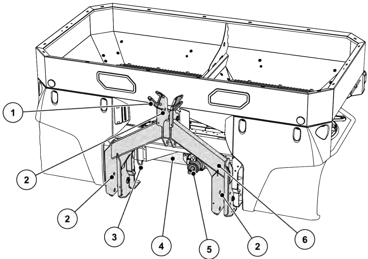
Рис. 6: Огляд конструкційних вузлів. Вигляд спереду
