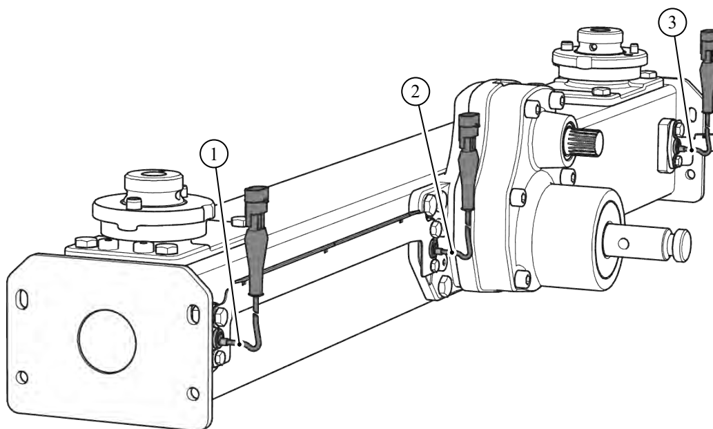
Рис. 8: Регулювання потоку матеріалу шляхом вимірювання крутного моменту розкидальних дисків
