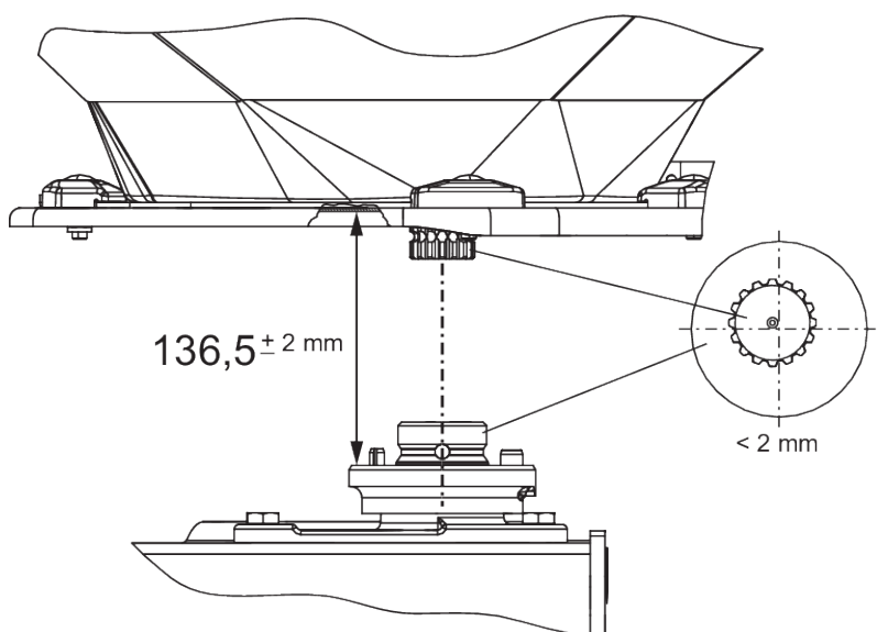
Рис. 59: Перевірка втулки положення розкидального диска
