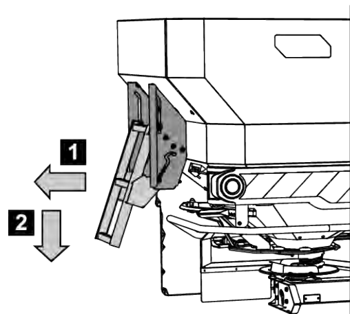
Рис. 50: Розкладання підніжки
