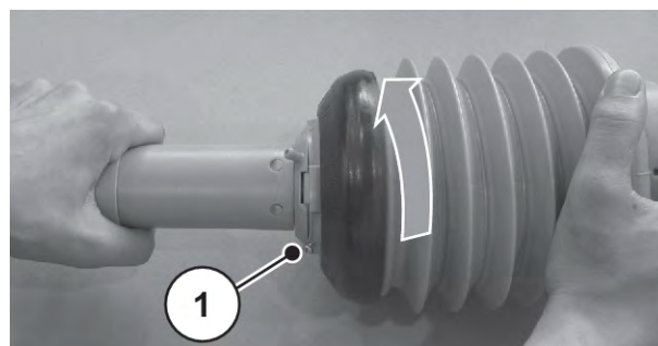
Рис. 11: Ослаблення кожуха карданного вала
