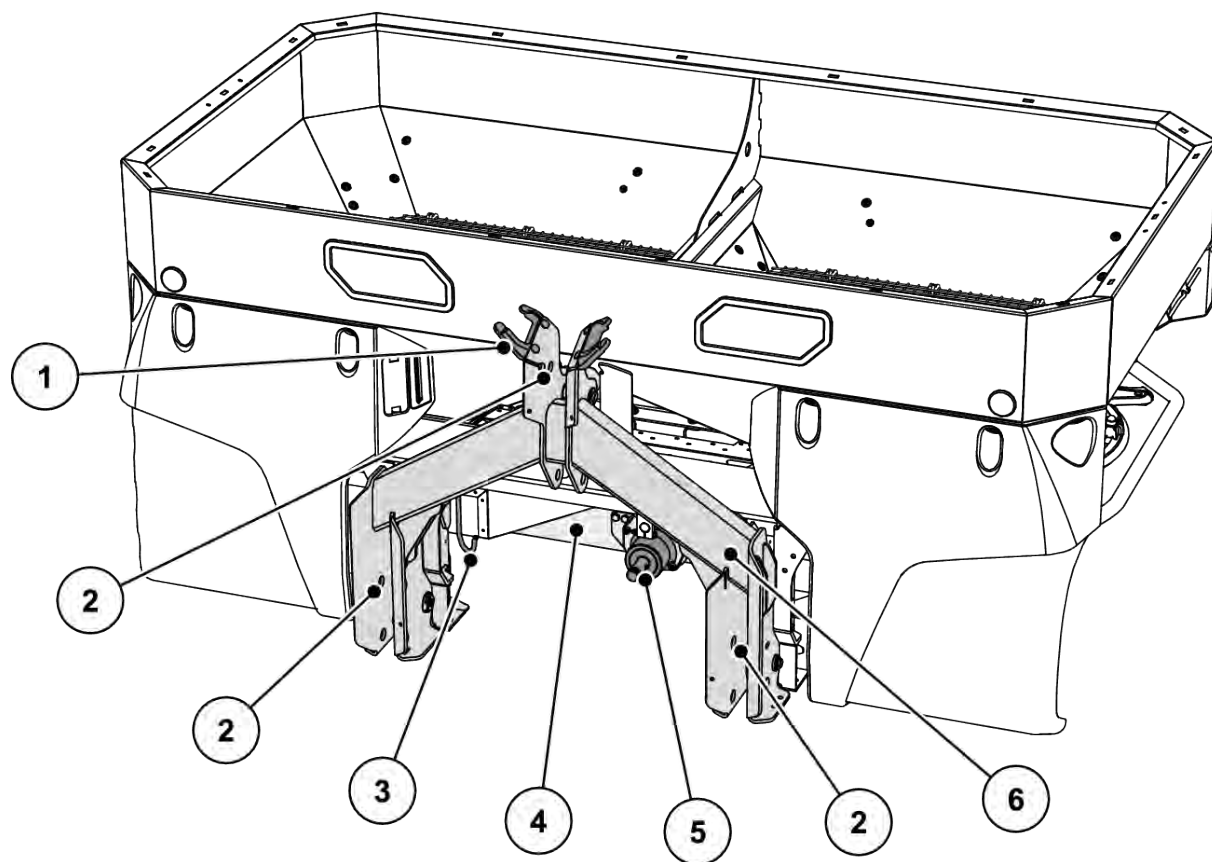
Kuva 6: Rakenneryhmäkuva: Etupuoli
