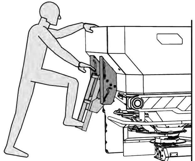
Kuva 48: Tikkaat ilman säiliön suojapeitettä
