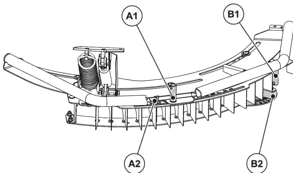
Kuva 30: TELIMAT-laitteen asettaminen
