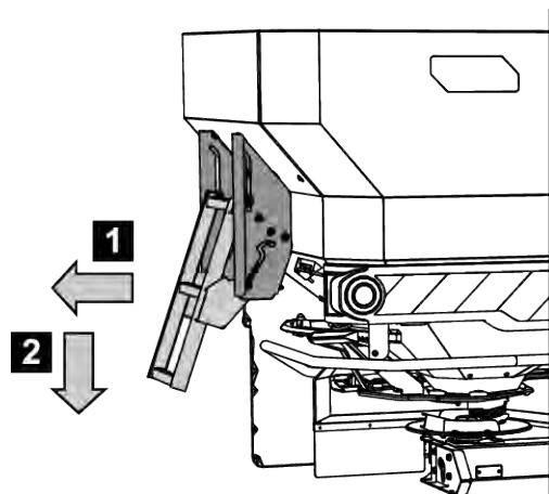
Kuva 50: Tikkaiden taittaminen auki
