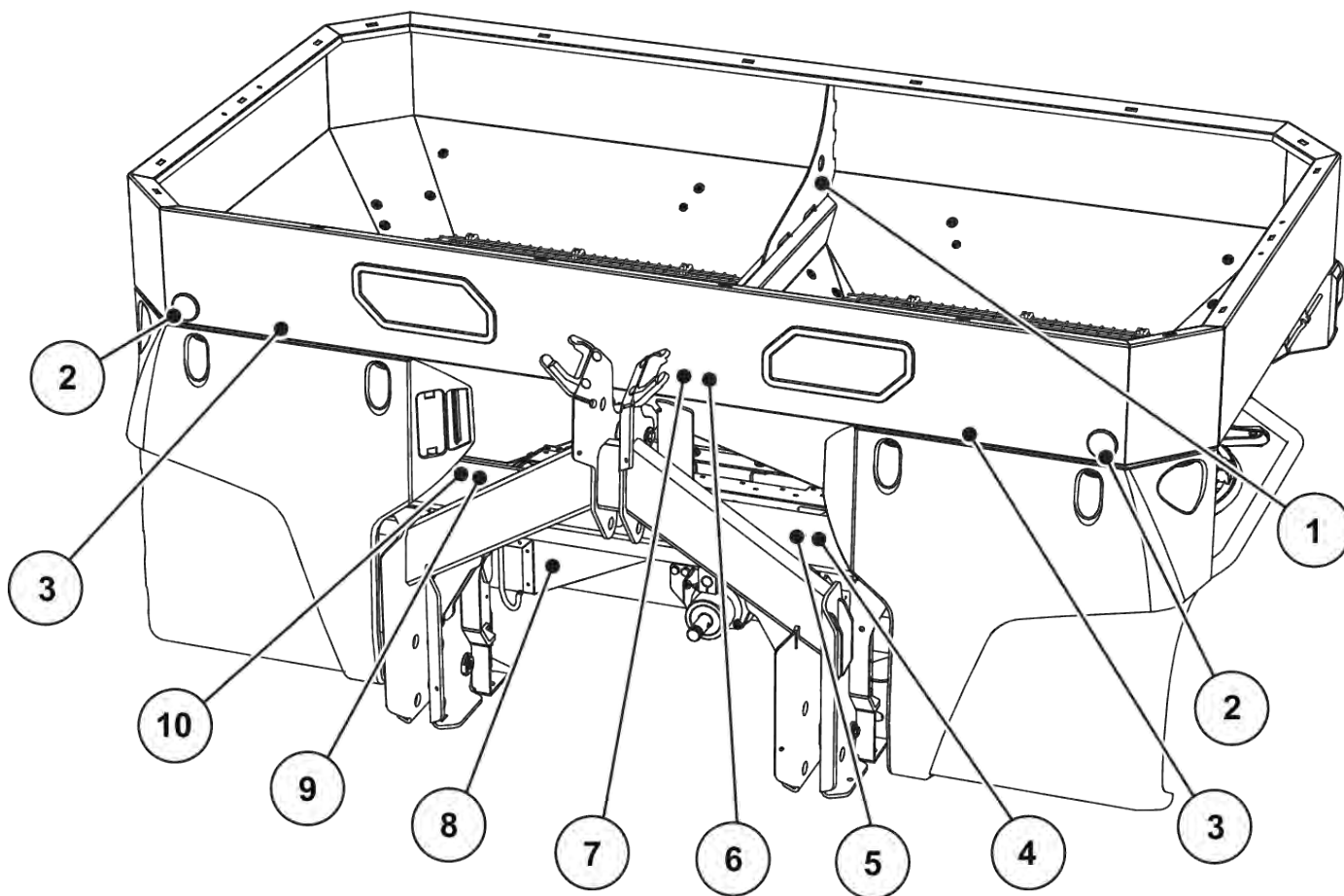
Kuva 2: Suojalaitteet, varoitus- ja ohjetarrat, etuosa
