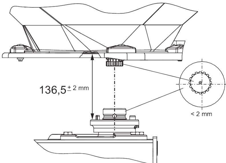
Att. 59: Izkliešanas diska rumbas pozīcijas pārbaude
