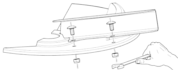
Att. 63: Atbrīvojiet izmešanas spārniņu skrūves.
