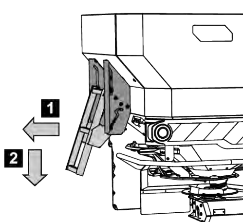
Att. 50: Kāpņu atliekšana
