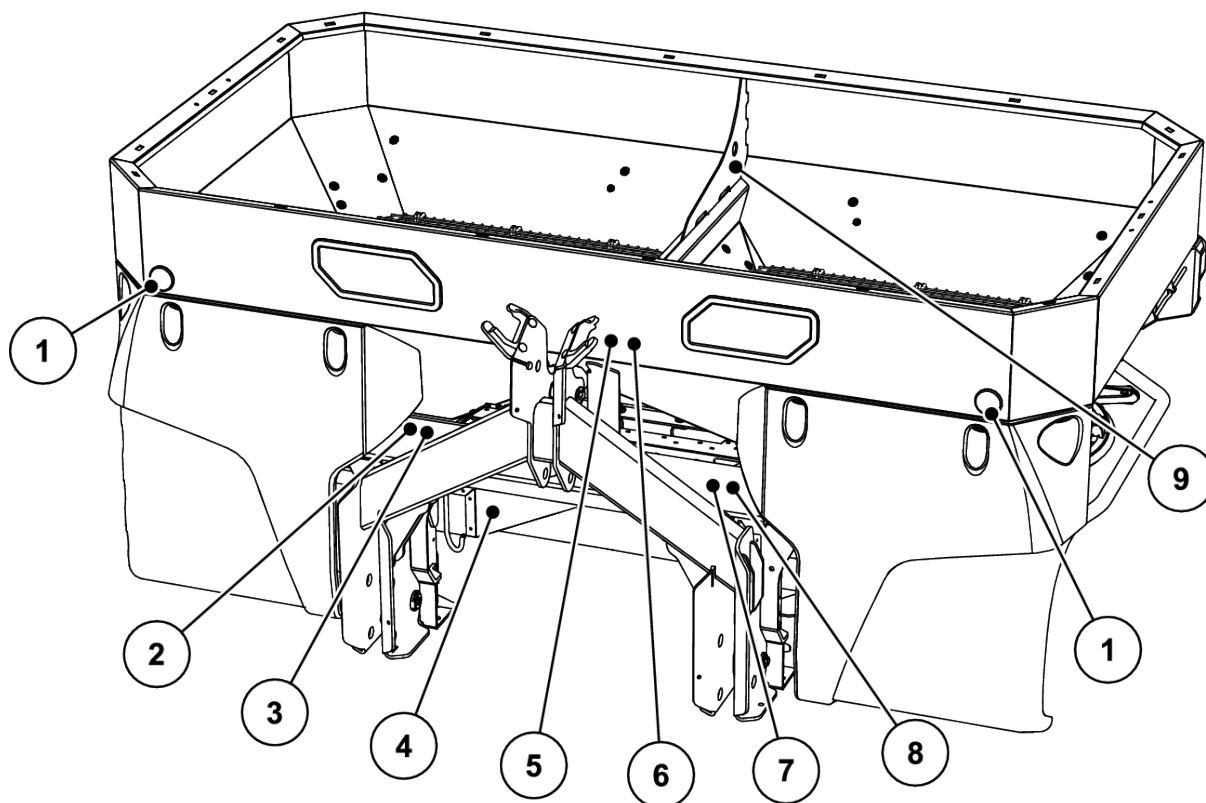
Att. 4: Drošības ierīces, brīdinājumu un instrukciju norādījumu uzlīmes, priekšpuse
