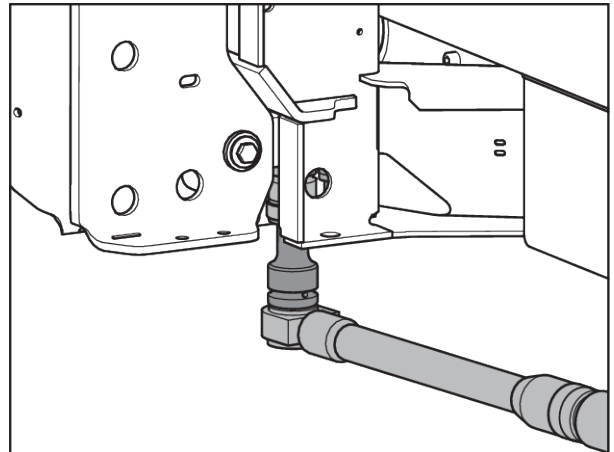
Att. 52: Tenzodevēja piestiprināšana (braukšanas virzienā kreisajā pusē)
