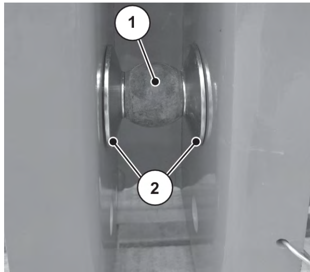
Att. 17: Distances starpliku pozīcija, uzkabīnot mašīnu
