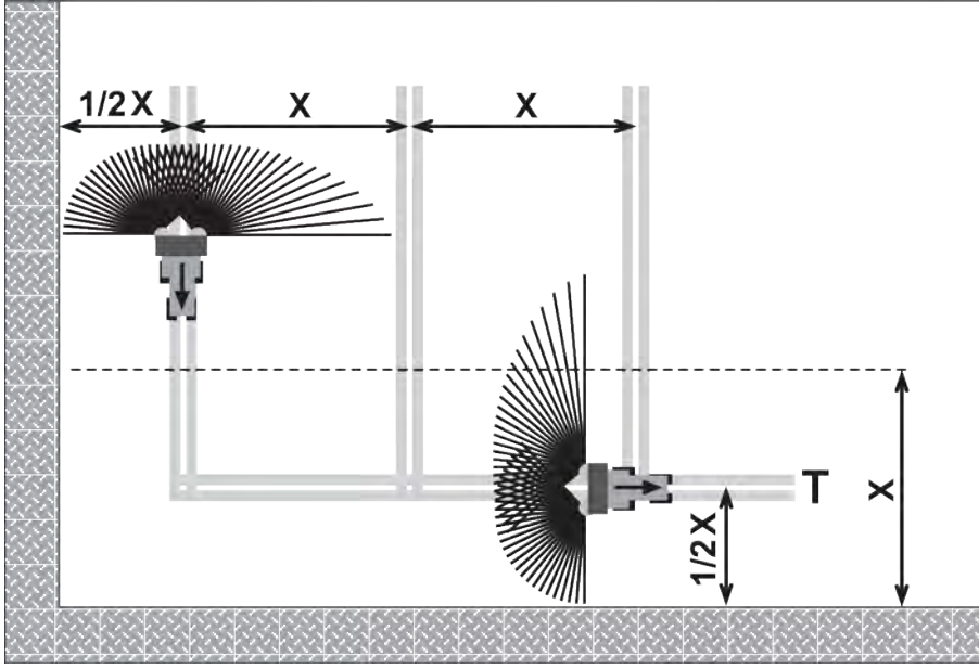
Şek. 37: Sınır serpme
