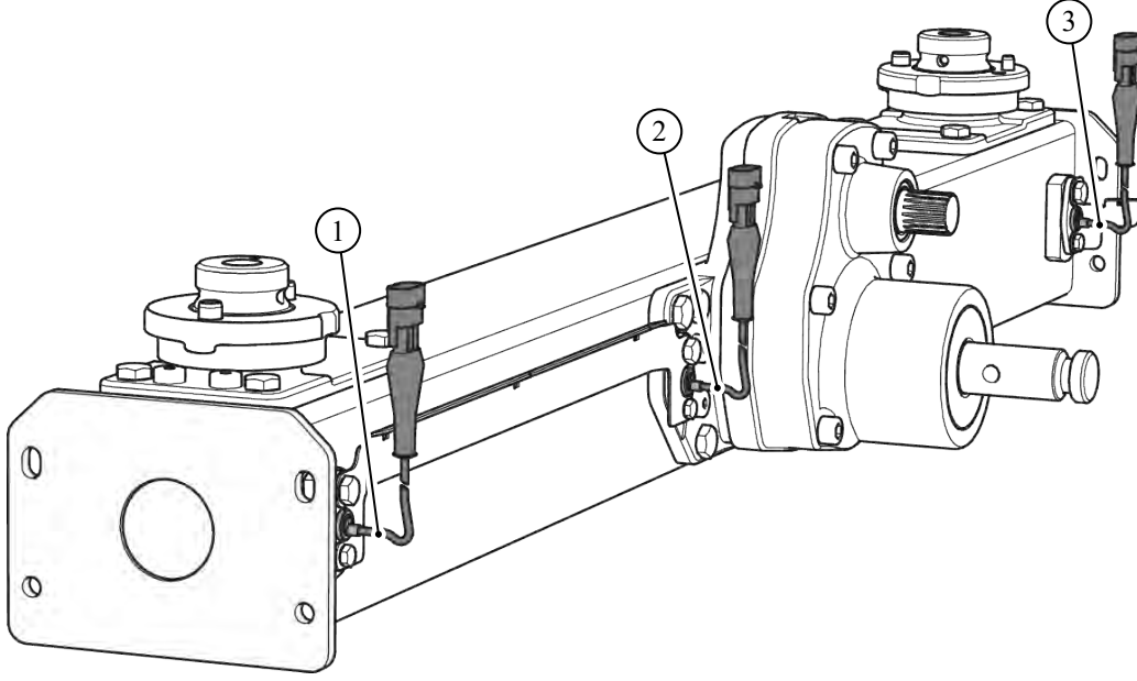
Şek. 8: Fırlatma disklerinin hızının ölçülmesi yoluyla kitle akışı denetimi
