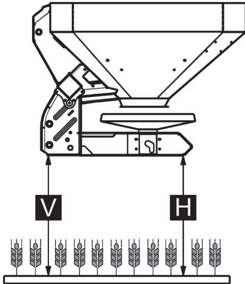
Şek. 19: Normal ve geç gübrelemede izin verilen azami montaj yüksekliği
