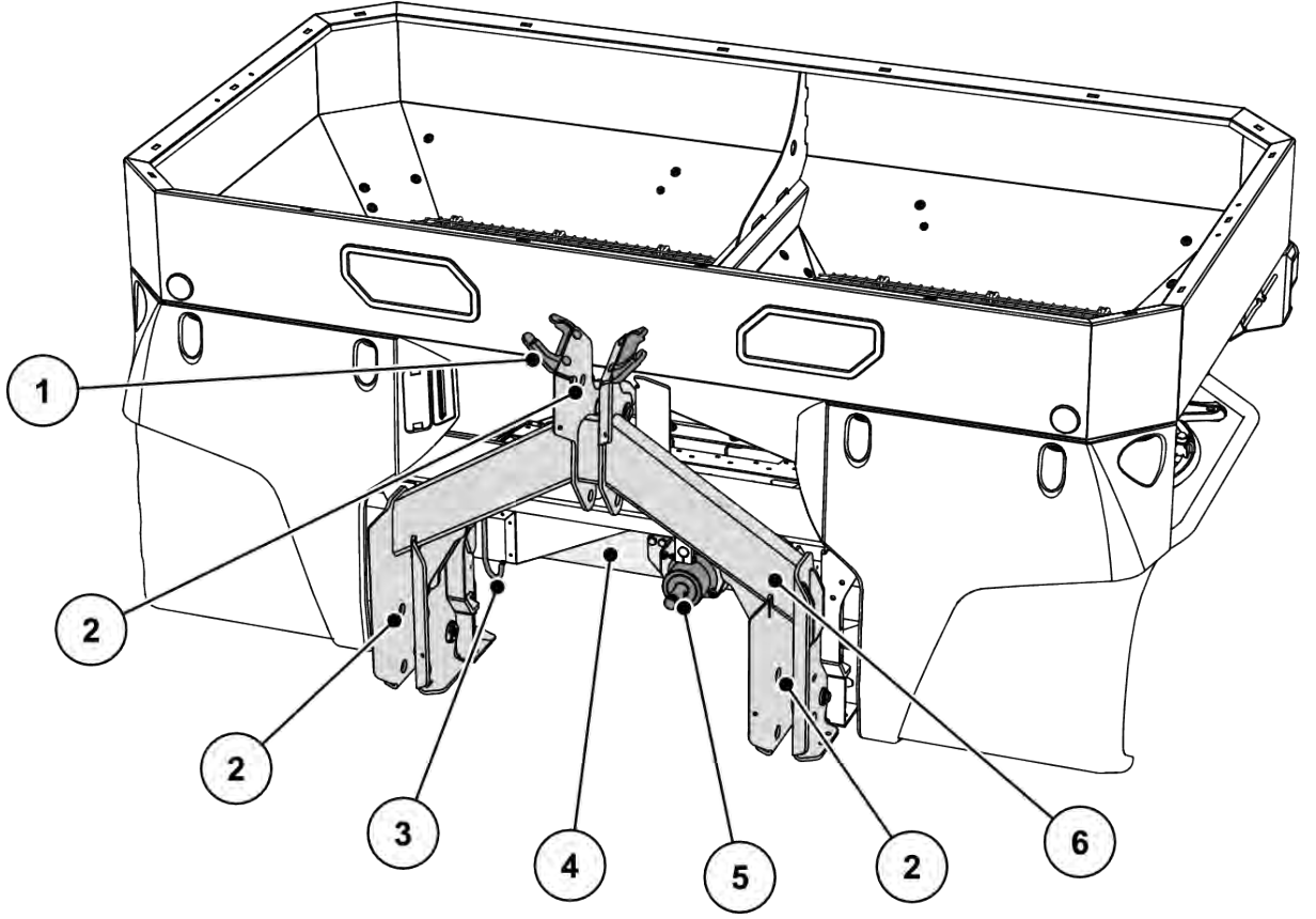
Şek. 6: Yapı gruplarına genel bakış: Ön taraf
