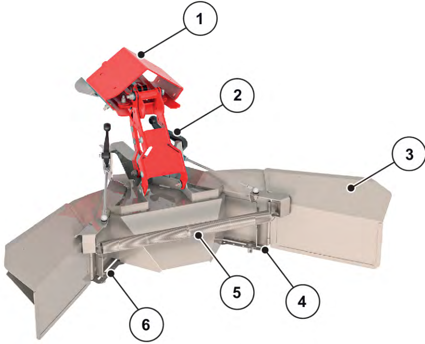
Şek. 29: Sınır serpme tertibatının ayarı
