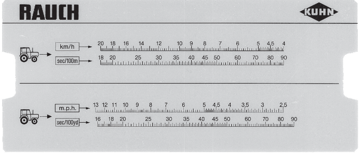
Şek. 40: Kesin sürüş hızının belirlenmesinde kullanılan skala
