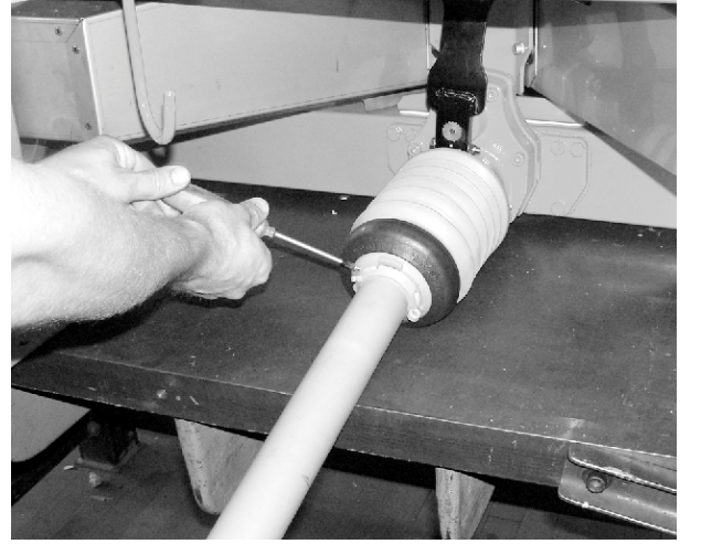
Şek. 15: Tahrik mili korumasını sabitleyin
