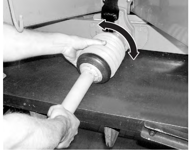
Şek. 14: Tahrik mili korumasını yerleştirin
