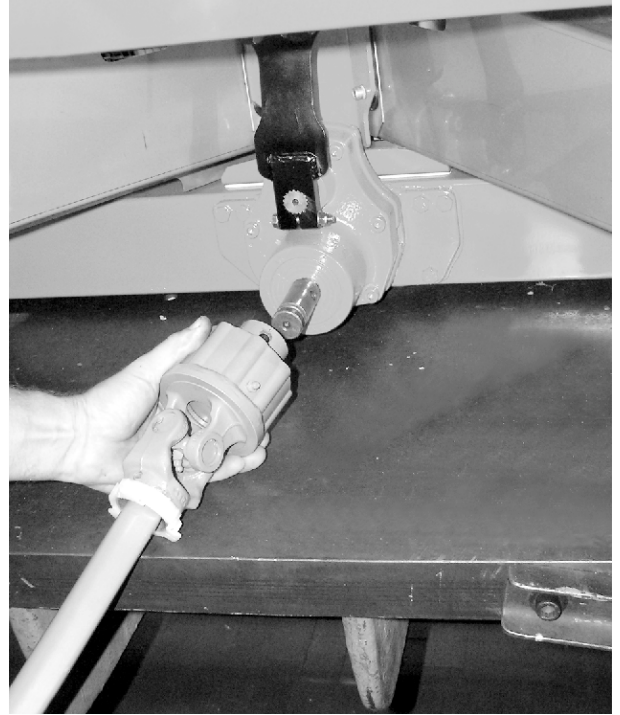
Şek. 12: Tahrik milini şanzıman miline monte edin
