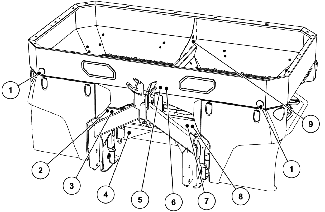
Şek. 4: Koruma donanımları, Uyarı ve talimat etiketleri, ön taraf
