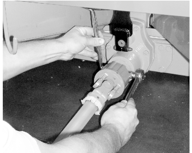
Şek. 13: Tahrik milini sabitleyin
