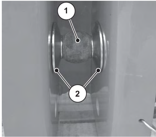
Şek. 17: Makine bağlantısında ara disklerin konumu
