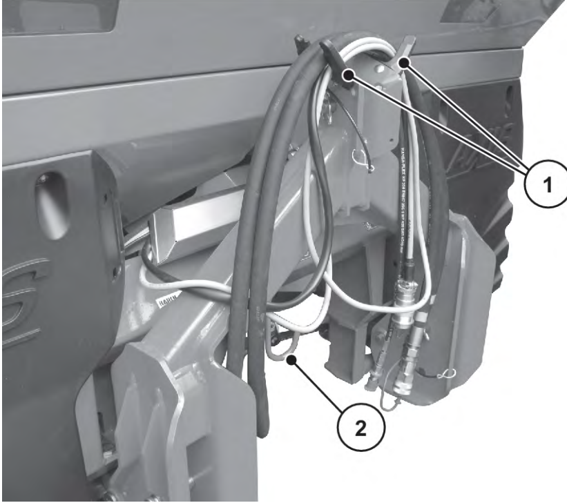
Şek. 47: Kablo ve hidrolik hortumları koyma yeri
