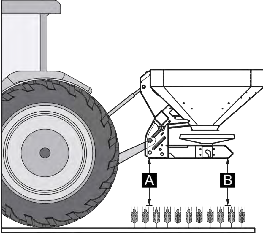
Şek. 20: Normal gübrelemede montaj konumu ve yüksekliği
