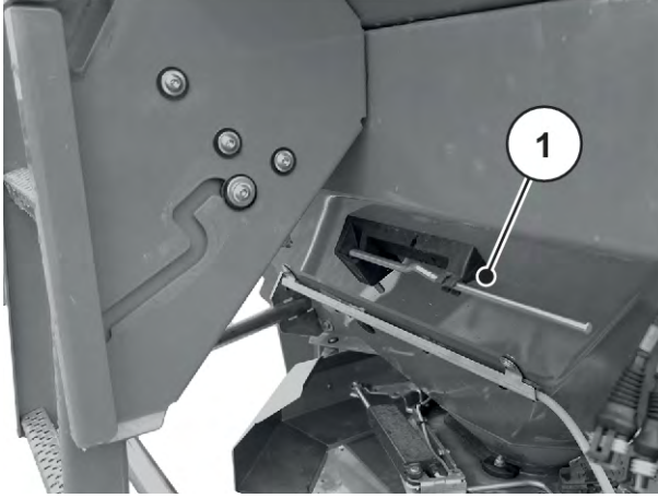
Şek. 32: AXIS xx.2 için ayar kolunun konumu
