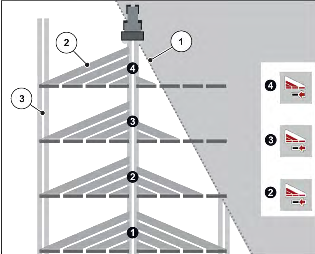
Şek. 39: Kısmi genişlik anahtarlama örneği
