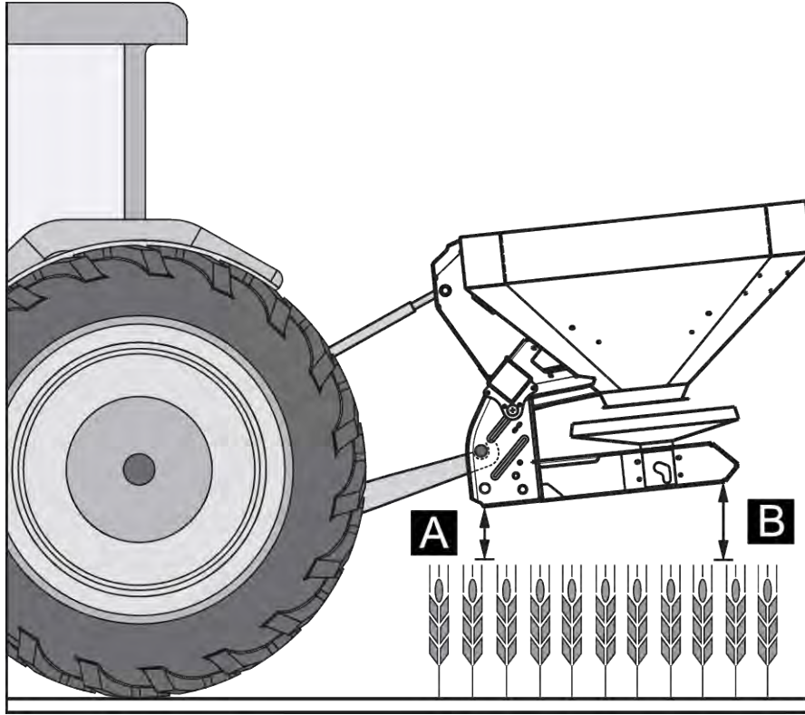
Şek. 21: Geç gübrelemede montaj konumu ve yüksekliği
