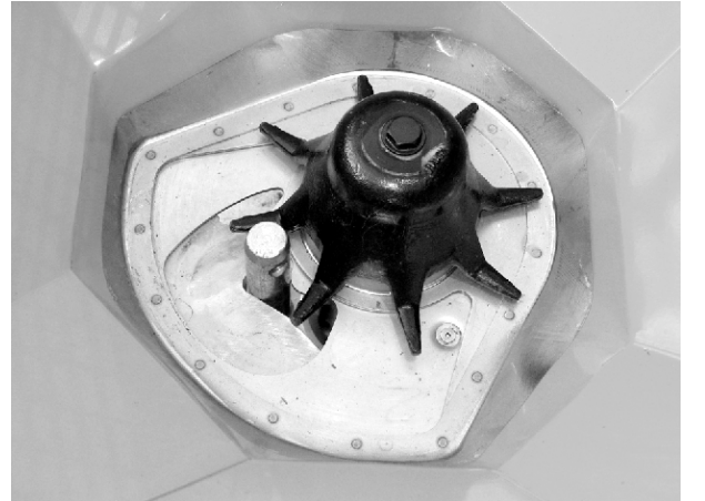
Şek. 65: Dozaj açıklığındaki alt bağlantı pimi
