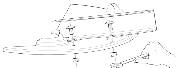
Sl. 63: Zrahljajte vijake trosilnih lopatic.
