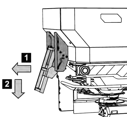
Sl. 50: Izvlek lestve
