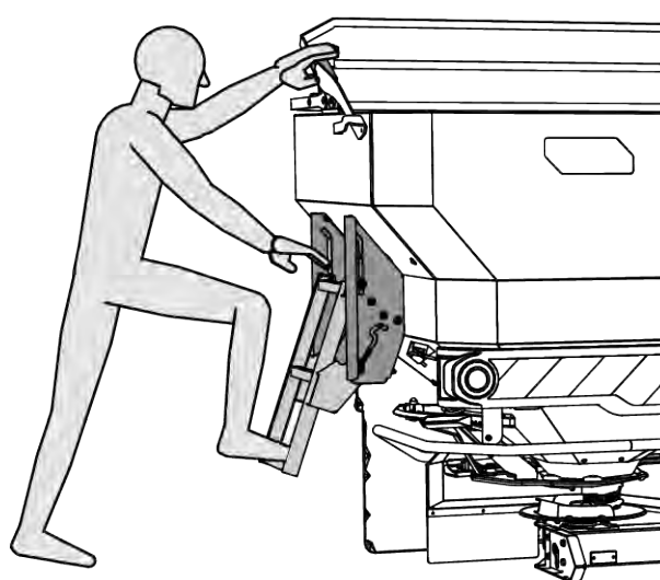
Sl. 49: Lestev s pokrivno ponjavo posode
