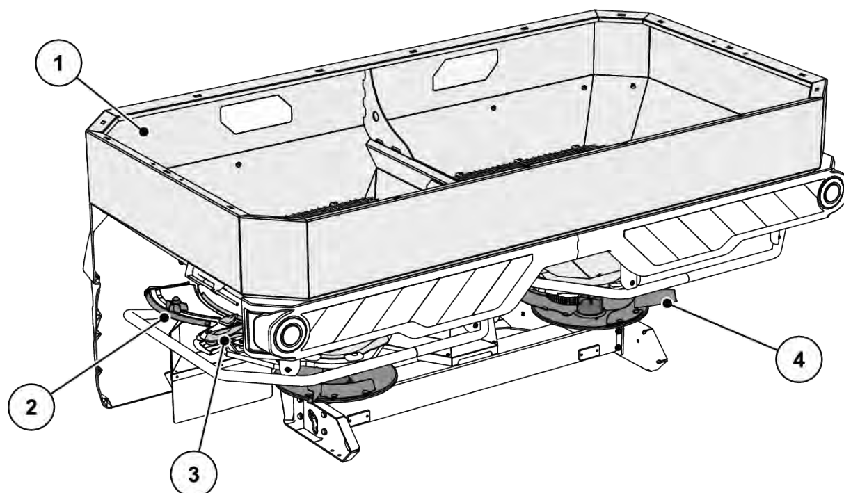
Obr. 7: Prehľad konštrukčných skupín: Zadná strana
