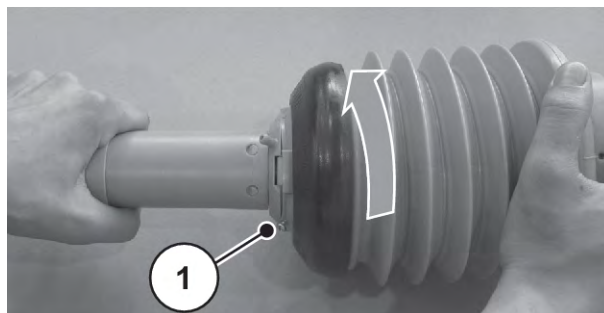
Obr. 11: Uvoľnenie krytu kĺbového hriadeľa
