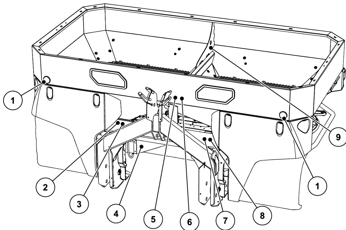
Obr. 4: Ochranné zariadenia, nálepky s varovnými upozoreniami a pokynmi, predná strana
