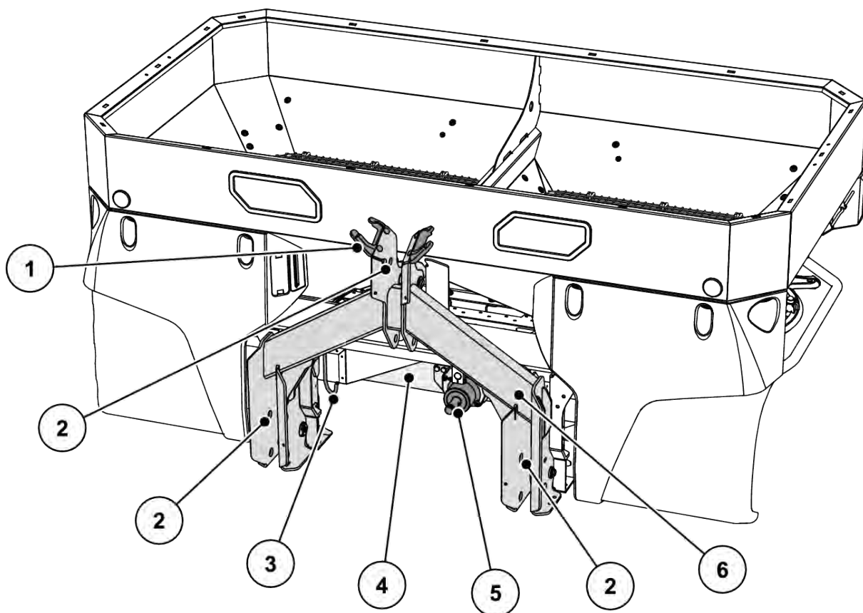
Obr. 6: Prehľad konštrukčných skupín: Predná strana
