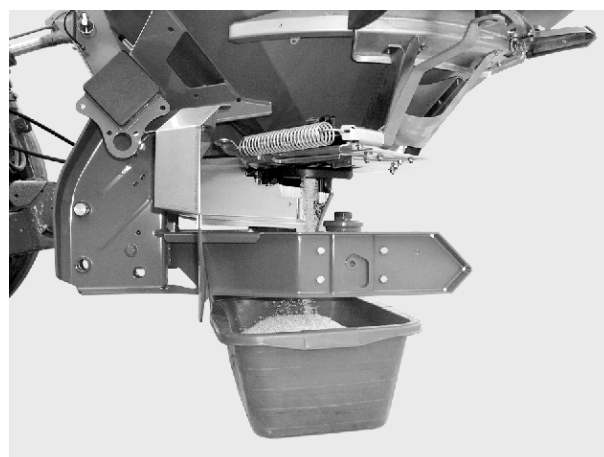
Obr. 45: Vykonanie skúšobného rozmetávania
