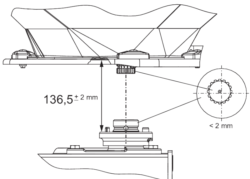
Obr. 59: Kontrola polohy náboja rozmetávacieho disku
