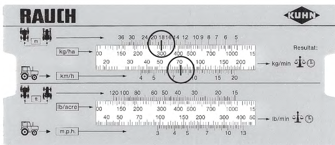
Obr. 41: Stupnica na zistenie požadovaného výstupného množstva za minútu
