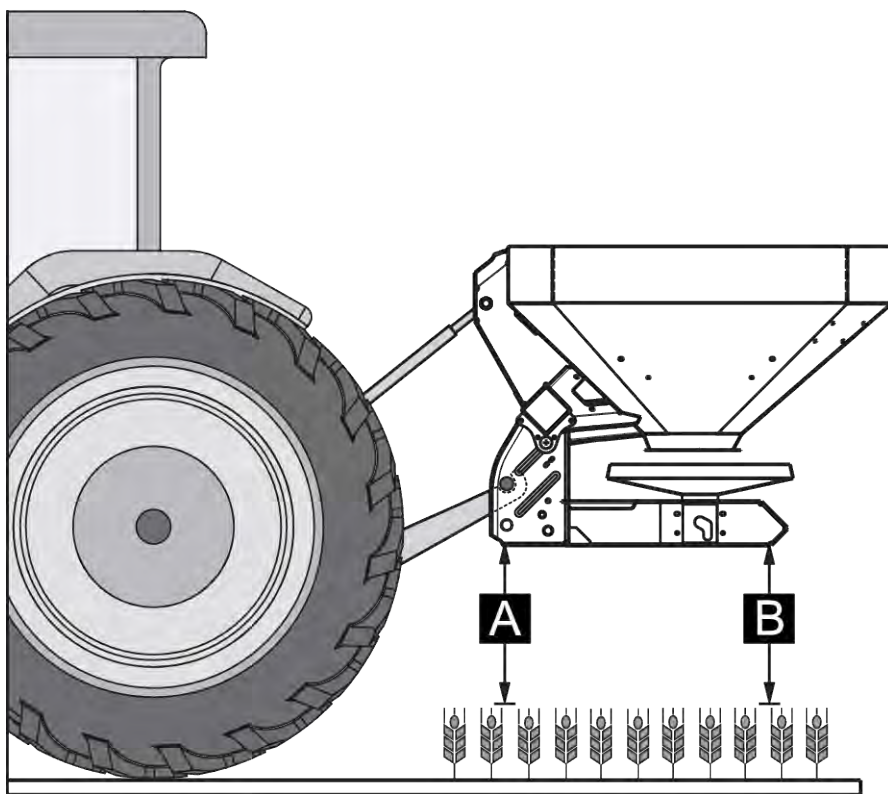
Obr. 18: Montážna poloha
