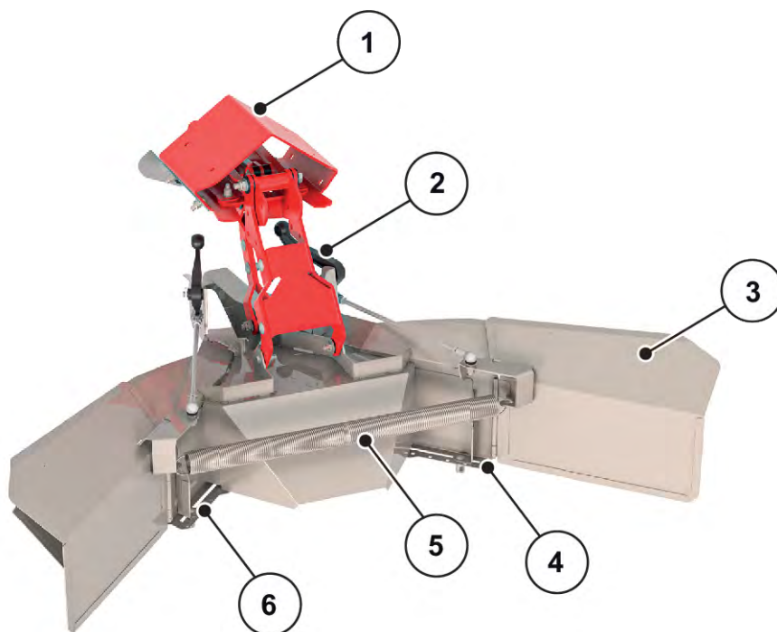
Obr. 29: Nastavenie zariadenia na hraničné rozmetávanie
