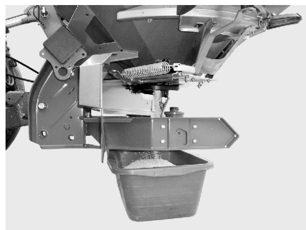
Jn. 45: Annustuskatse läbiviimine
