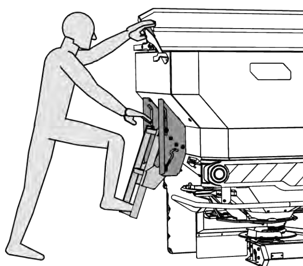
Jn. 49: Trepp koos punkrikattega
