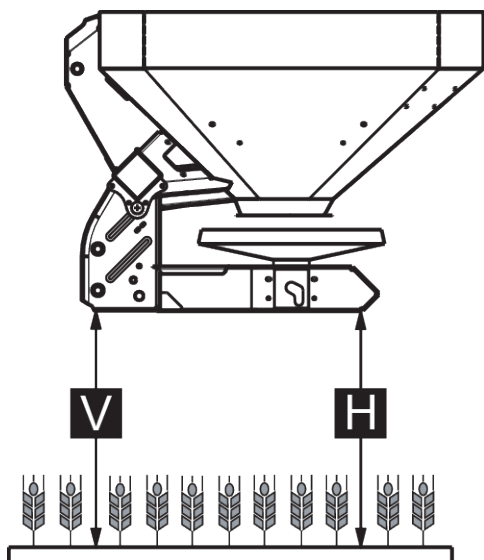
Jn. 19: Maksimaalne lubatav paigalduskõrgus tavalise ja hilise väetamise korral
