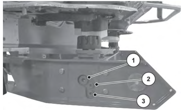
Jn. 71: Transmissiooniõli lisamis- ja väljalaskmiskohad
