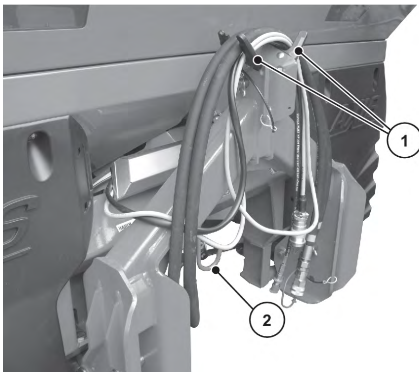
Jn. 47: Kaablite ja hüdraulikavoolikute hoidik
