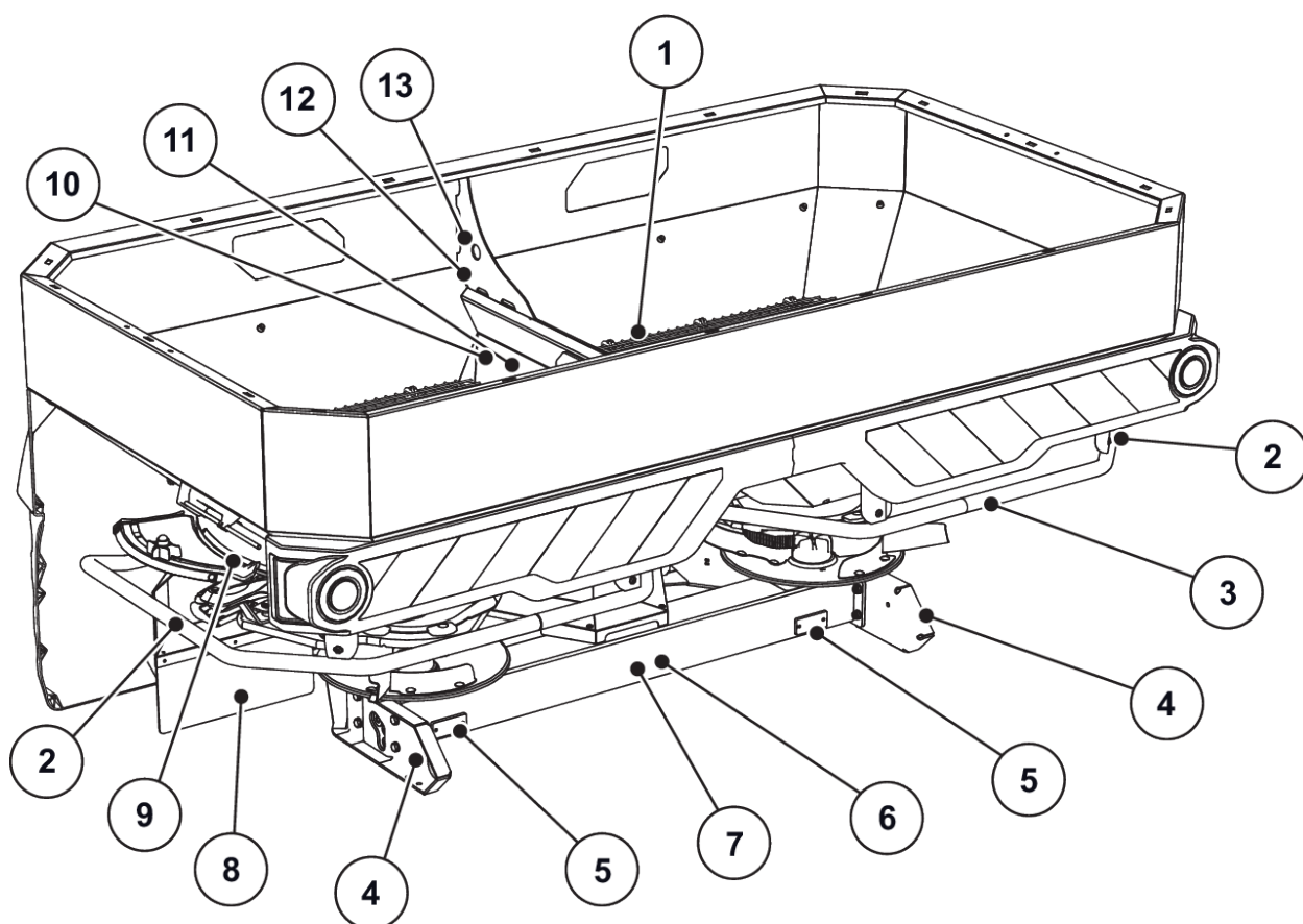
Jn. 3: Kaitseesadised, hoiatuste ja juhiste kleebsed, tagakülg
