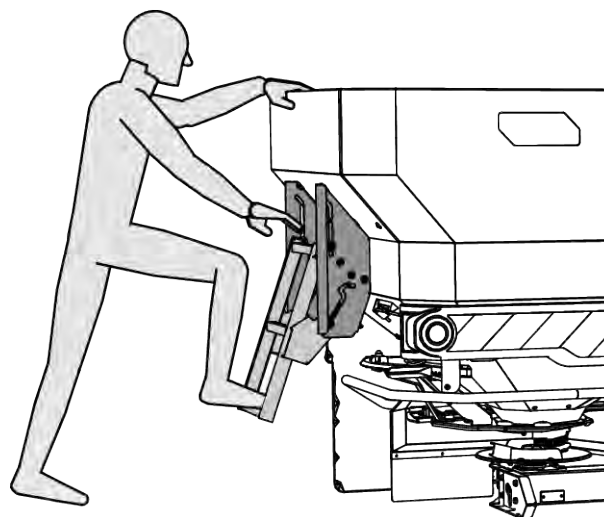
Jn. 48: Trepp ilma punkrikatteta
