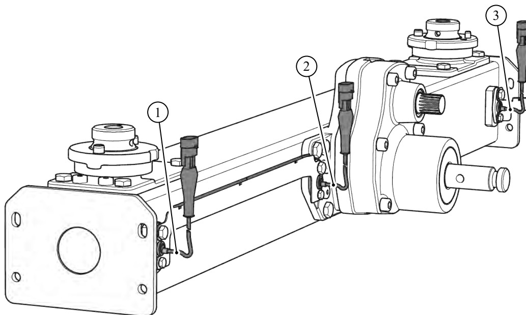
Jn. 8: Massivoolu reguleerimine kettatüüpide pöördemomendi mõõtmise abil
