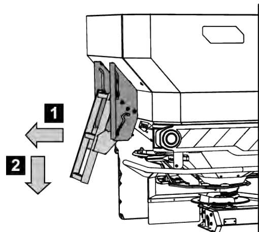
Jn. 50: Trepi lahtiklappimine
