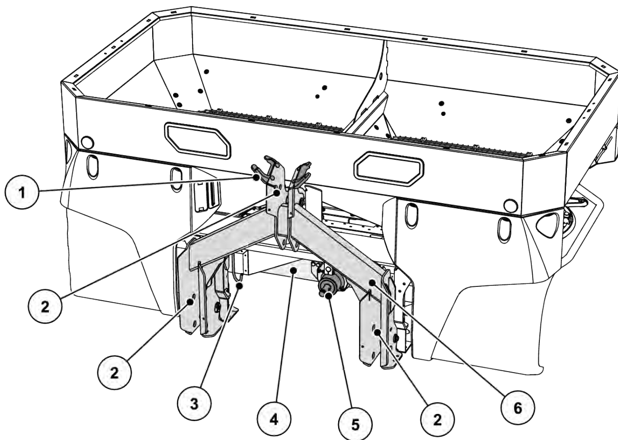
Jn. 6: Koostesõlmede ülevaade: Esikülg
