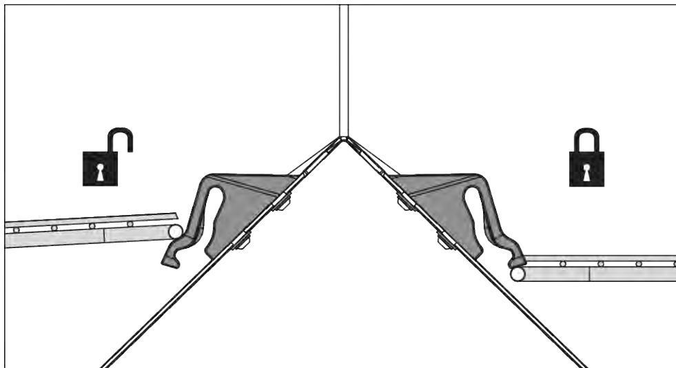
Jn. 55: Kaitsevõre lukustuse avamine/sulgumine
