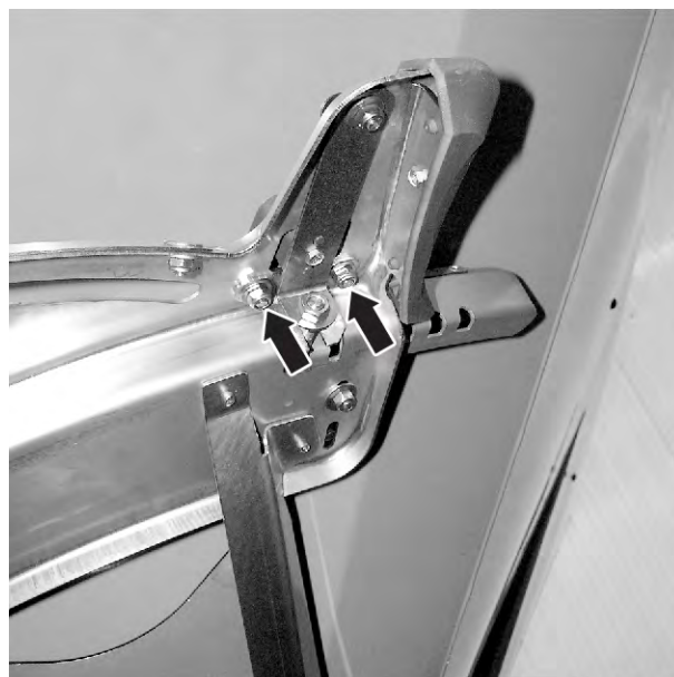
Jn. 70: Äraandmispunkti reguleerimisplaadi avamine
