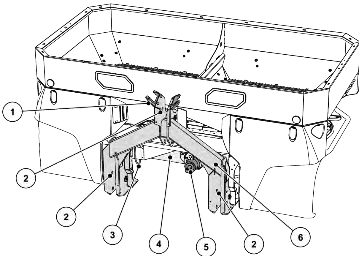
Ábr. 6: Részegységek áttekintése: első oldal
