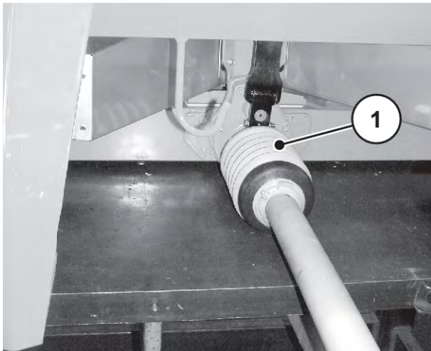
[1] Kardántengelyvédő
