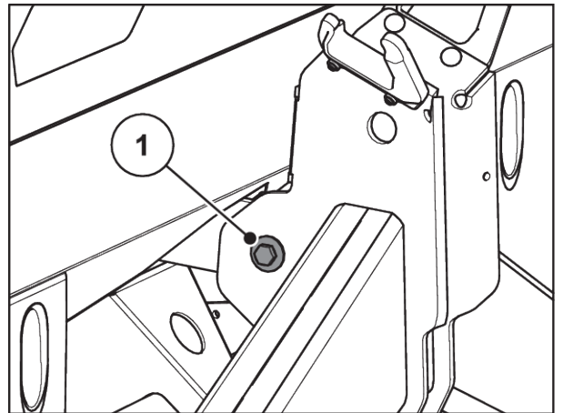
Ábr. 53: A húzórud rögzítése a mérőkereten
