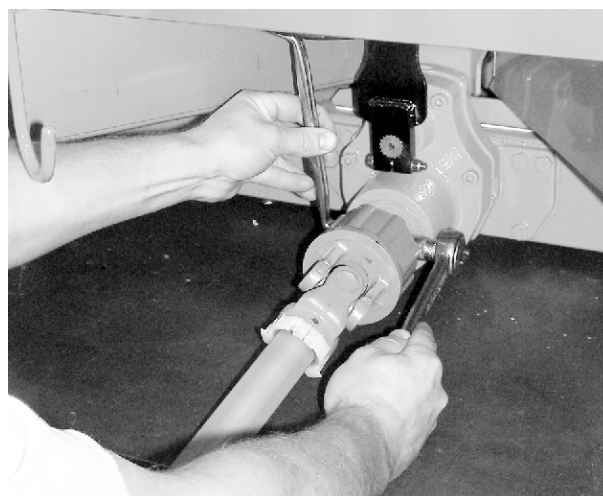
Ábr. 13: Kardántengely rögzítése
