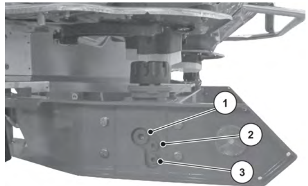
Ábr. 71: Hajtóműolaj betöltési és leeresztési helyei
