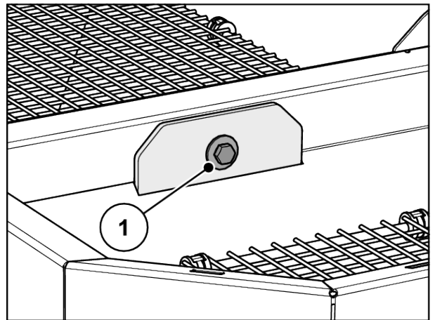
Ábr. 54: A húzórud rögzítése a tartályban
