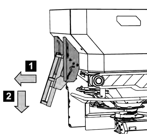
Ábr. 50: Fellépő kihajtása
