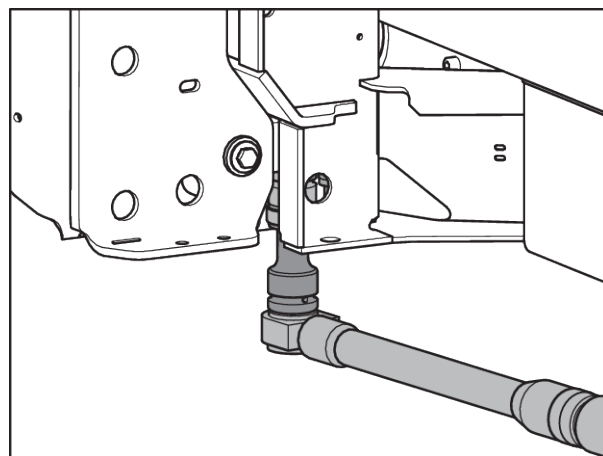
Sl. 52: Pričvršćivanje ćelije za vaganje (u smeru vožnje levo)
