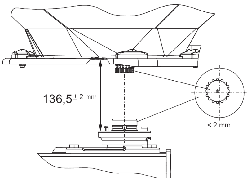
Sl. 59: Provera položaja glavčine diska za rasipanje
