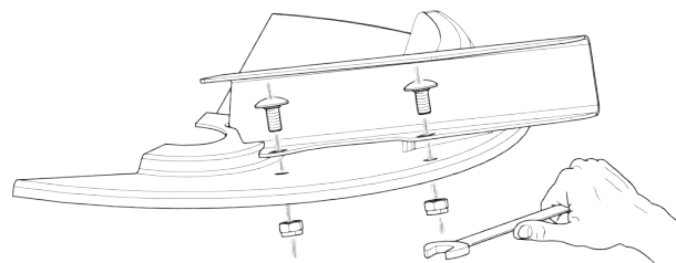
Sl. 63: Otpuštanje zavrtnja na lopatici za rasipanje
