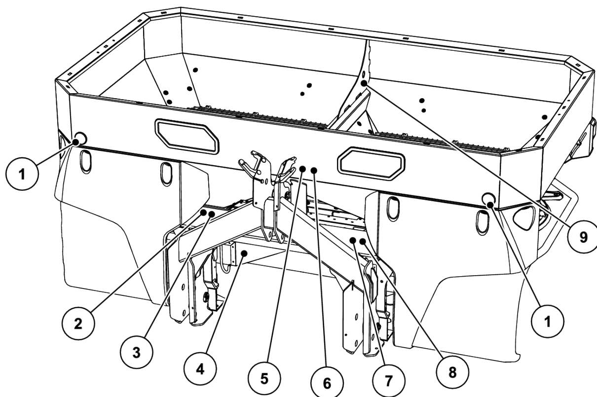
Sl. 4: Zaštitna oprema, nalepnice sa upozorenjima i napomenama na prednjoj strani
