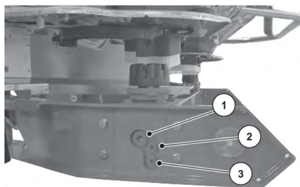
Sl. 71: Mesta za punjenje i ispuštanje ulja za prenosnike
