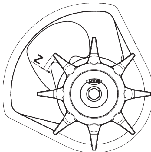
Sl. 61: Opseg habanja glave mešalice
