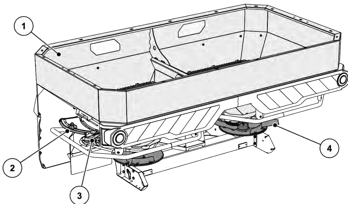
Sl. 7: Pregled sklopova: Zadnja strana
