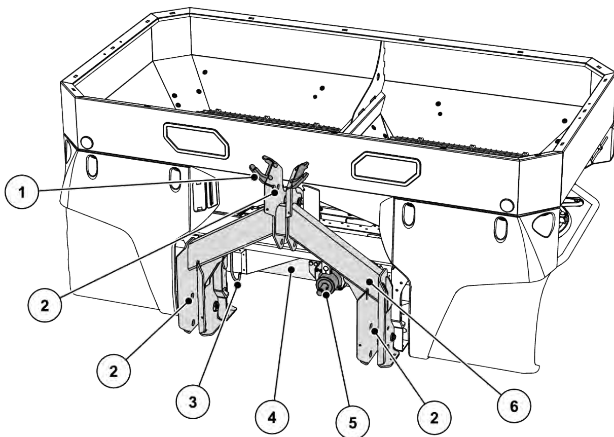
Рис. 6: Обзор конструктивных узлов: Передняя сторона
