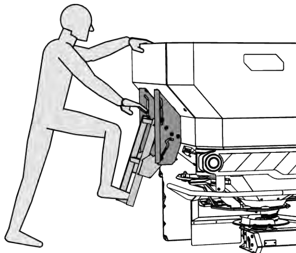
Рис. 48: Подъем без брезента на бункере
