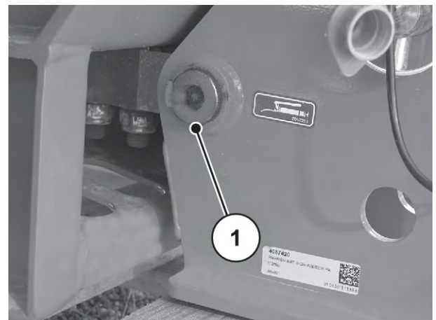
Fig. 73: Smørepunkt vektspreader
