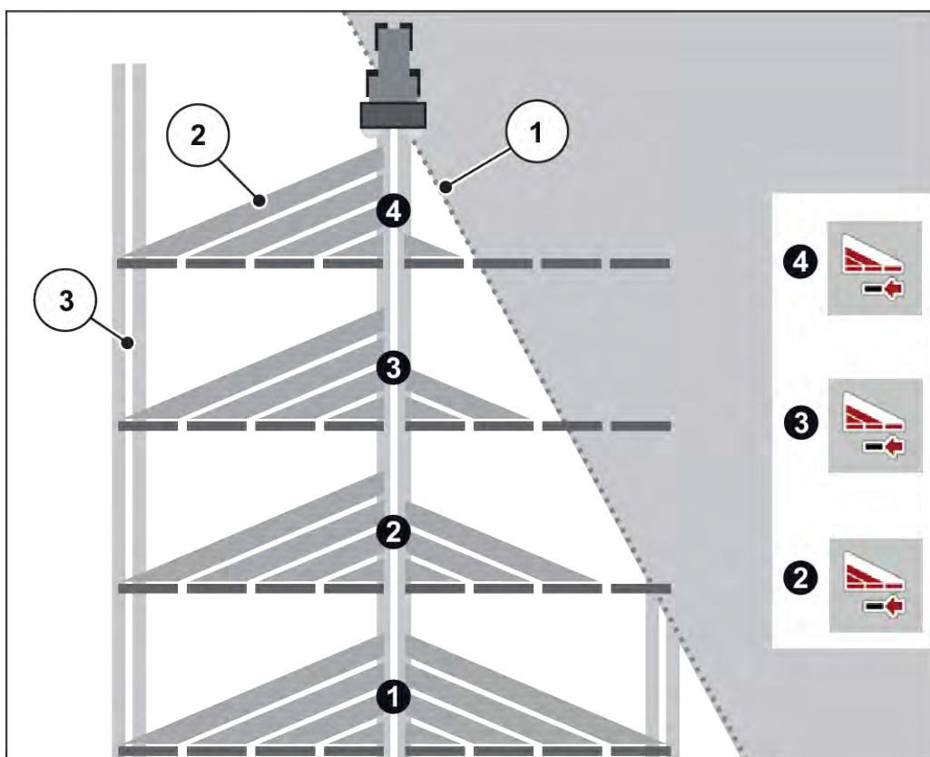
Fig. 39: Eksempel delbreddekobling
