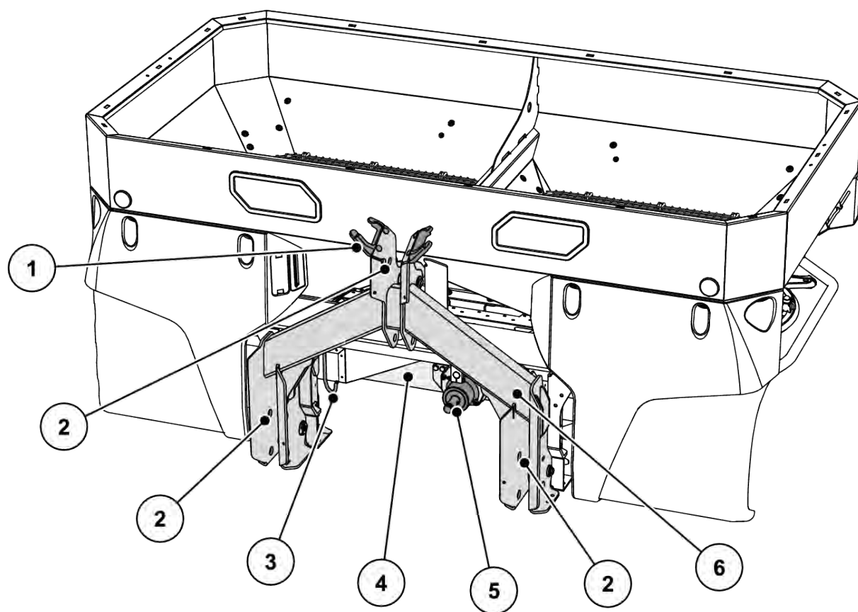
Fig. 6: Komponentoversikt: Forside
