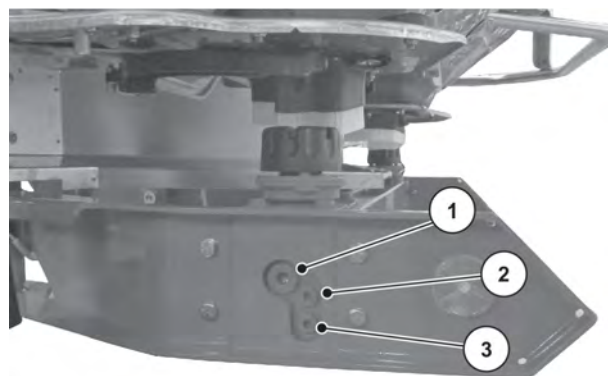
Fig. 71: Fylle- og tappesteder for girolje
