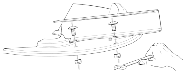
Fig. 63: Løsne skruene til spredevingen
