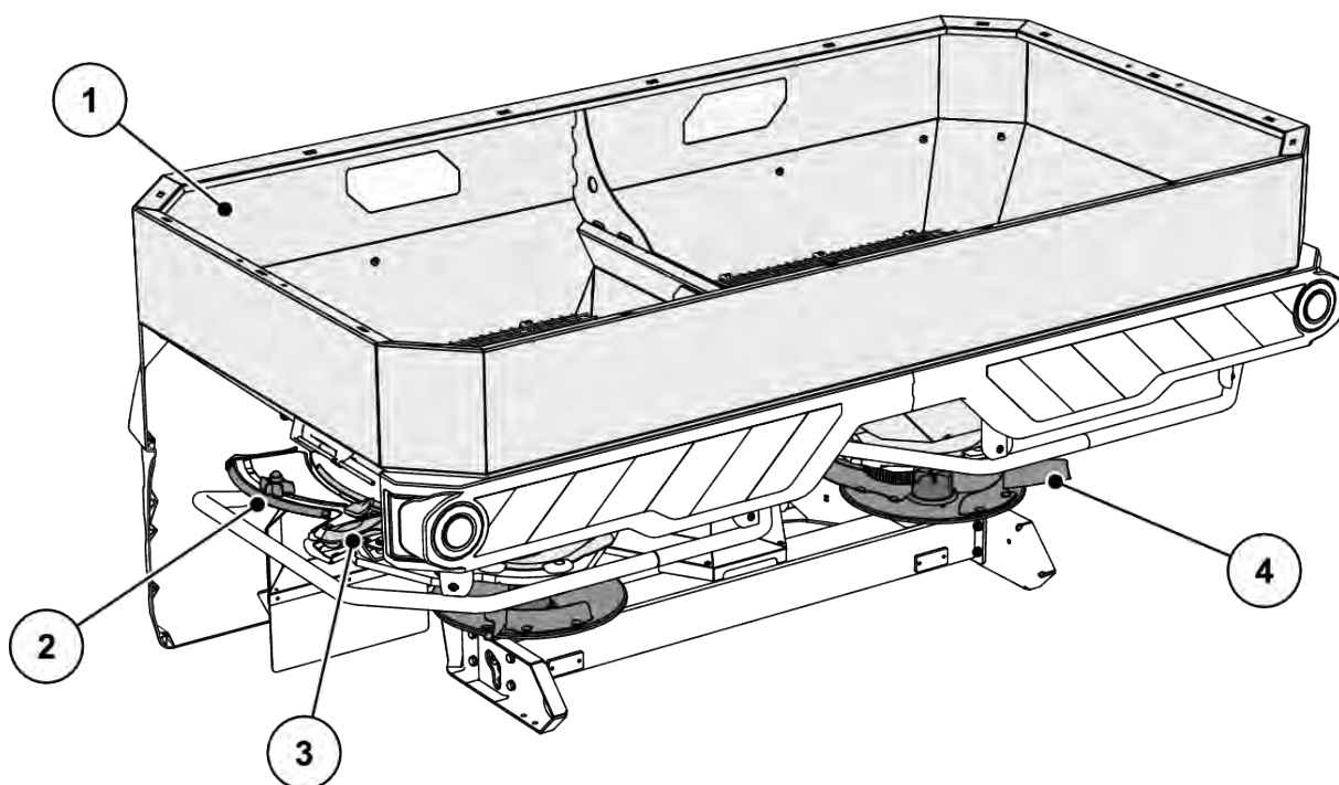
Fig. 7: Komponentoversikt: Bakside
