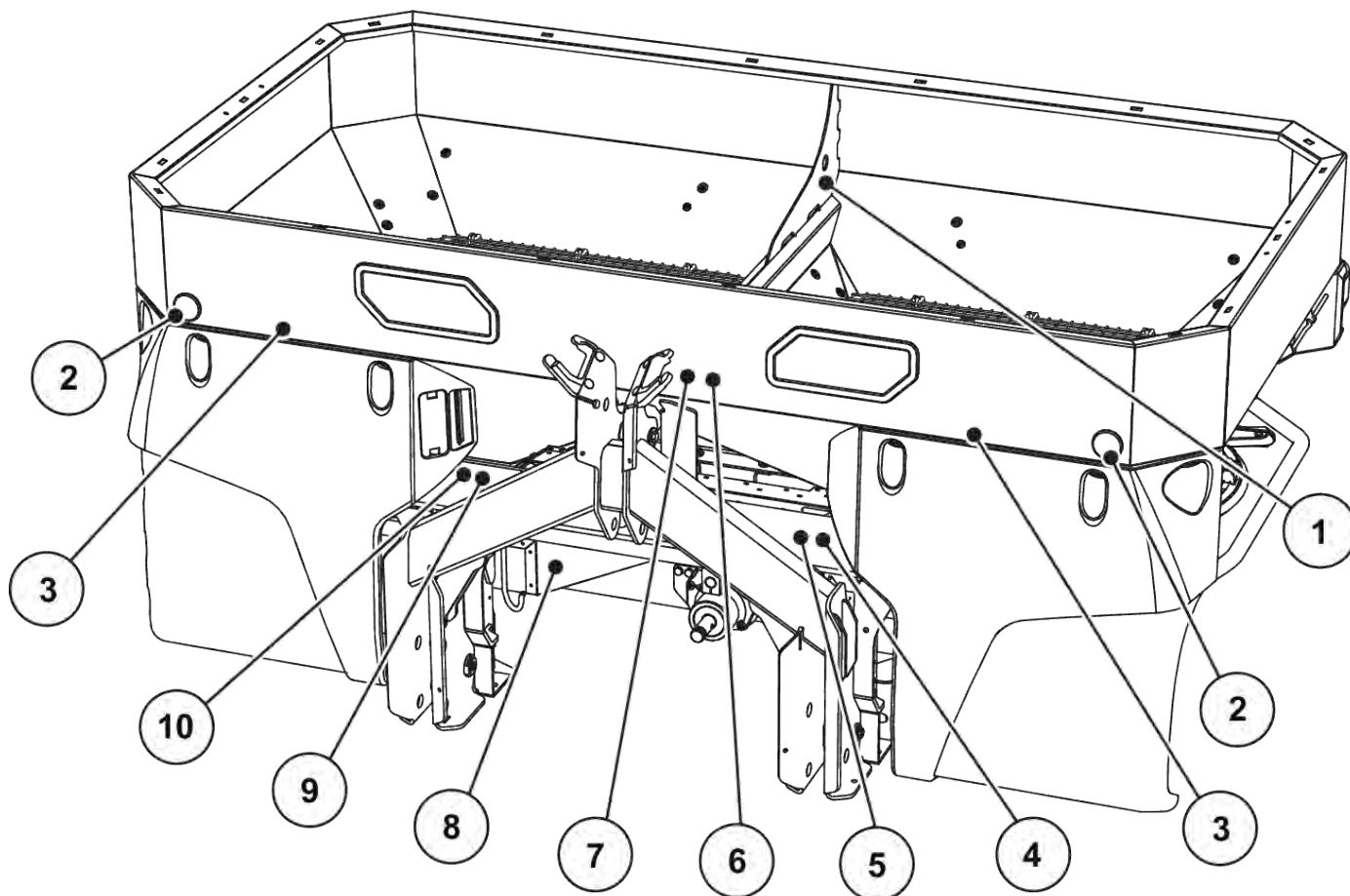
Fig. 2: Beskyttelsesinnretninger, klistremerke Advarsler og instruksjonsanvisninger, framside
