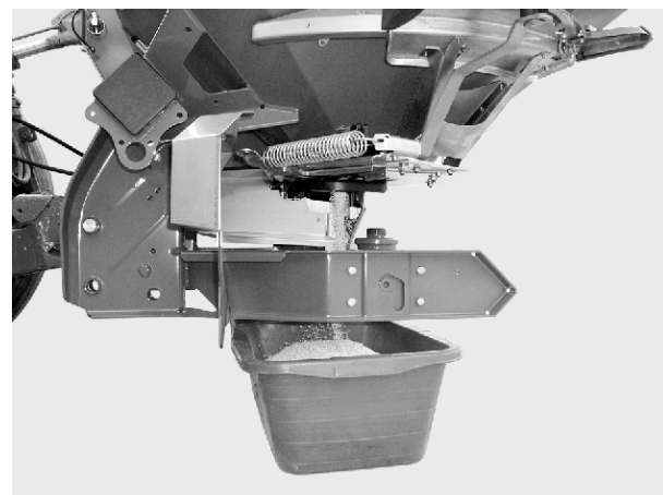
Fig. 45: Utføre kalibreringstest
