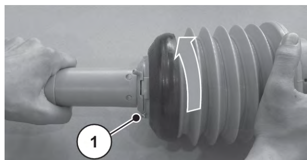
Fig. 11: Løsne kardangakselbeskyttelsen
