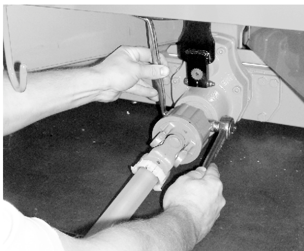
Fig. 13: Fest kardangakselen
