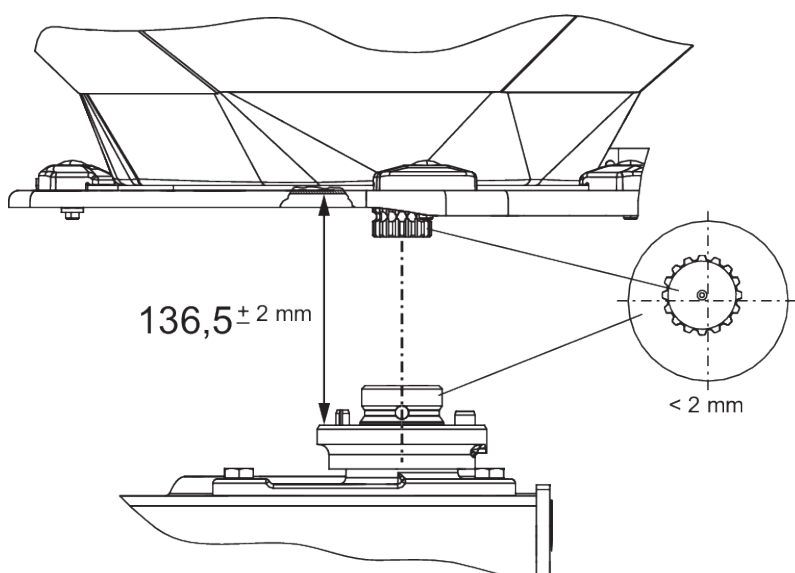
Sl. 59: Provjera glavčine diska za rasipanje
