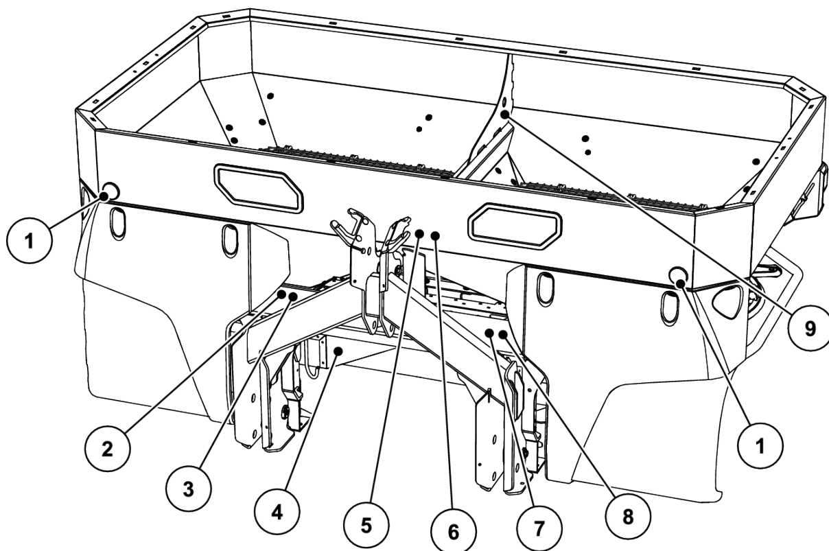
Sl. 4: Zaštitna oprema, naljepnice s upozorenjima i napomenama, prednja strana
