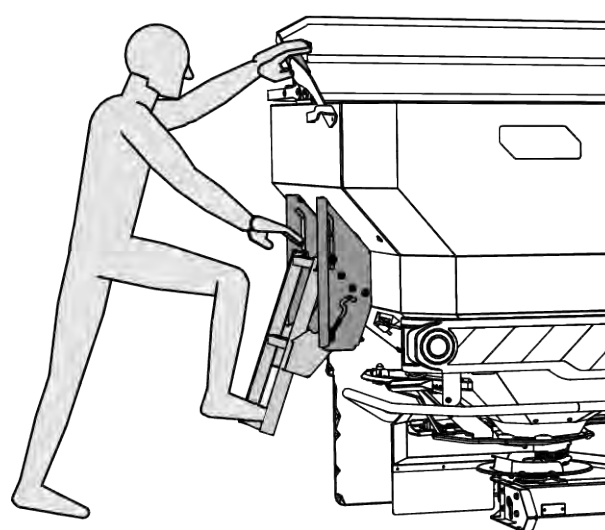
Sl. 49: Ljestve s pokrovnom ceradom spremnika
