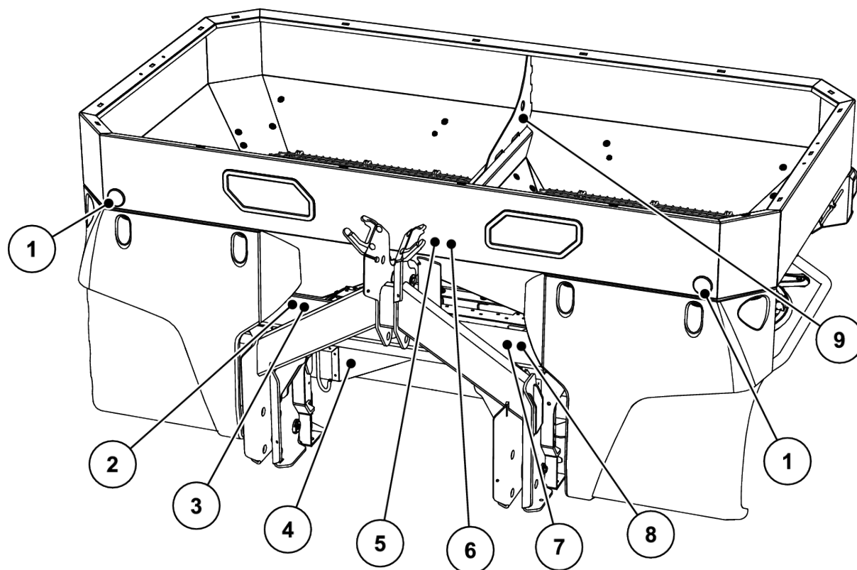
Fig. 4: Beskyttelsesordninger samt advarsels- og instruktionsmærkater på forsiden
