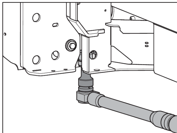
Fig. 52: Fastgørelse af vejecellen (til venstre set i kørselsretningen)
