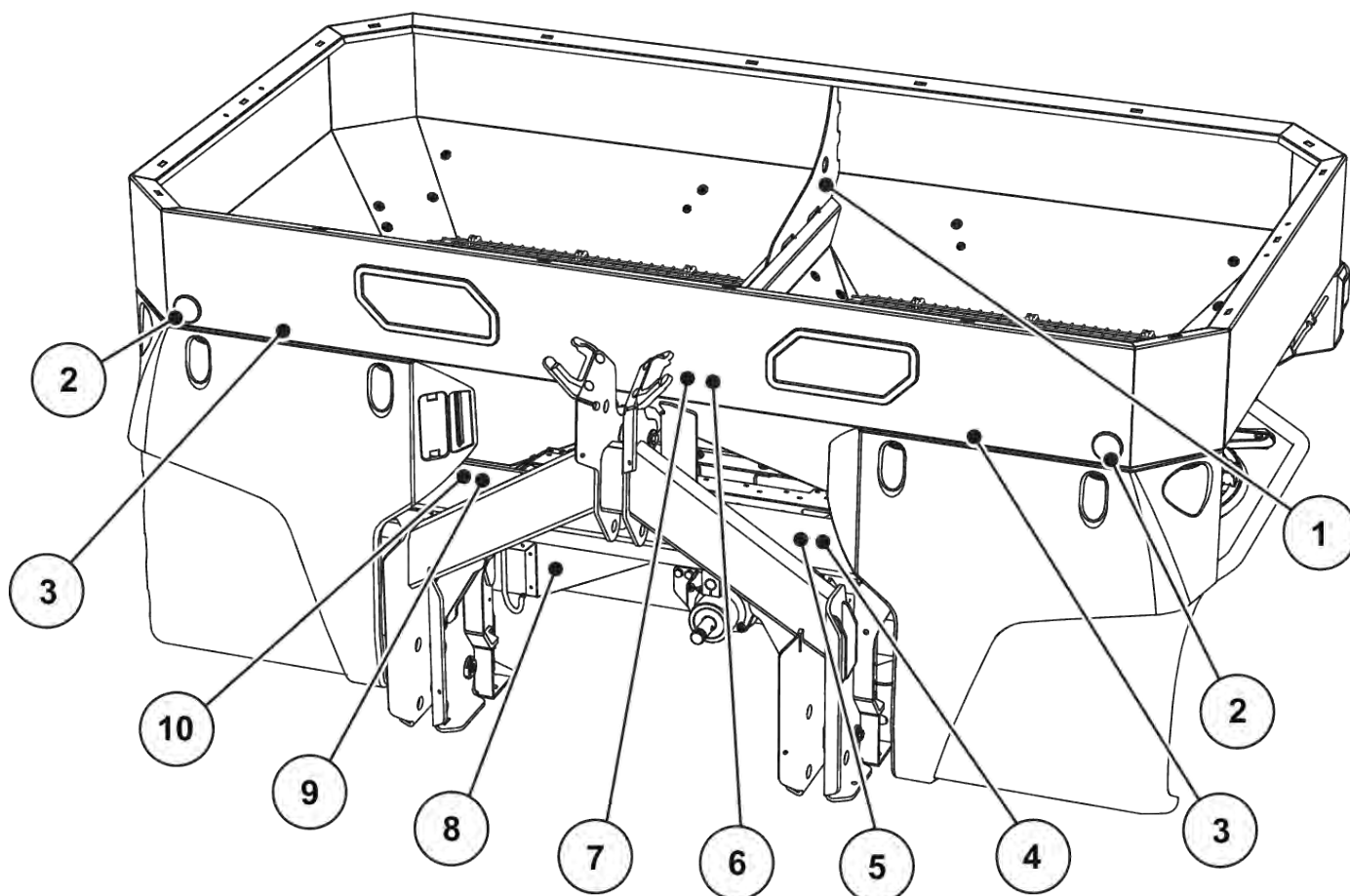
Fig. 2: Beskyttelsesanordninger samt advarsels- og instruktionsmærkater på forsiden
