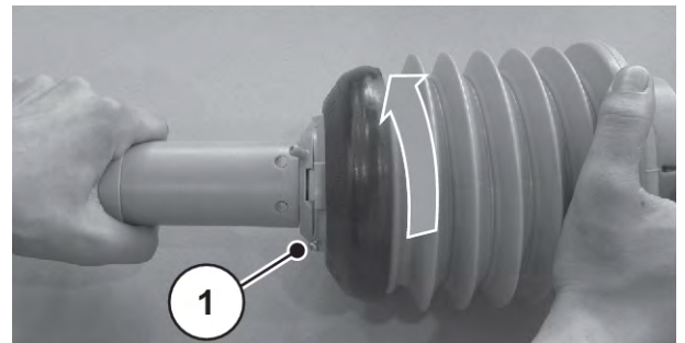
Ilust. 11: Soltar la protección de eje articulado
