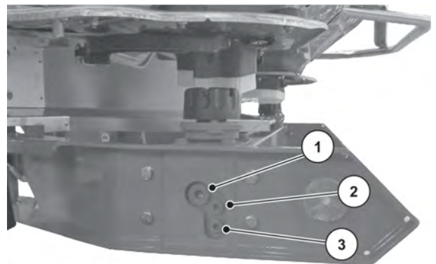
Ilust. 67: Puntos de llenado y de vaciado del aceite de engranaje
