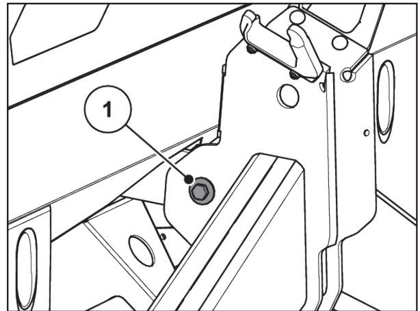
Ilust. 49: Fijación de la barra de tracción en el bastidor de pesaje
