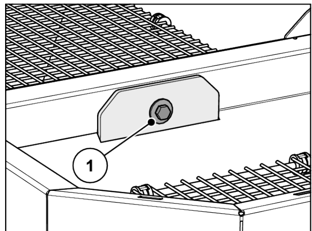
Ilust. 50: Fijación de la barra de tracción en el depósito
