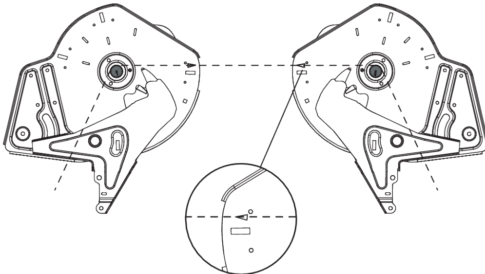
Ilust. 65: Comprobar el ajuste del punto de aplicación
