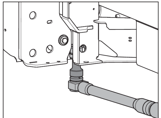
Ilust. 48: Fijación de la célula de pesaje (en sentido de la marcha a la izquierda)
