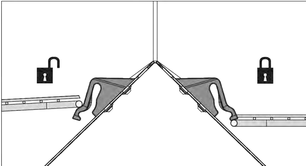
Ilust. 51: Cierre de la rejilla de protección abierto/cerrado
