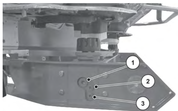
Ilust. 71: Puntos de llenado y de vaciado del aceite de engranaje
