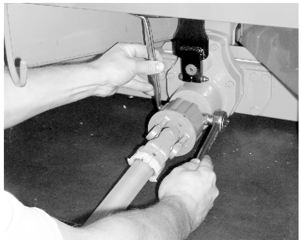
Ilust. 13: Fijar el eje articulado
