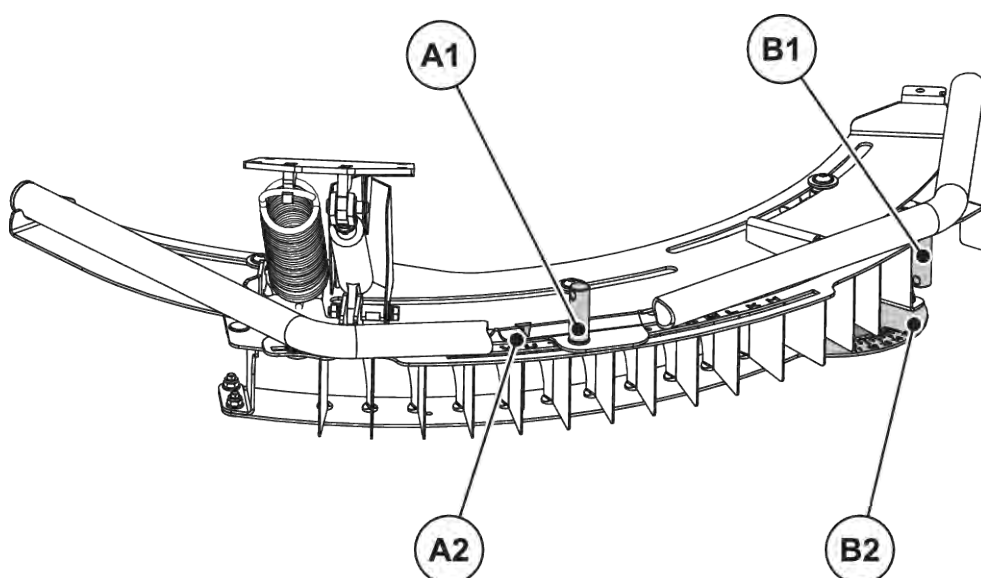
Ilust. 30: Ajustar el dispositivo TELIMAT
