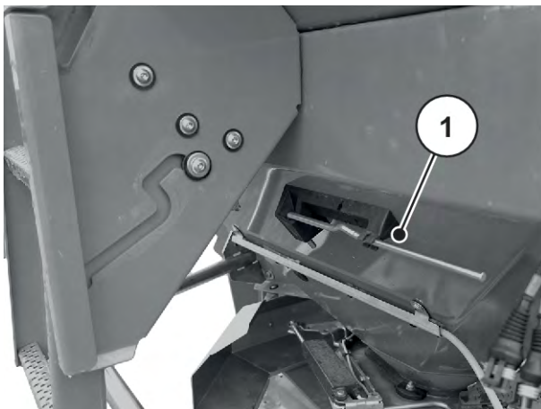
Ilust. 32: Posición de la palanca de ajuste del EJE xx.2
