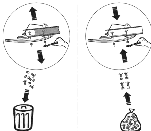
Ilust. 64: Utilizar tuercas nuevas de autobloqueo
