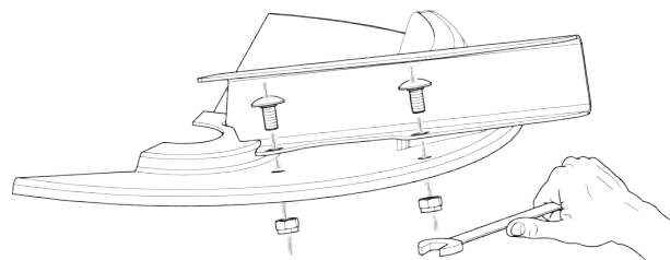
Ilust. 63: Afloje los tornillos de las aletas de dispersión
