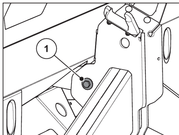
Ilust. 53: Fijación de la barra de tracción en el bastidor de pesaje
