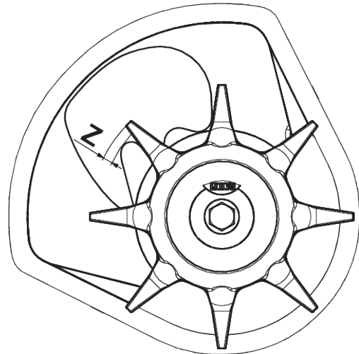
Ilust. 61: Área de desgaste del cabezal agitador
