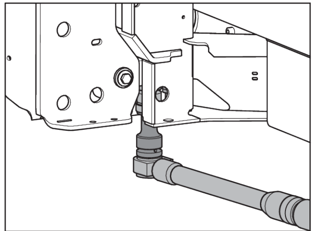
Ilust. 52: Fijación de la célula de pesaje (en sentido de la marcha a la izquierda)
