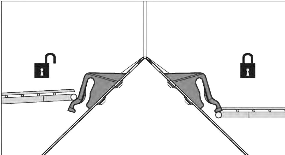
Ilust. 55: Cierre de la rejilla de protección abierto/cerrado
