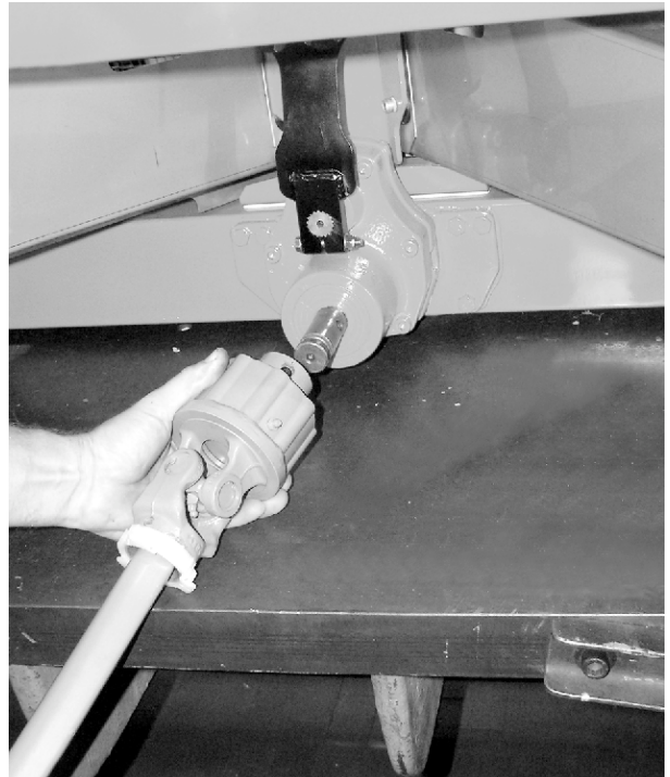
Ilust. 12: Inserción del eje articulado en el muñón de engranaje
