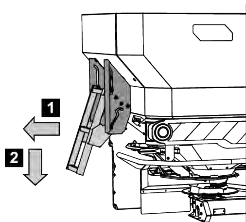
Afb. 50: Opstapje uitklappen
