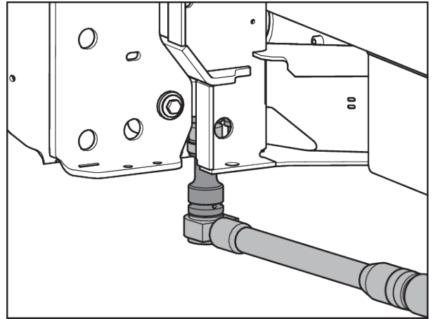
Afb. 52: Bevestiging van de weegcel (in rijrichting links)
