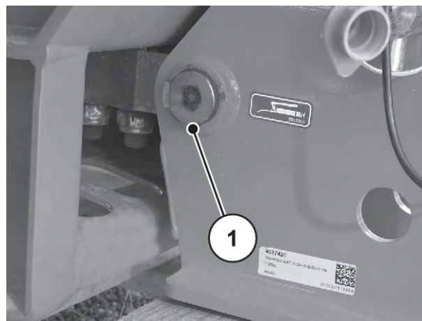
Afb. 73: Smeerplaats weegstrooier
