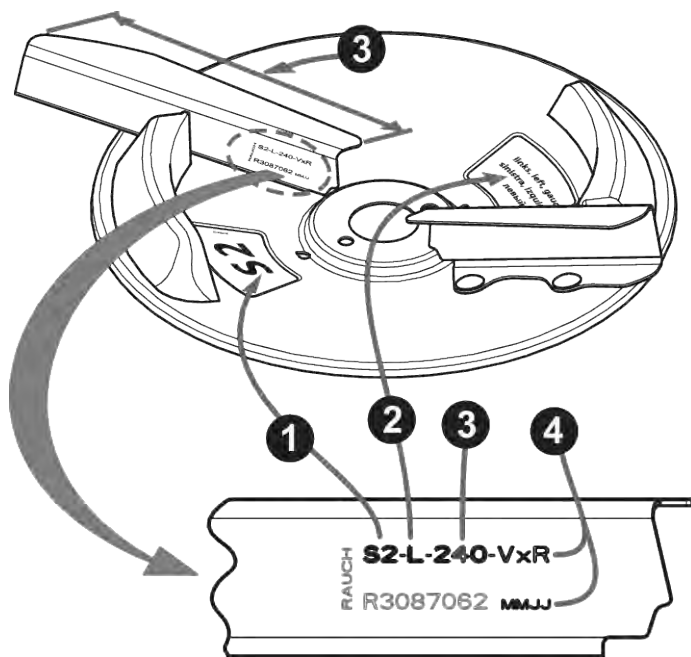
Afb. 62: Opschrift strooischijf
