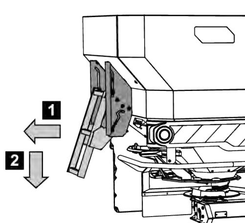
Fig. 50: Deplierea scării
