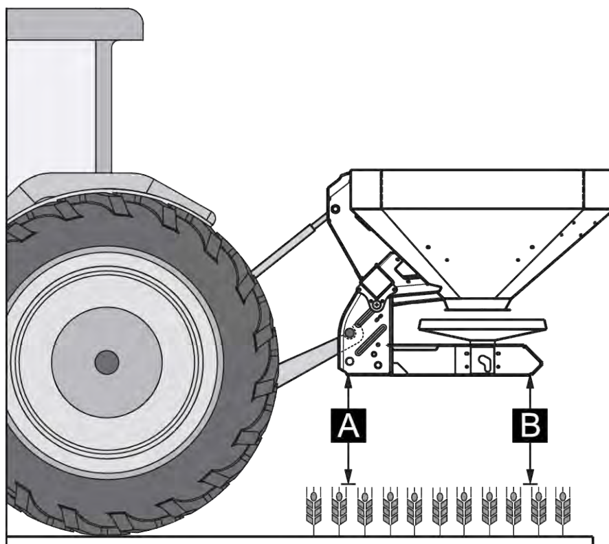
Fig. 20: Poziția și înălțimea de atașare în cazul fertilizării normale
