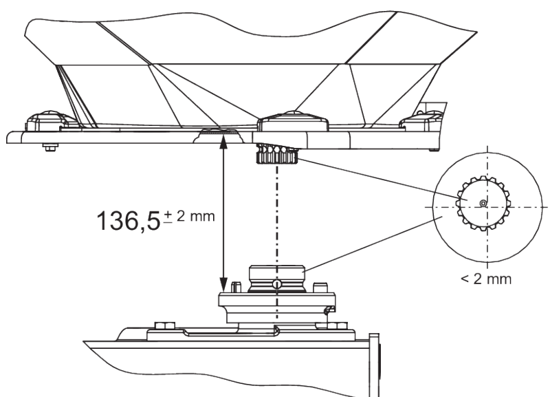
Fig. 59: Verificarea poziției butucului discului aruncător
