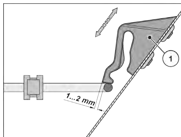
Fig. 57: Cote pentru verificarea funcționării dispozitivului de blocare a grilajului de protecție
