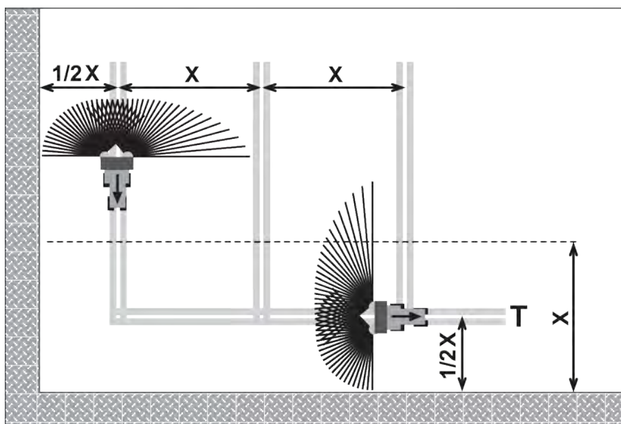
Fig. 37: Împrăștiere la limită
