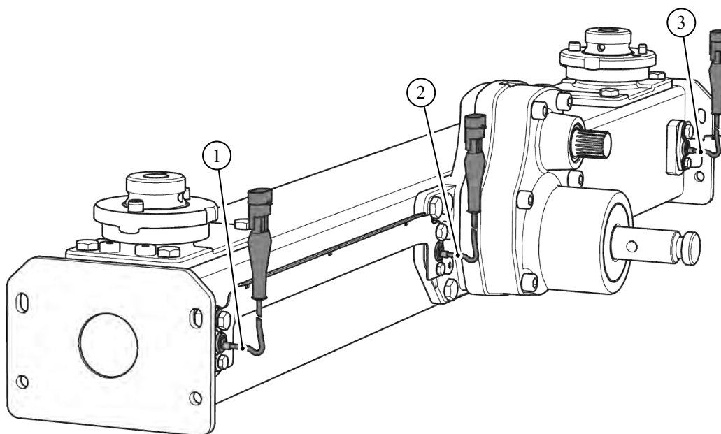
Fig. 8: Reglarea debitului masic prin măsurarea momentului de rotație al discurilor aruncătoare
