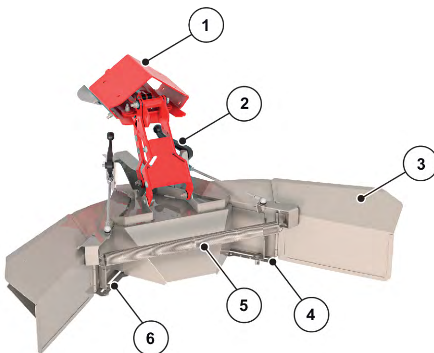
Fig. 29: Reglarea dispozitivului de împrăștiere la limită
