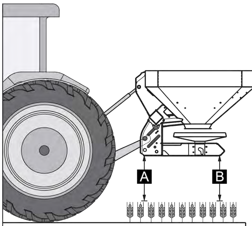
Fig. 18: Poziția de montare
