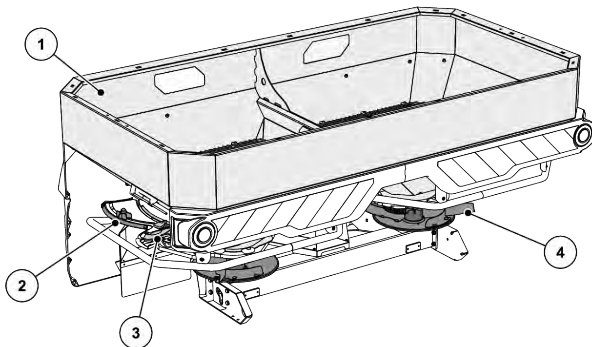
Fig. 7: Prezentare generală a subansamblelor: Partea din spate
