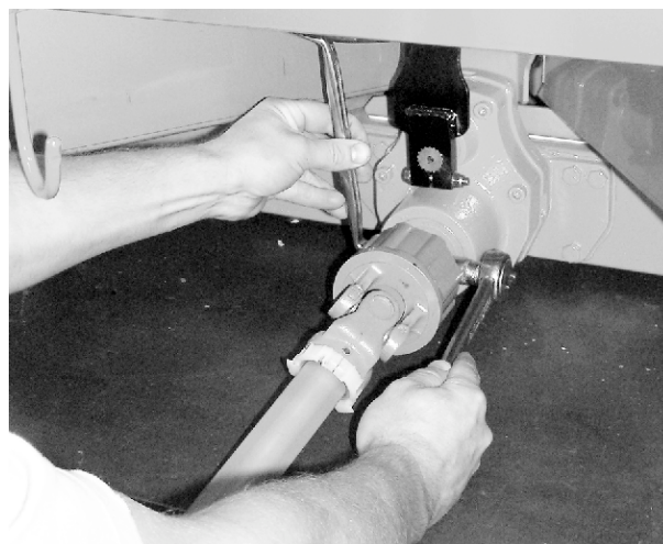
Fig. 13: Fixarea arborelui cardanic
