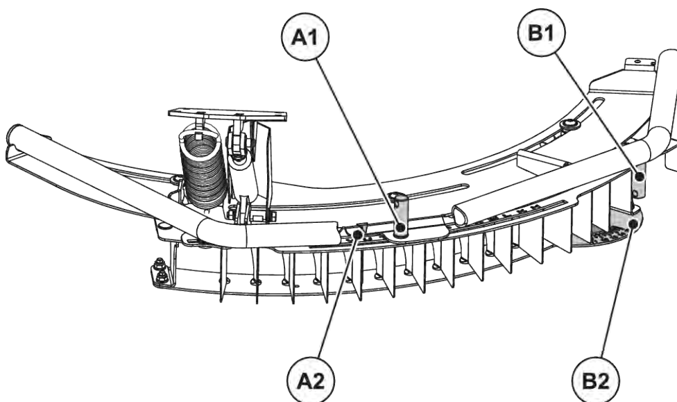
Fig. 30: Reglarea dispozitivului TELIMAT
