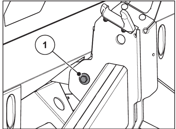
Mynd 48: Festing álagsstangar á vigtunargrind
