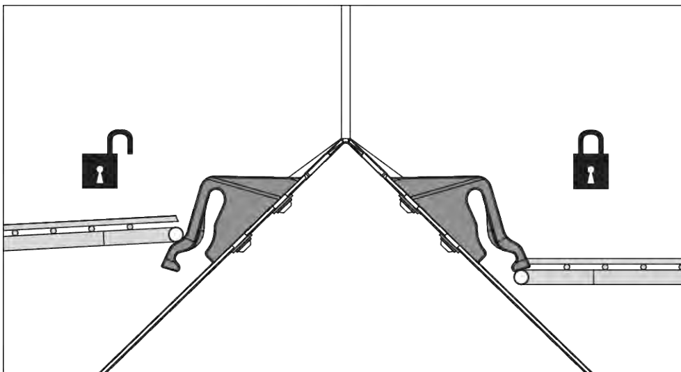
Mynd 50: Hlífðargrind ólæst/í lás
