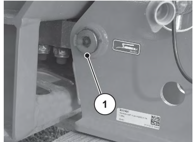
Mynd 68: Smurstaður dreifara með álagsnema [1] Smurstaður
