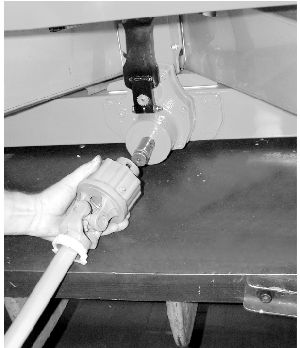
Mynd 12: Drifskafinu stungið á drifásinn
