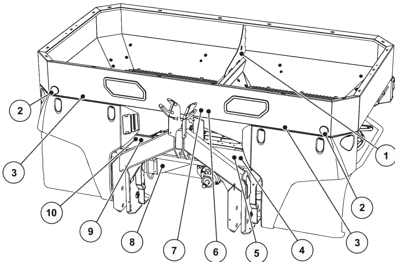
Mynd 2: Hlíðarbúnaður, limmiðar með viðvörunum og leiðbeiningum á framhlið
