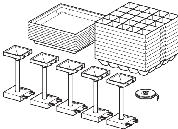
Mynd 10: sérbúnaður PPS5
