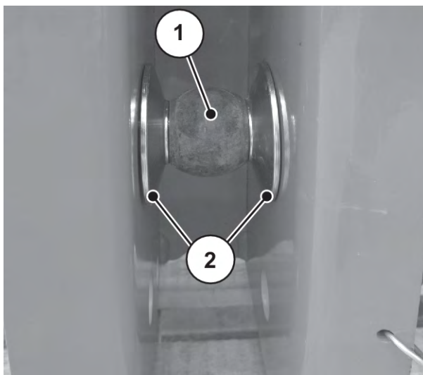
Mynd 17: Staðsetning millileggja þegar vélin er sett á
