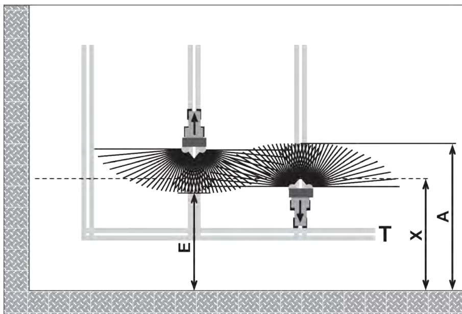
Mynd 38: Venjuleg dreifing
