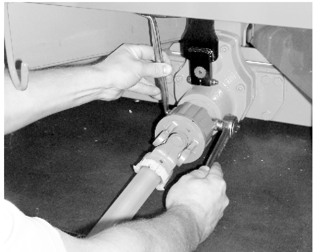
Mynd 13: Drifskafið fest
