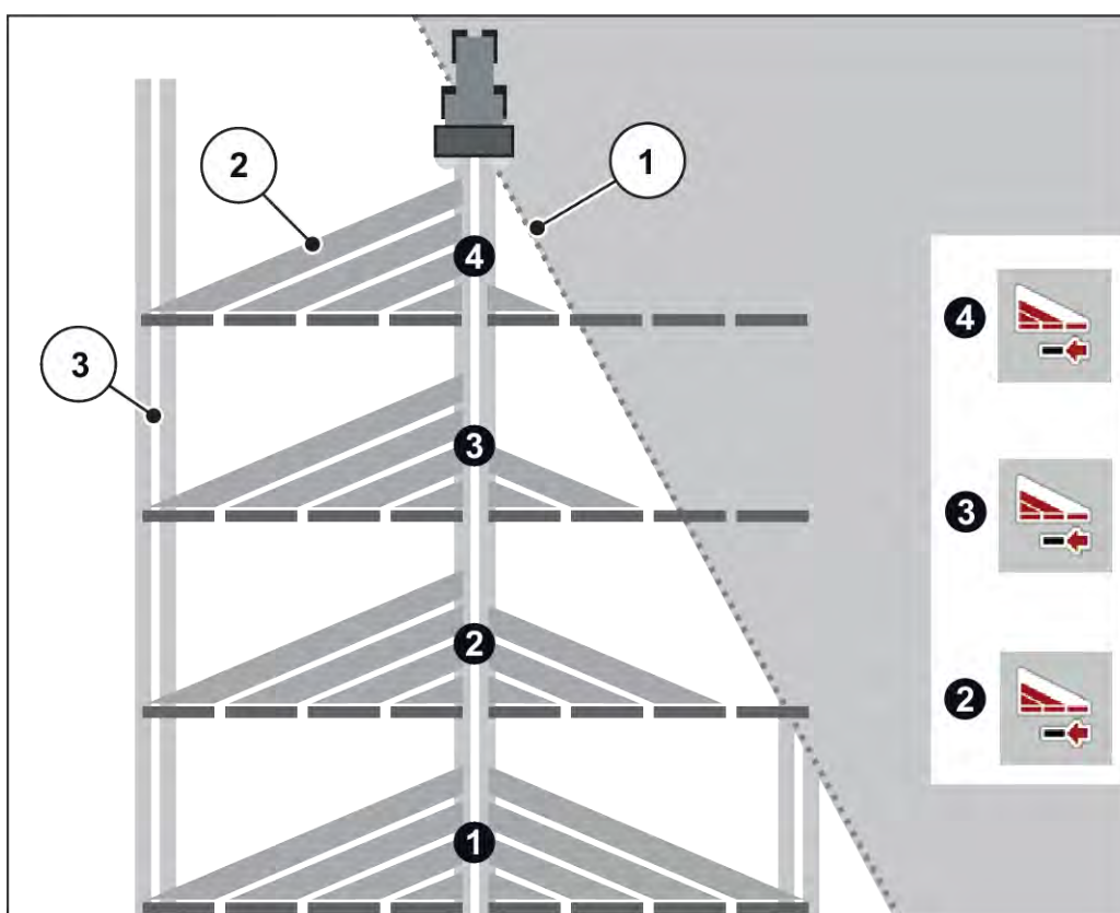
Mynd 39: Dæmi um kaflastýringu
