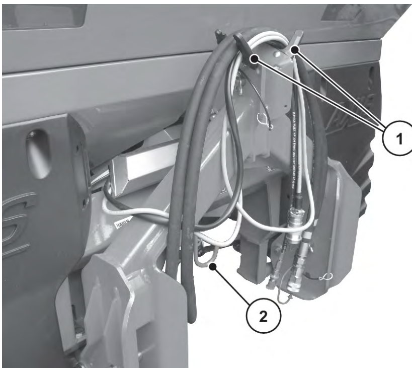
Mynd 47: Festing fyrir snúrur og vökvaslöngur
