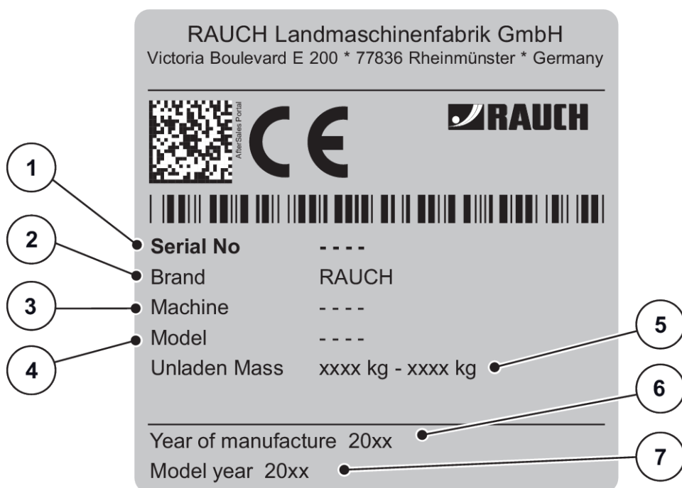
Mynd 5: Upplýsingaplata framleiðanda
