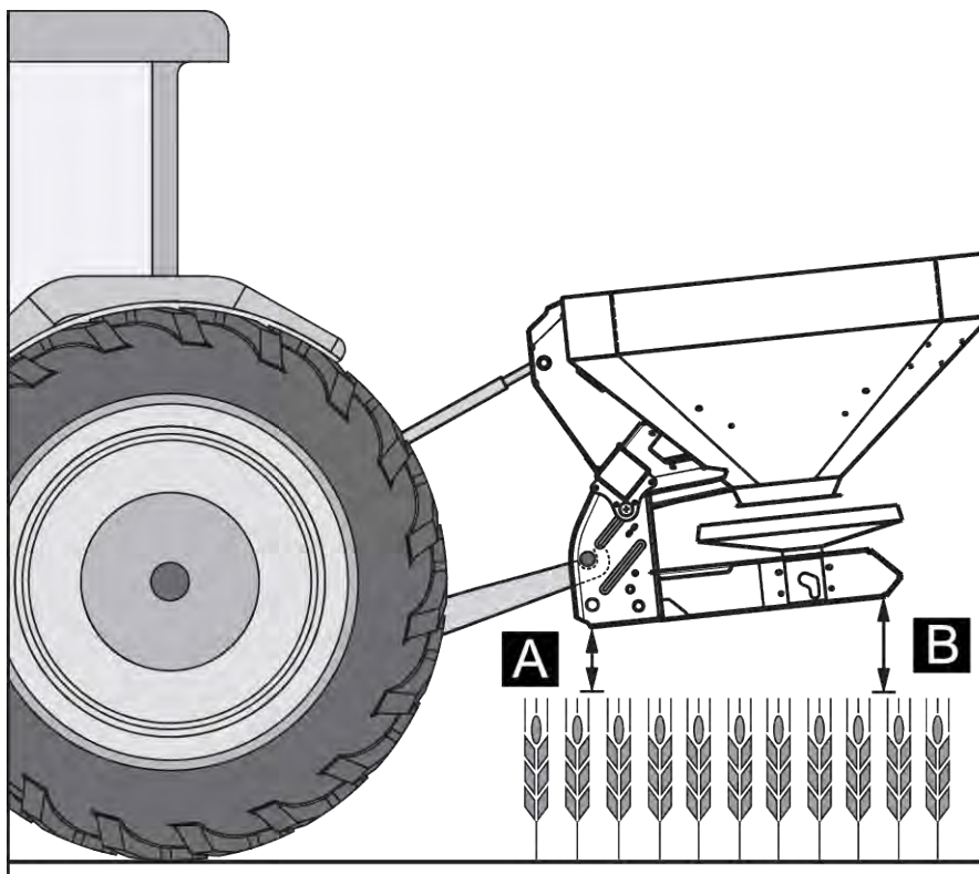
Mynd 21: Uppsetningarstaða og -hæð við síðbúna áburðargjöf
