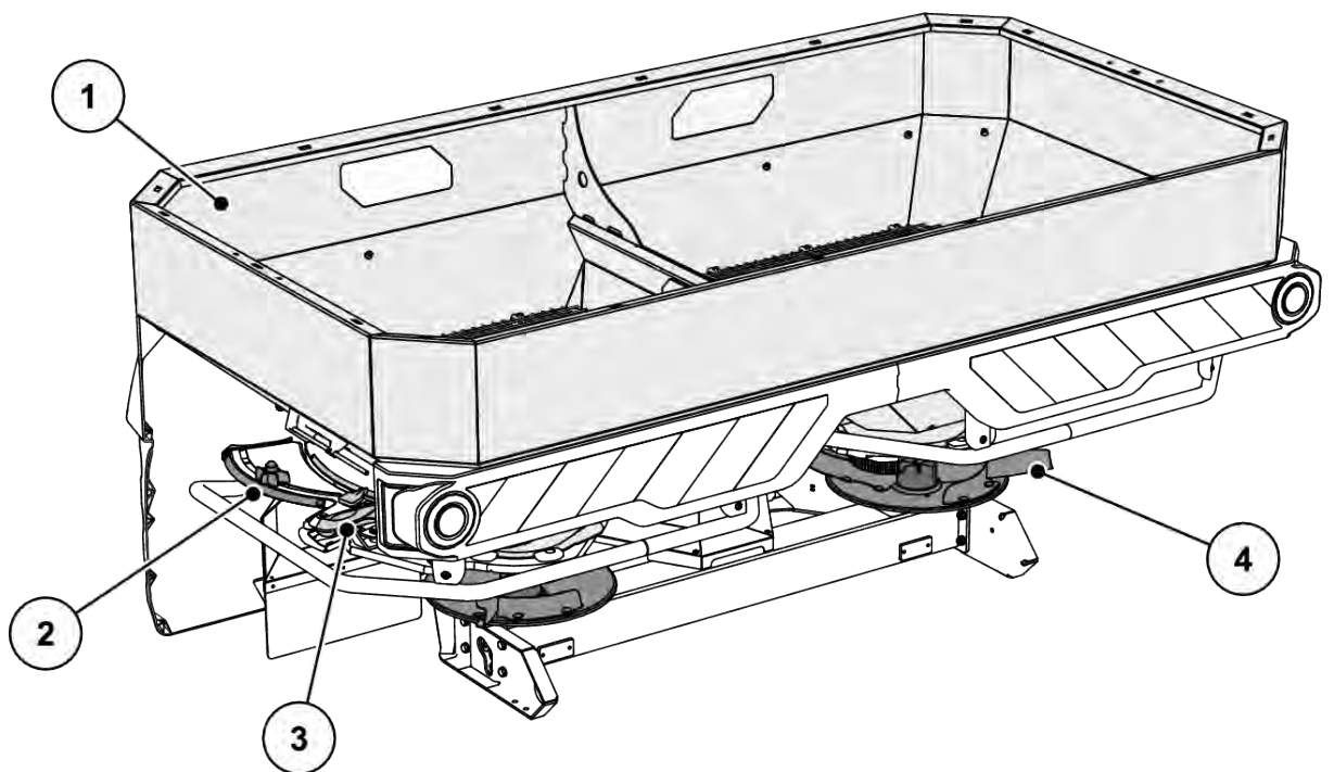
Mynd 7: Yfirlit yfir vélarhluta: Bakhlið
