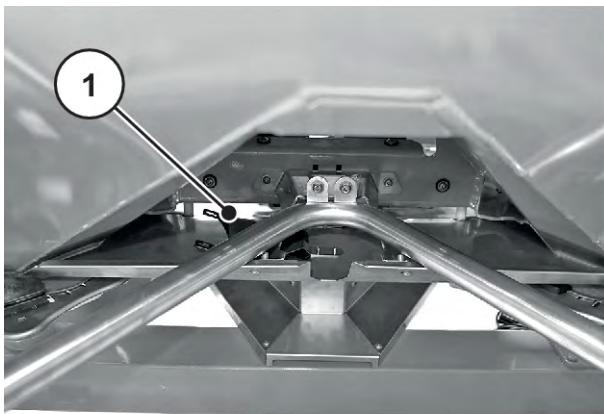
Mynd 42: Renna fyrir dreifingarprófun
