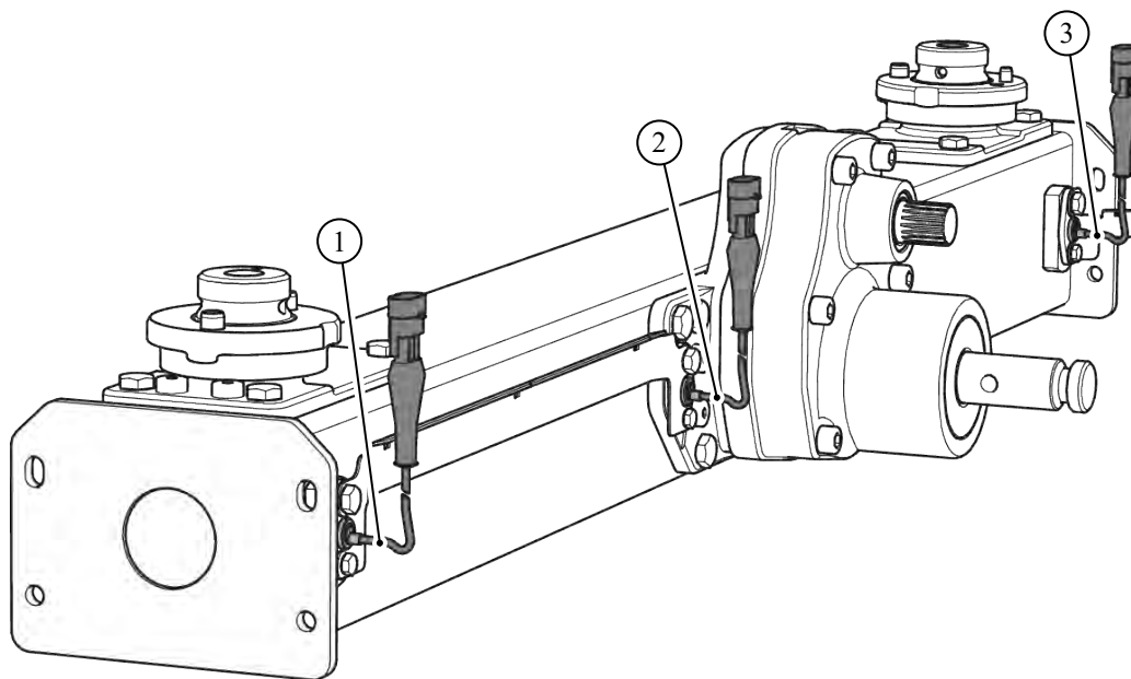
Mynd 8: Massaflæðisstýring með því að mæla tog dreifiskífanna
