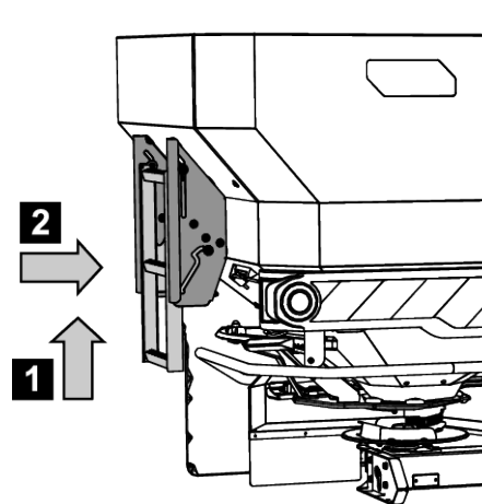
Mynd 51: Trappa í innfældri stöðu
