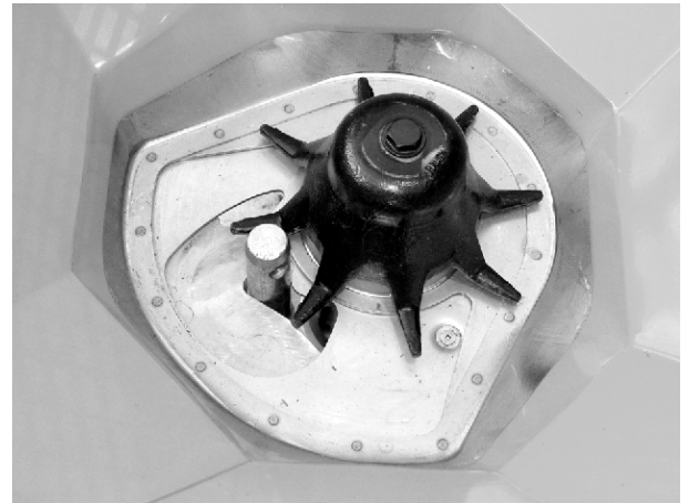
Σχ. 61: Μπουλόνι κάτω συνδέσμου μέσα στο δοσομετρικό άνοιγμα
