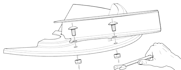
Σχ. 63: Χαλάρωση βιδών των πτερυγίων διασκορπισμού
