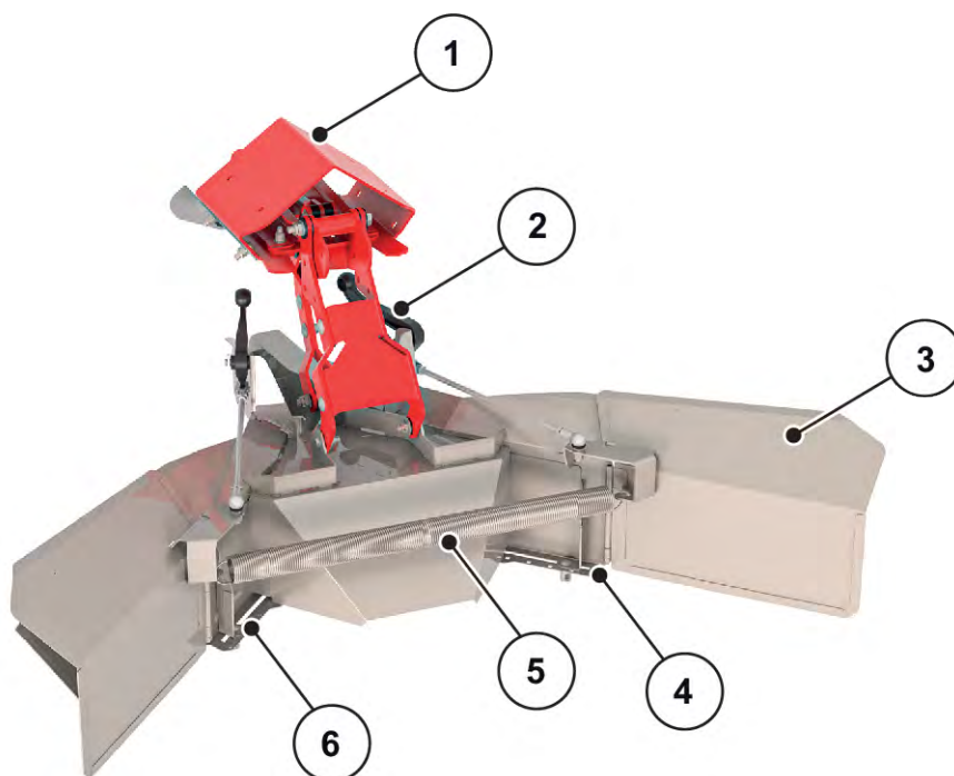
Σχ. 29: Ρύθμιση της διάταξης διασκορπισμού ορίων
