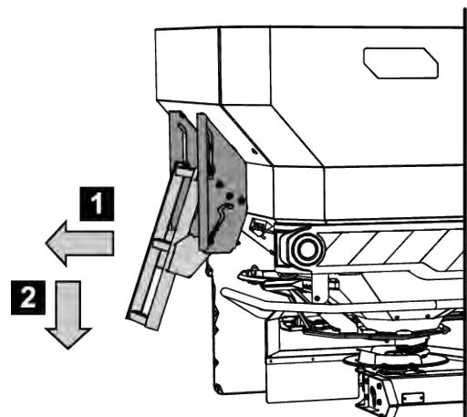
Σχ. 50: Ξεδίπλωμα βοηθήματος πρόσβασης
