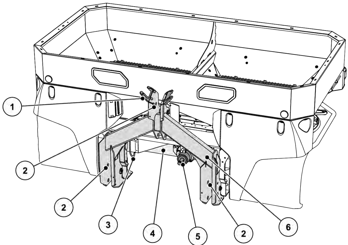
Σχ. 6: Επισκόπηση κατασκευαστικών ομάδων: Μπροστινή πλευρά
