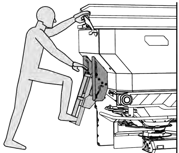
Σχ. 49: Πρόσβαση με κάλυμμα χοάνης.
