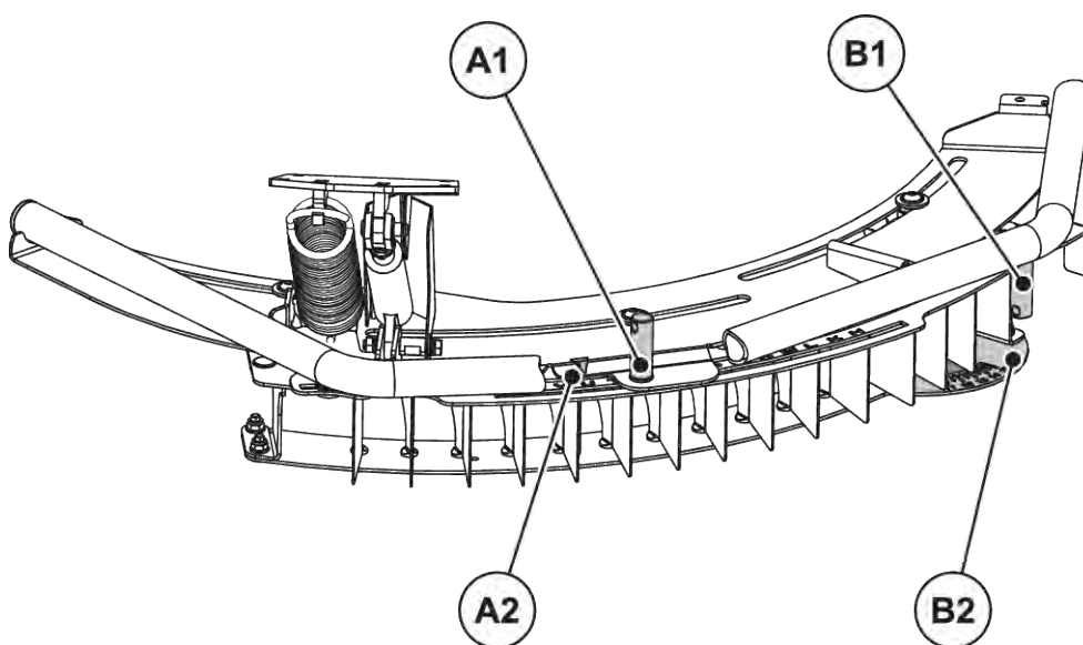
Σχ. 30: Ρύθμιση διάταξης TELIMAT
