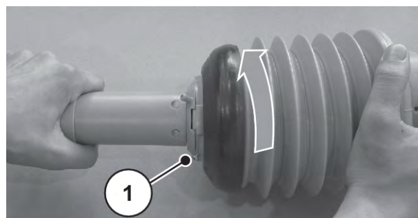
Фиг. 11: Развиване на защитата на карданныя вал
