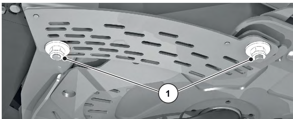
Фиг. 67: Закрепващи винтове на скалата
