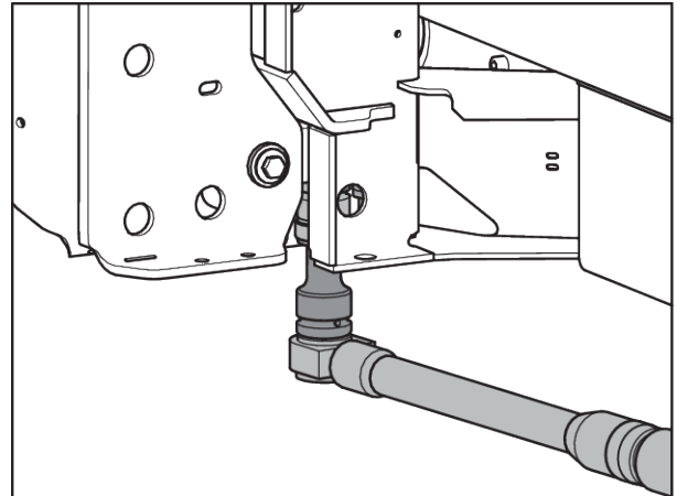
Rys. 48: Zamocowanie sensora wagi (w kierunku jazdy w lewo)
