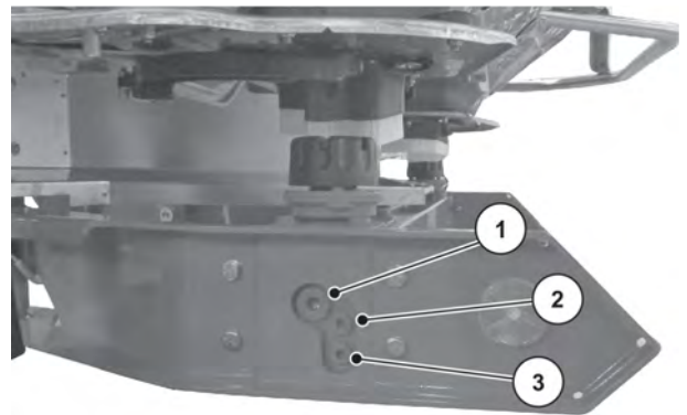
Rys. 67: Miejsca wlewania i spuszczenia oleju przekładniowego
