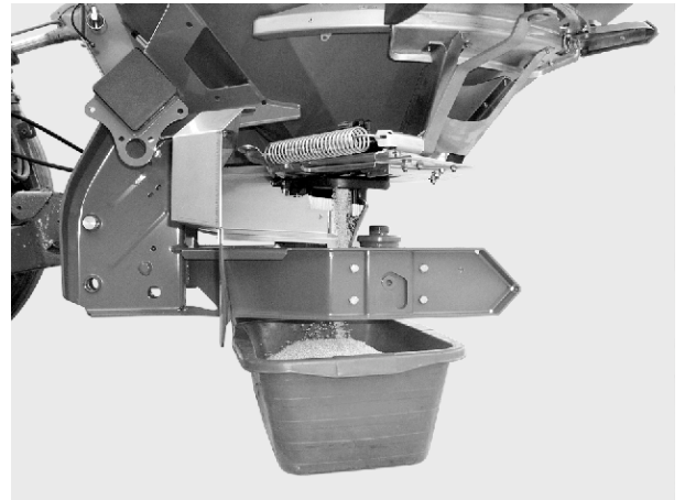
Rys. 45: Wykonanie próby rozsiewu
