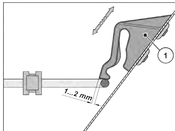
Rys. 53: Wymiar kontrolny do sprawdzania działania blokady kratki ochronnej
