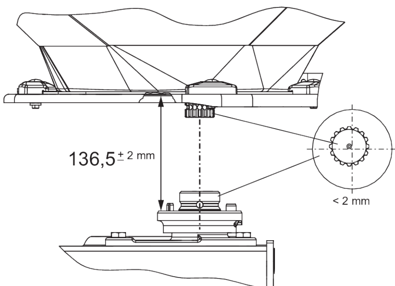
Rys. 55: Sprawdzenie położenia piasty tarcz rozrzucających
