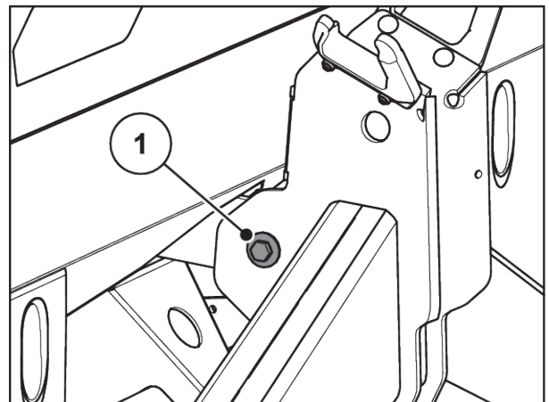
Rys. 53: Mocowanie ciągła do ramy wagi
