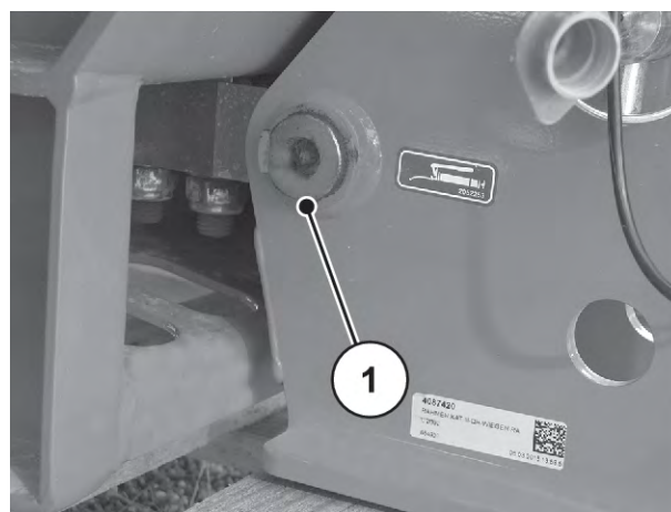
Rys. 73: Punkt smarowania rozsiwacza wagowego
