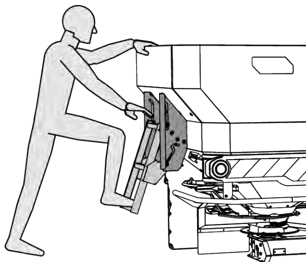
Rys. 48: Wchodzenie na drabinkę przy braku planeki na pojemniku
