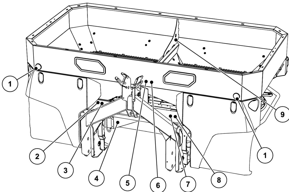
Rys. 4: Urządzenia zabezpieczające, naklejki wskazówek ostrzegawczych i informacyjnych, widok z przodu
