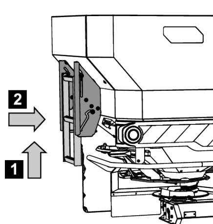
III. 51: Scaletta in posizione chiusa
