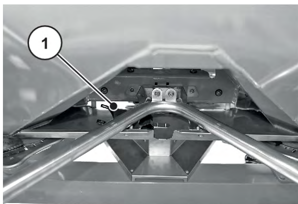
III. 42: Scivolo per il test di taratura
