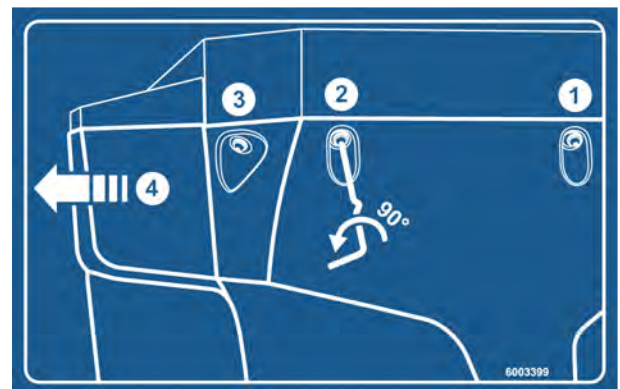
III. 58: Adesivo con istruzioni parasporca
