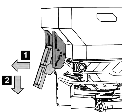
III. 50: Apertura della scaletta
