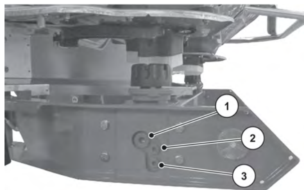
III. 71: Punti di rifornimento e scarico dell'olio del riduttore
