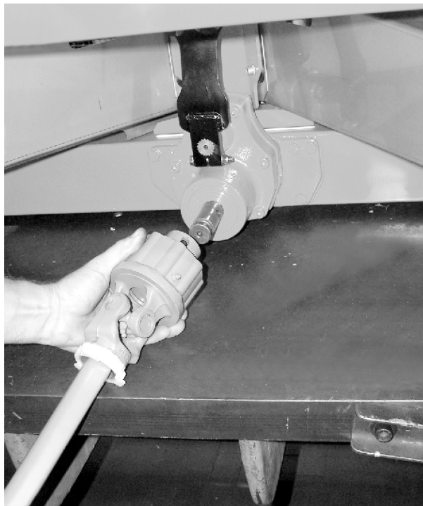
III. 12: Inserimento dell'albero cardanico sul perno del riduttore
