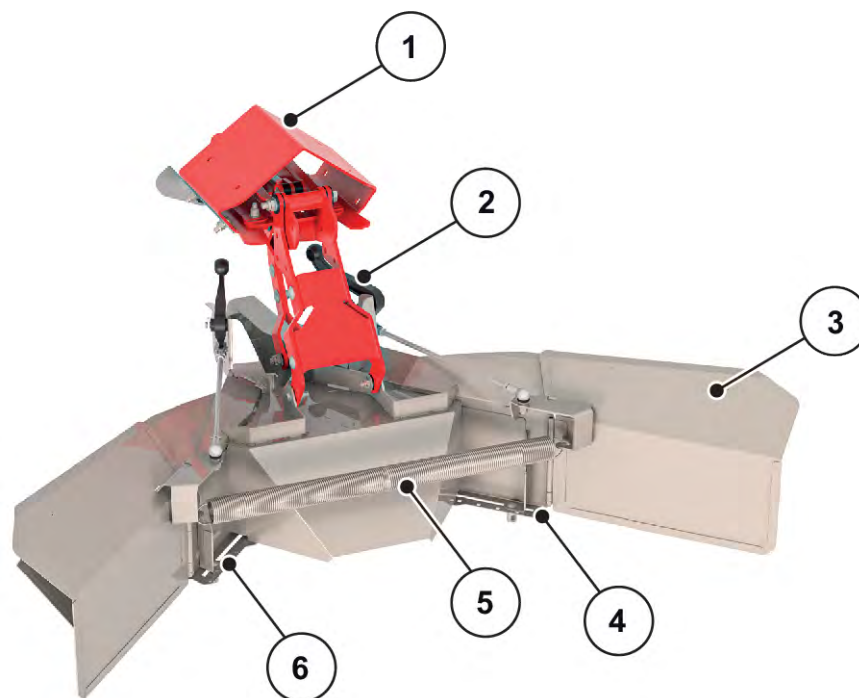
Abb. 29: Einstellung der Grenzstreueinrichtung
