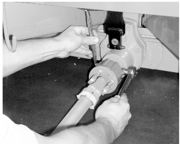
Abb. 13: Gelenkwelle befestigen
