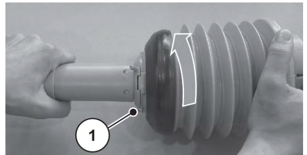
Abb. 11: Gelenkwellenschutz lösen
