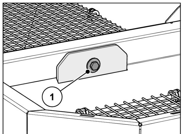
Abb. 50: Befestigung des Zugstabes im Behälter
