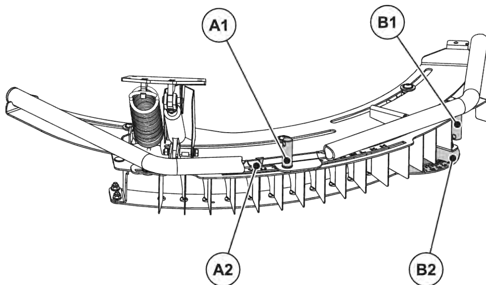
Abb. 30: TELIMAT Einrichtung einstellen
