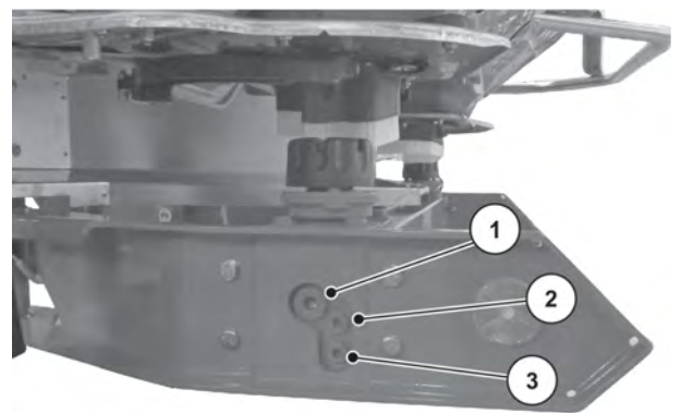
Abb. 67: Einfüll- und Ablassstellen für Getriebeöl
