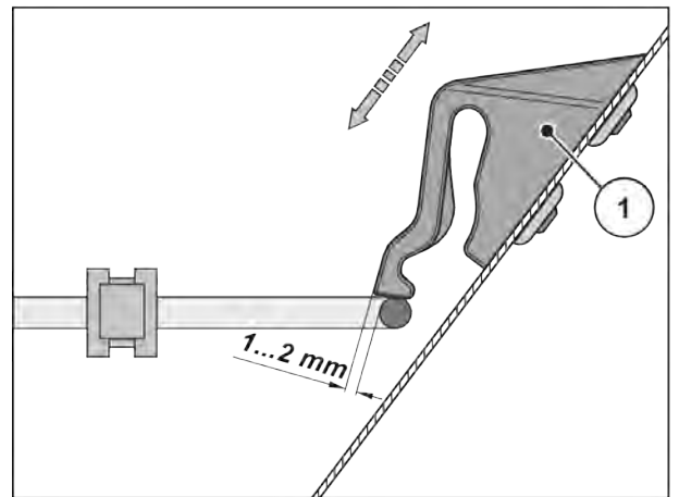
Abb. 53: Prüfmaß zur Funktionskontrolle der Schutzgitterverriegelung
