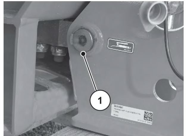
Abb. 69: Schmierstelle Wiegestreuer
