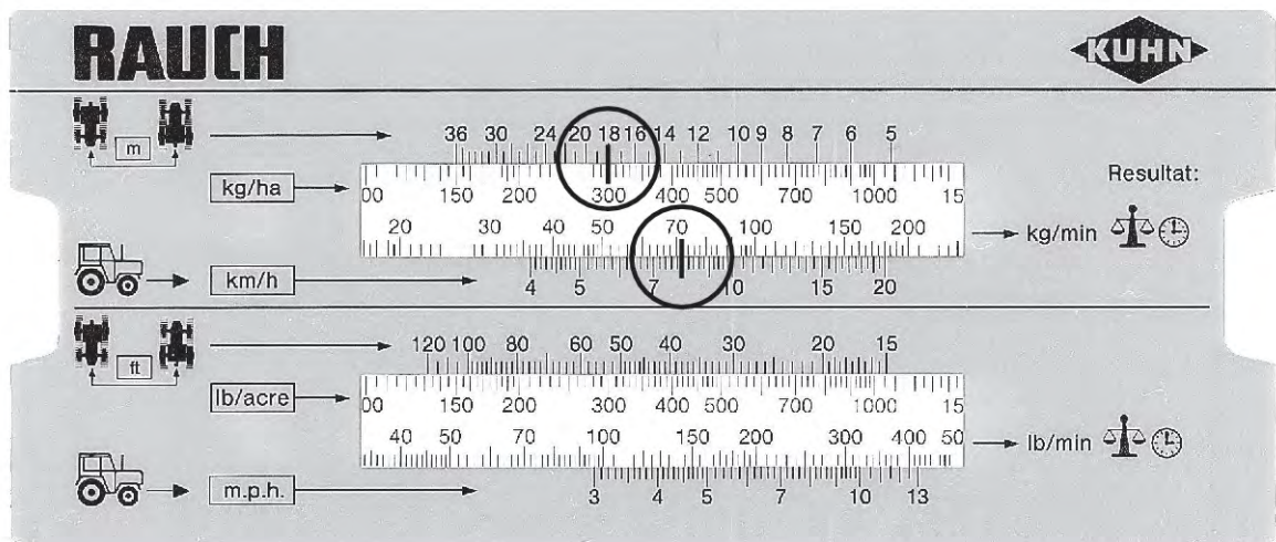
Abb. 41: Skala zur Ermittlung der Soll-Auslaufmenge pro Minute
