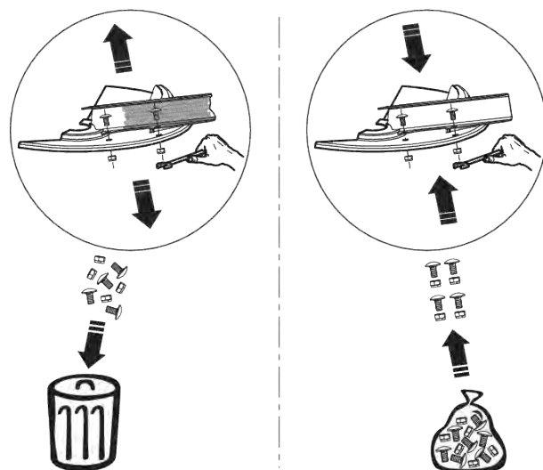
Sl. 65: Koristiti nove samoosiguravajuće navrtke
