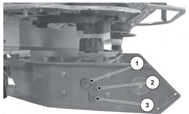
Sl. 72: Mesta za punjenje i ispuštanje ulja za prenosnike
