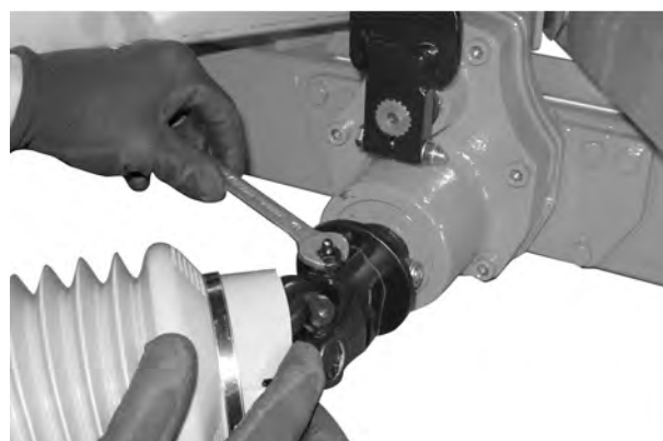
Sl. 15: Pritezanje priključka za podmazivanje
