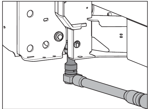
Sl. 53: Pričvršćivanje ćelije za vaganje (u smeru vožnje levo)
