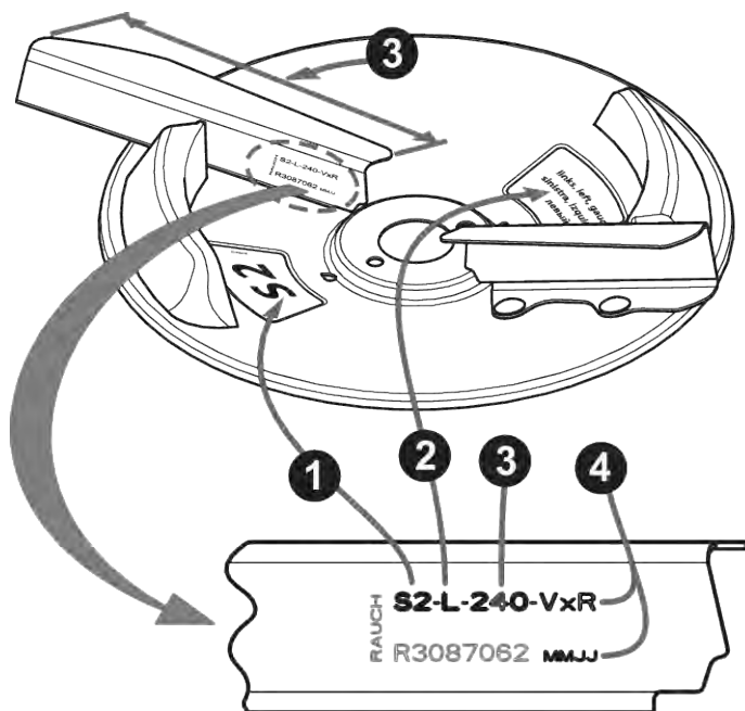
Sl. 63: Natpis na disku za rasipanje
