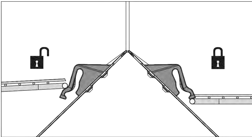
III. 56: Bloccaggio della griglia protettiva aperto/chiuso
