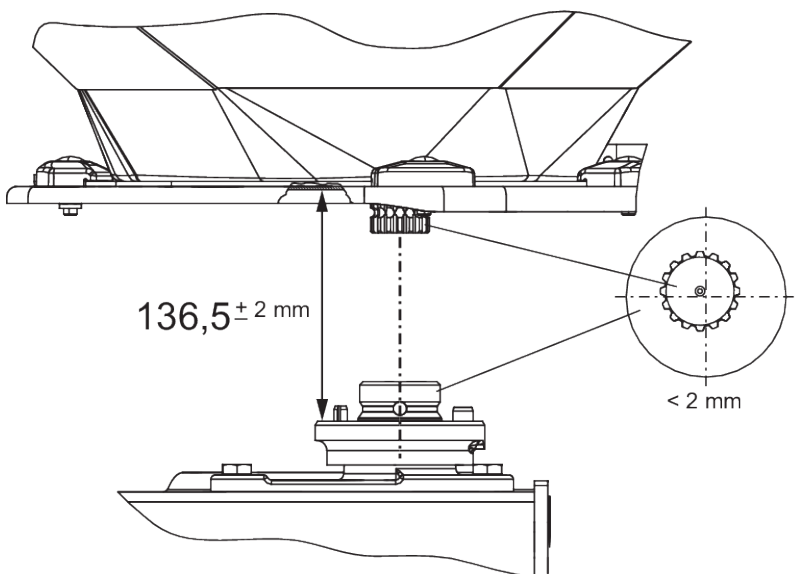
Ill. 60: Controllo della posizione del mozzo del disco di lancio
