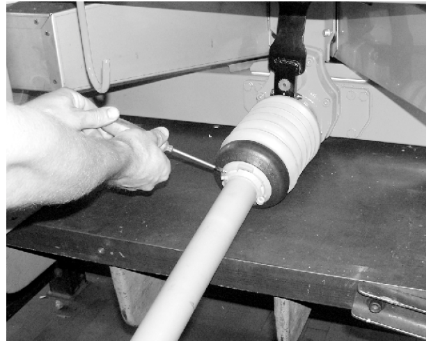
III. 17: Fissare la protezione dell'albero cardanico
