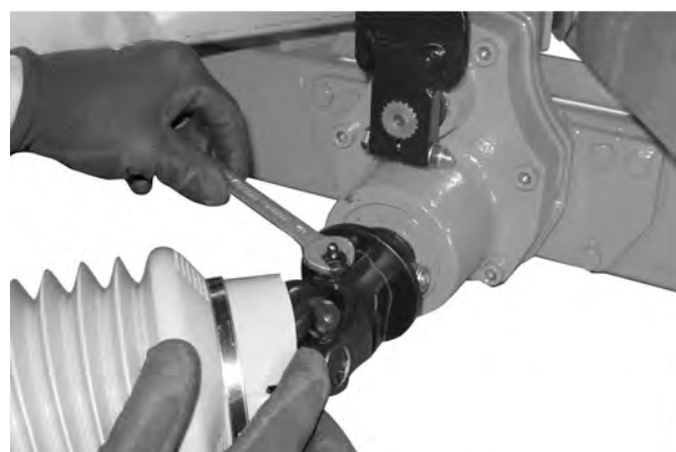
III. 15: Serraggio del raccordo per lubrificazione
