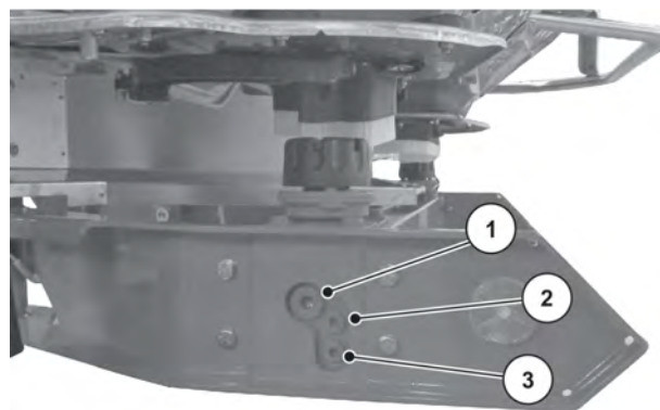
Ill. 72: Punti di rifornimento e scarico dell'olio del riduttore
