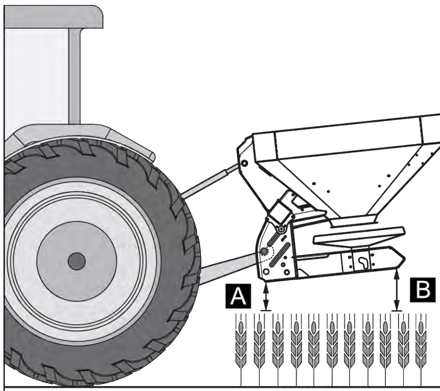
Ill. 26: Posizione e altezza di montaggio nella concimazione tardiva
