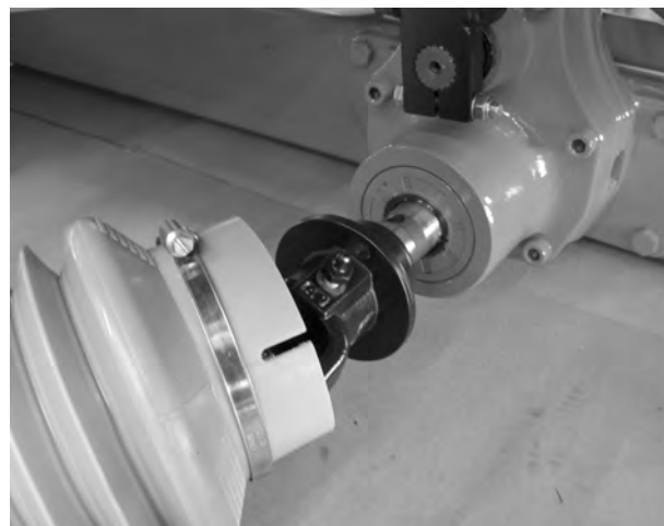
III. 13: Inserimento dell'albero cardanico sul perno del riduttore
