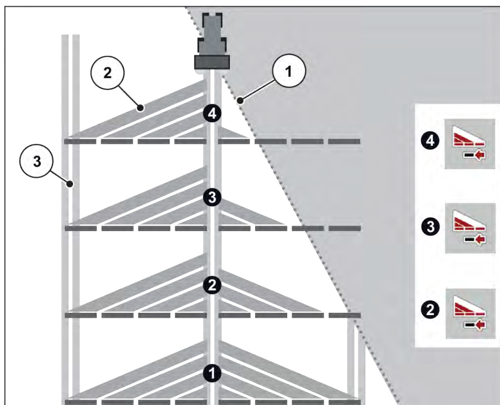
Ill. 44: Esempio di attivazione delle larghezze laterali
