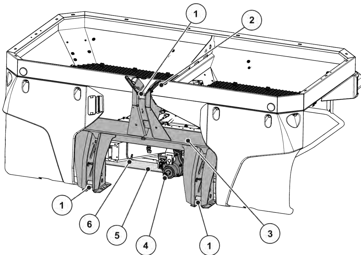
Att. 5: Konstruktijas grupu pārskats: Priekšpuse
