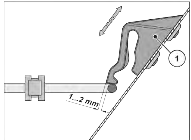
Att. 57: Pārbaudes mērs aizsargrežģa fiksatora darbības pārbaudei
