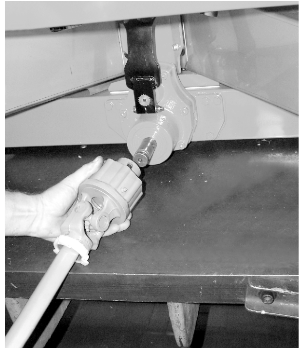
Att. 17: Kardānvārpstas uzbīdīšana uz pārvada vārpstas kakla
