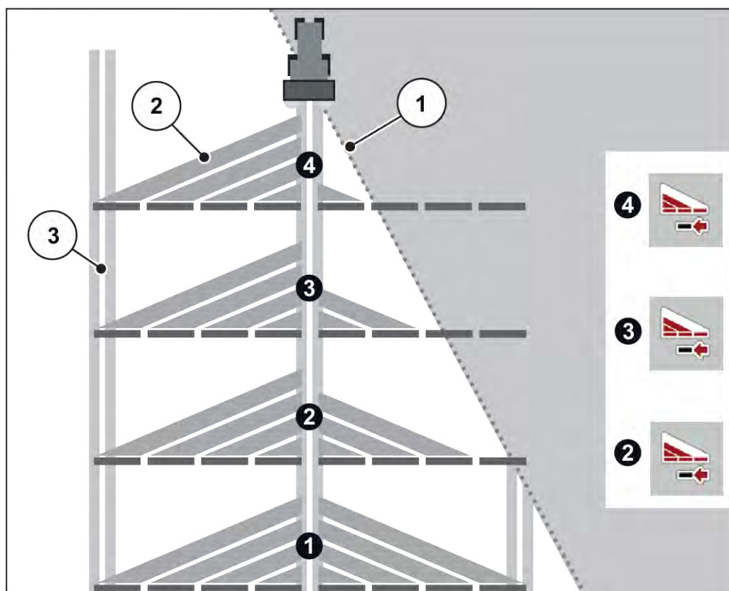
Att. 43: Piemērs daļējā platuma mainīšanai
