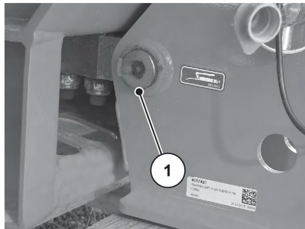
Att. 73: Eļļošanas vieta izkliedētājam ar svariem
