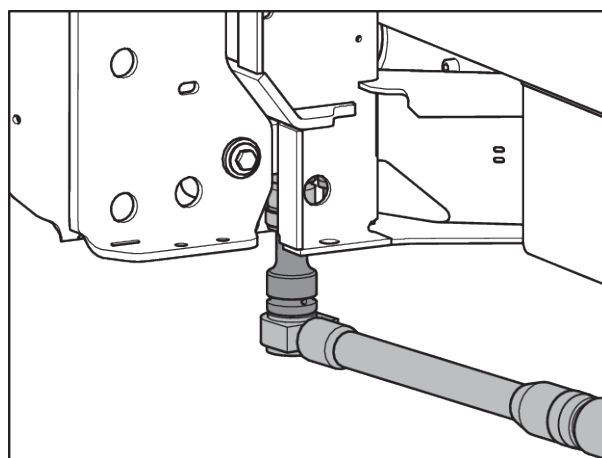
Att. 52: Tenzodevēja piestiprināšana (braukšanas virzienā kreisajā pusē)
