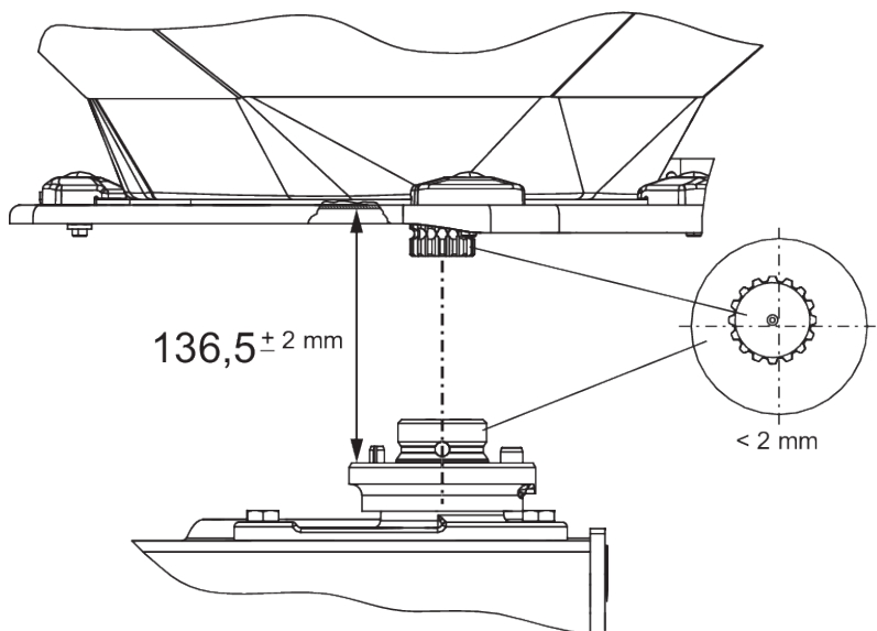
Att. 59: Izkliešanas diska rumbas pozīcijas pārbaude
