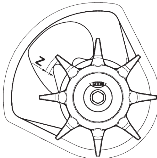
Att. 61: Maisītāja galvas nodiluma zona
