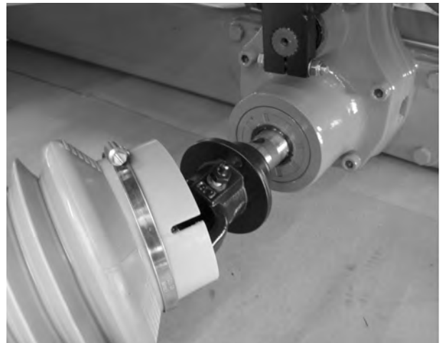
Att. 12: Kardānvārpstas uzbīdīšana uz pārvada vārpstas kakla
