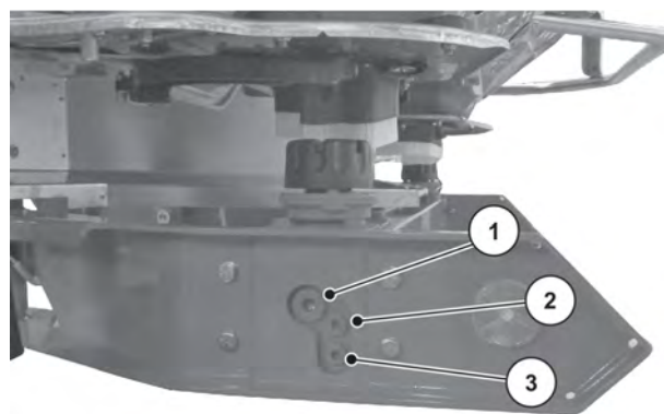
Att. 71: Transmisijas eļļas iepildīšanas un iztecinašanas vietas
