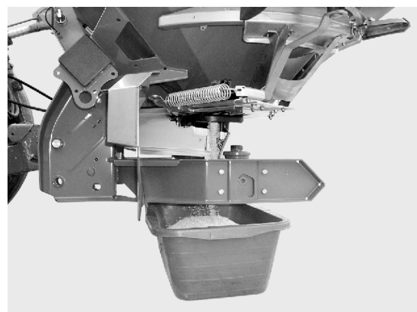
Att. 49: Dozēšanas izmēģinājuma veikšana
