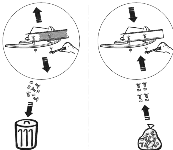
Att. 64: Izmantojiet jaunus pašfiksējošos uzgriežņus
