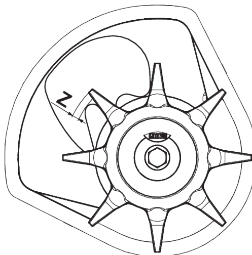
Fig. 61: Omrörarhuvudets slitageområde.
