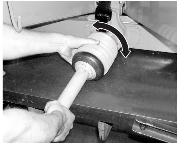
Fig. 15: Sätta dit kraftöverföringsaxelns skydd
