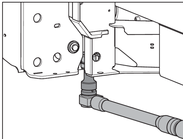
Sl. 52: Pričvršćivanje mjerne ćelije za vaganje (u smjeru vožnje lijevo)
