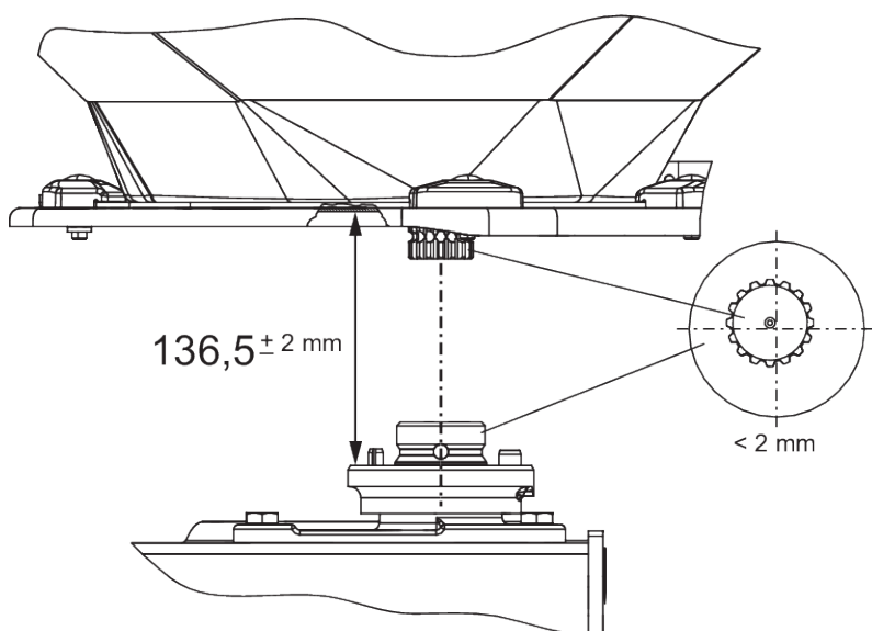
Ilust. 59: Comprobar la posición del cubo de disco de dispersión
