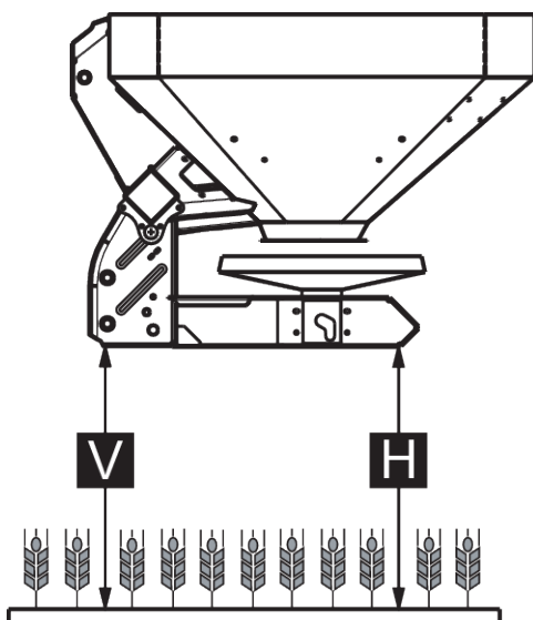
Ilust. 23: Altura de montaje máxima permitida en el abonado normal y tardío
