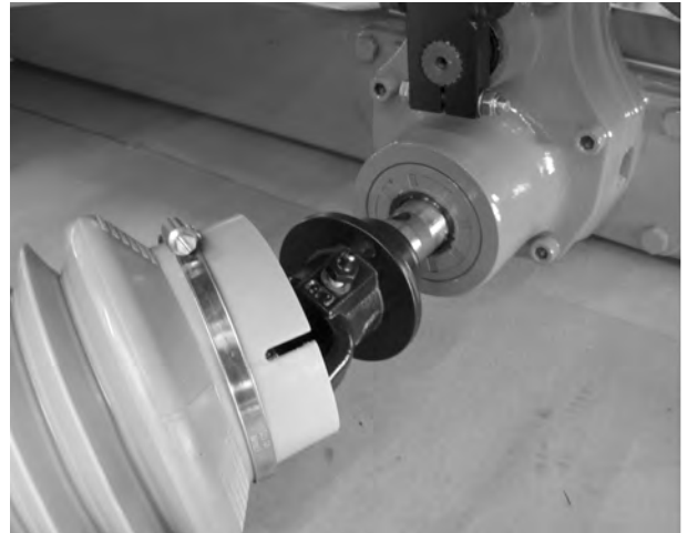
Ilust. 12: Insertar el eje articulado en el muñón de engranaje
