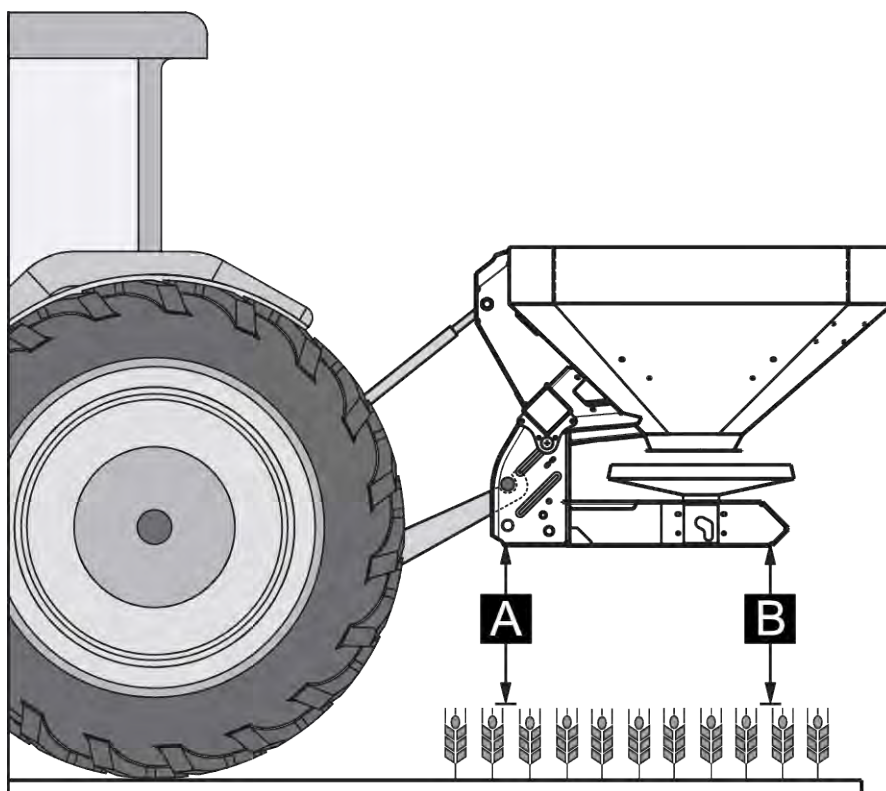
Ilust. 24: Posición y altura de montaje para el abonado normal
