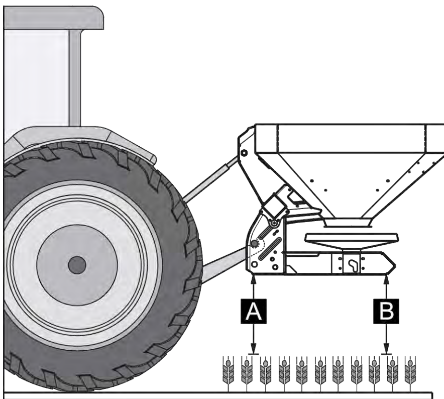
Ilust. 22: Posición de montaje
