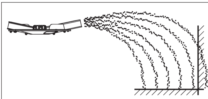
Ilust. 29: Dispersión de margen en el abonado normal
