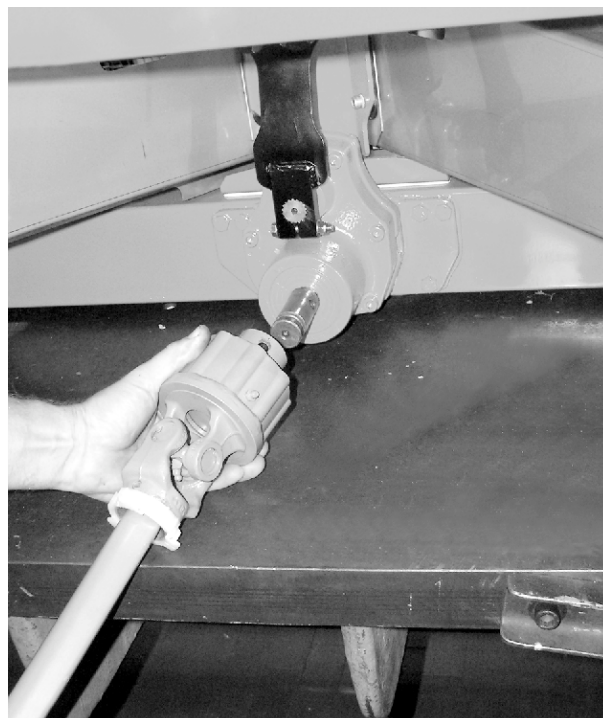
Ilust. 17: Inserción del eje articulado en el muñón de engranaje
