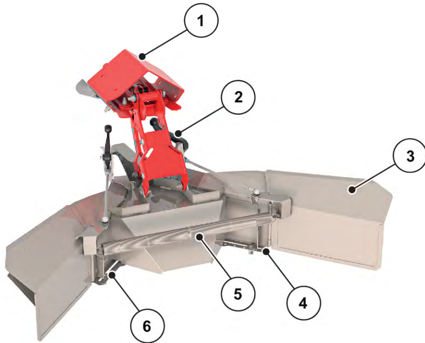
Рис. 33: Налаштування обмежувача ширини розкидання
