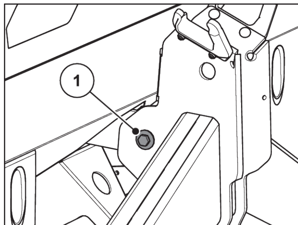
Рис. 53: Кріплення натяжної штанги на рамі ваг
