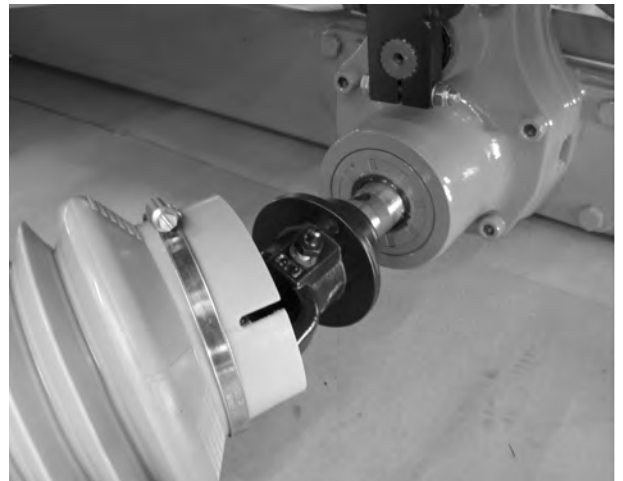
Рис. 12: Встановлення карданного вала на цапфу редуктора
