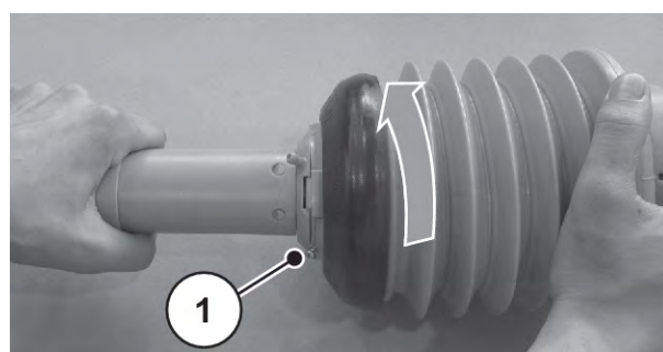
Рис. 10: Ослаблення кожуха карданного вала
