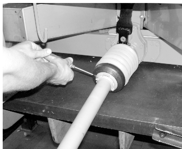
Рис. 16: Кріплення кожуха карданного вала
