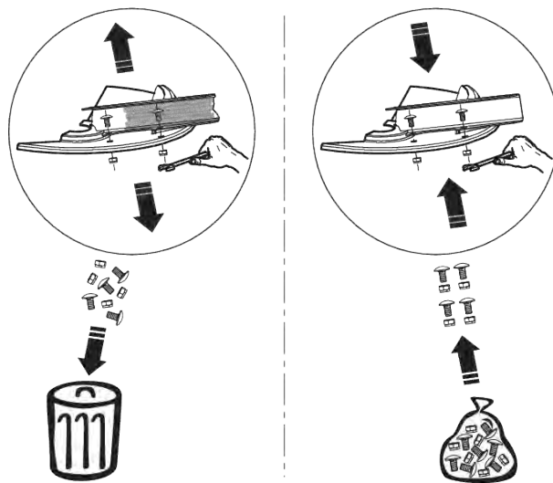
Kuva 64: Uusien itselukittuvien mutterien käyttö
