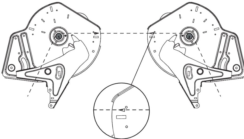
Kuva 69: Luovutuspisteasetuksen tarkistus
