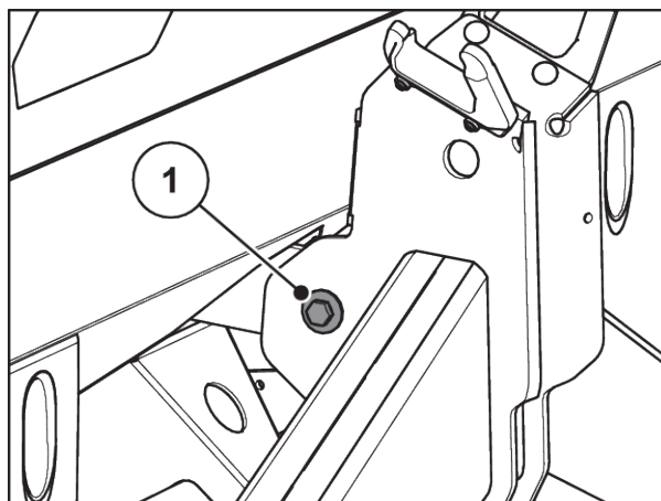
Sl. 53: Pričvršćivanje vučne šipke na okvir za vaganje
