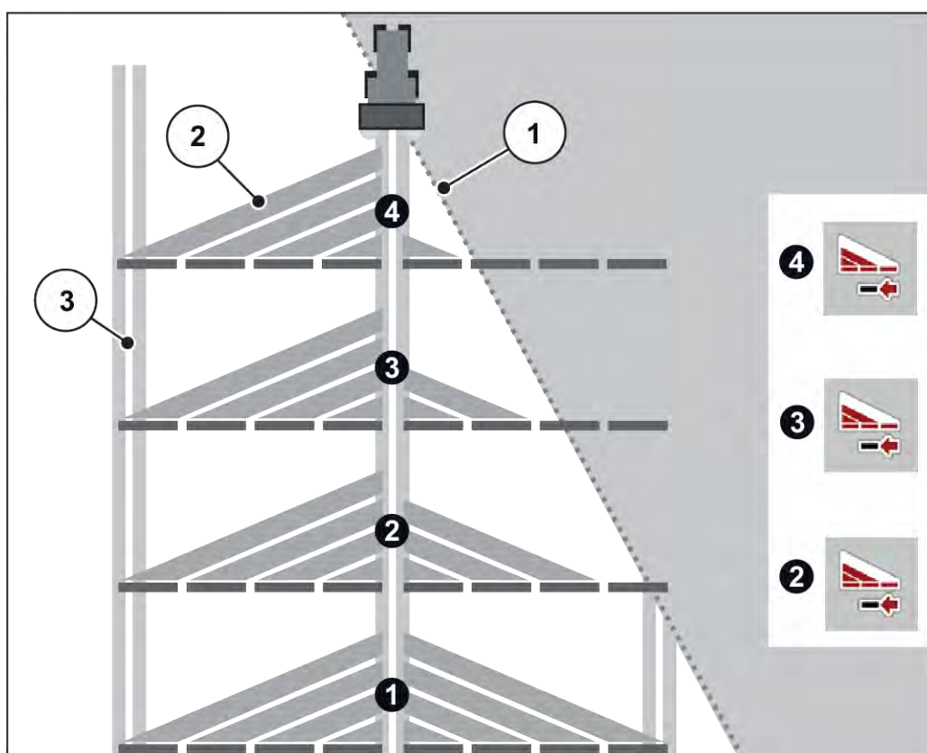
Sl. 43: Primer prebacivanja širine sekcije
