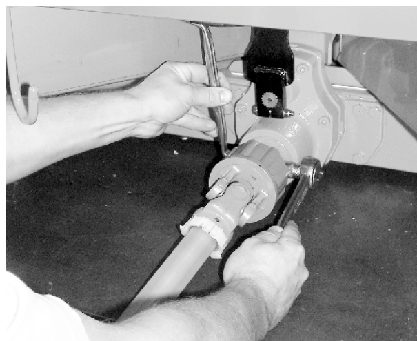
Sl. 18: Pričvršćivanje zglobnog vratila
