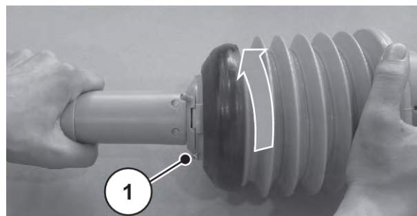
Sl. 10: Otpuštanje zaštite zglobnog vratila
