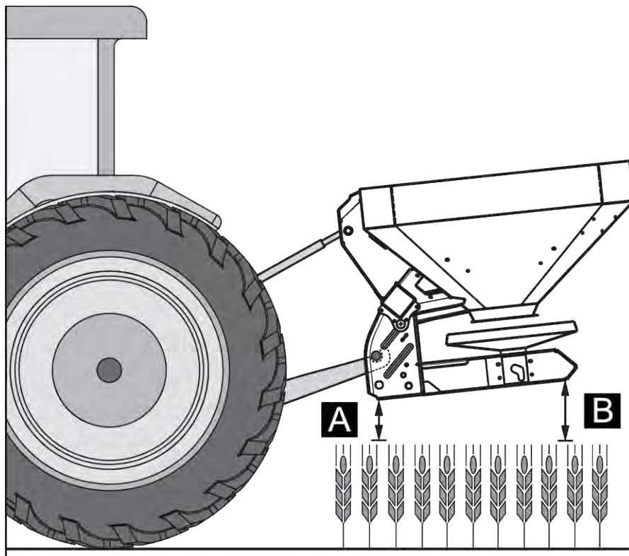
Ilust. 25: Posição e altura de montagem na fertilização tardia
