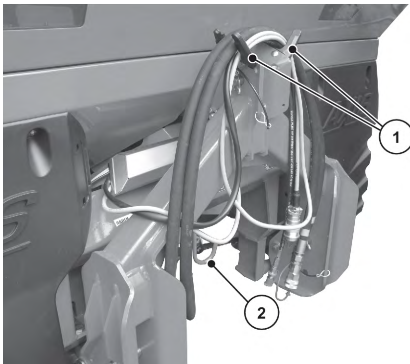
Ilust. 51: Deposição dos cabos e das mangueiras hidráulicas
