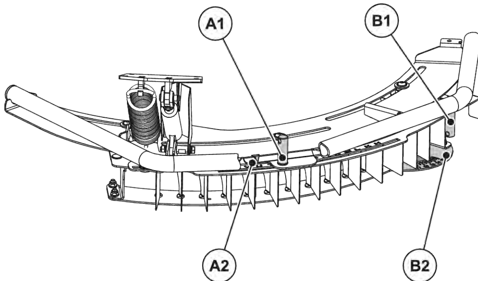
Ilust. 34: Ajustar o dispositivo TELIMAT
