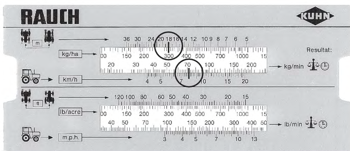
Ilust. 45: Escala para a determinação da quantidade nominal de saída por minuto
