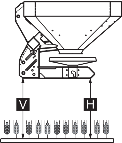
Ilust. 23: Altura de montagem máxima permitida na fertilização normal e tardia
