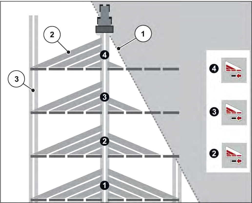
Ilust. 43: Exemplo de comutação de larguras parciais
