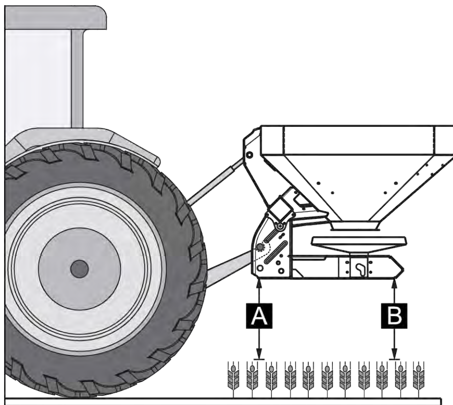
Afb. 24: Aanbouwpositie en -hoogte in de normale bemesting
