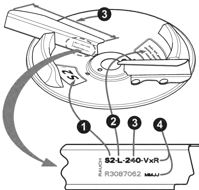
Afb. 62: Opschrift strooischijf
