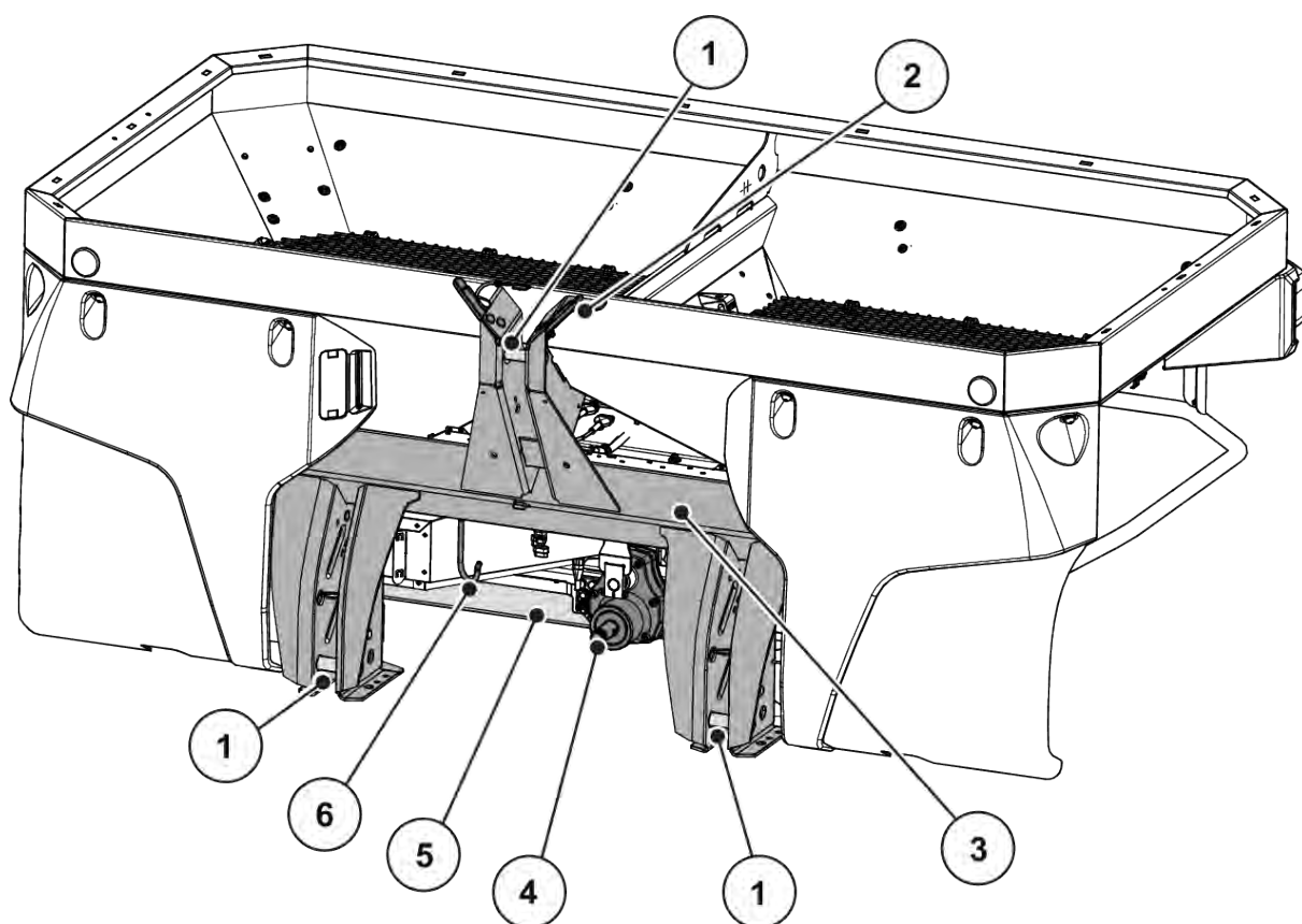
Afb. 5: Module-overzicht: Voorzijde
