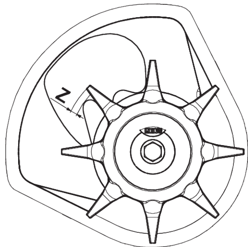
Afb. 61: Slijtagezone van de roerkop
