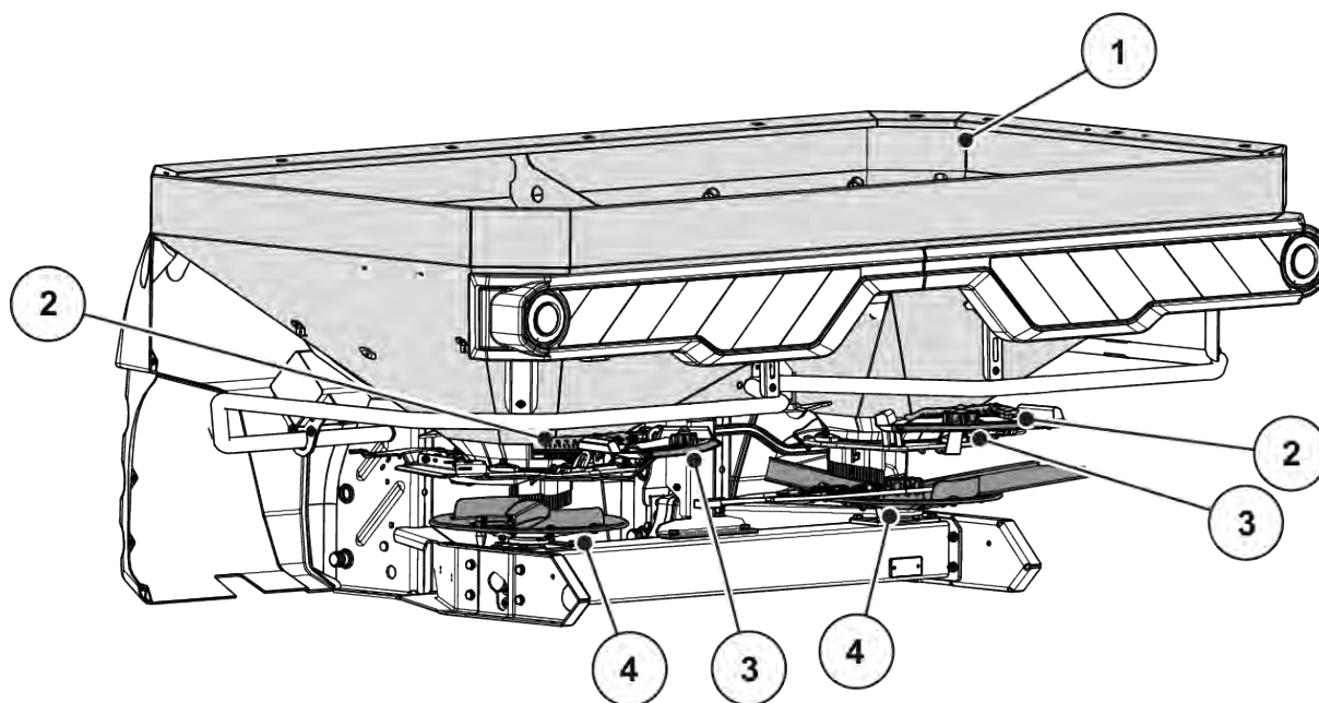
Fig. 6: Prezentare generală a subansamblurilor: Partea din spate
