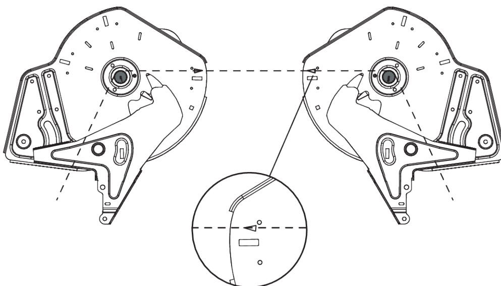
III. 69: Controllo della regolazione del punto di applicazione
