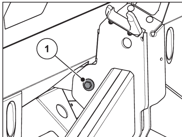
III. 53: Fissaggio della barra di trazione al telaio di pesatura
