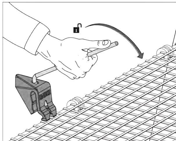
III. 56: Apertura del bloccaggio della griglia protettiva
