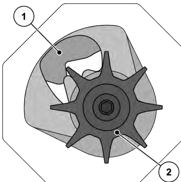
III. 8: Agitatore
