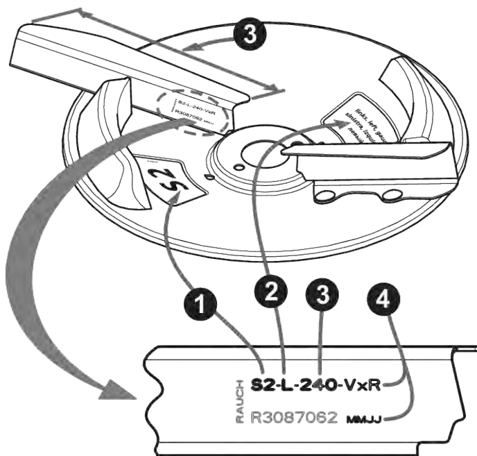
III. 62: Indicazione del tipo di disco di lancio
