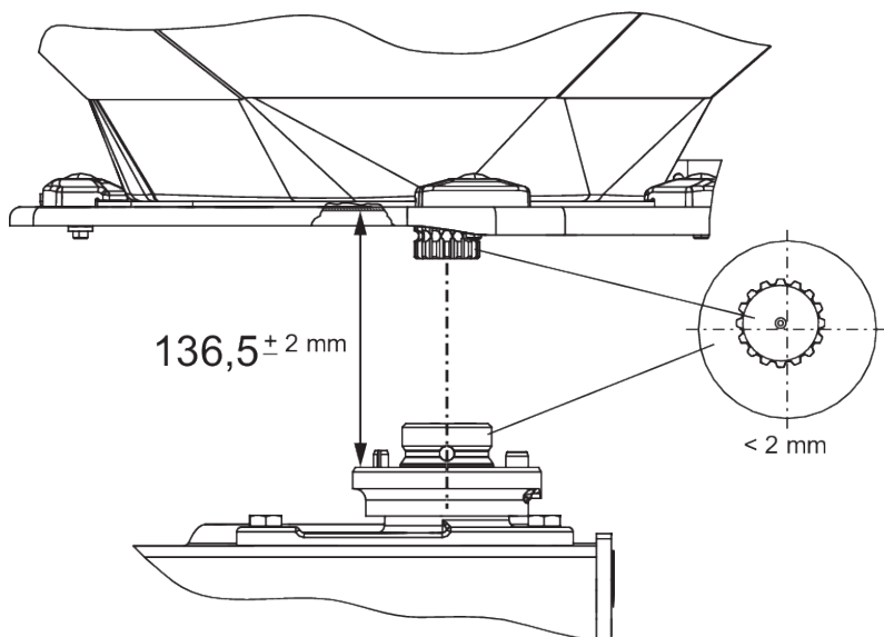
Ill. 59: Controllo della posizione del mozzo del disco di lancio
