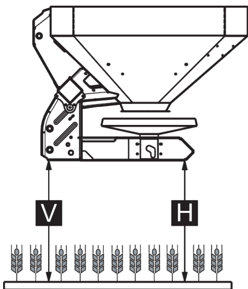
Ill. 23: Altezza di montaggio massima ammessa nella concimazione normale e tardiva
