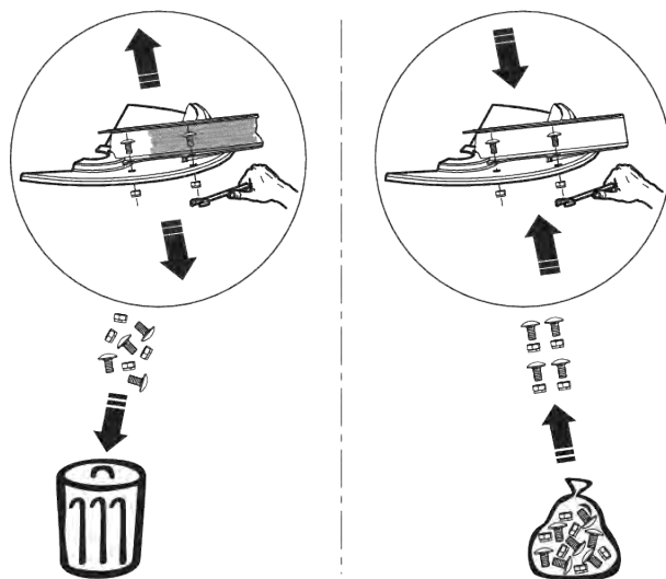
III. 64: Utilizzo di dadi autobloccanti nuovi
