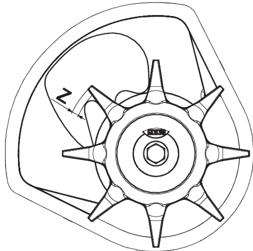
III. 61: Limite di usura della testa dell'agitatore
