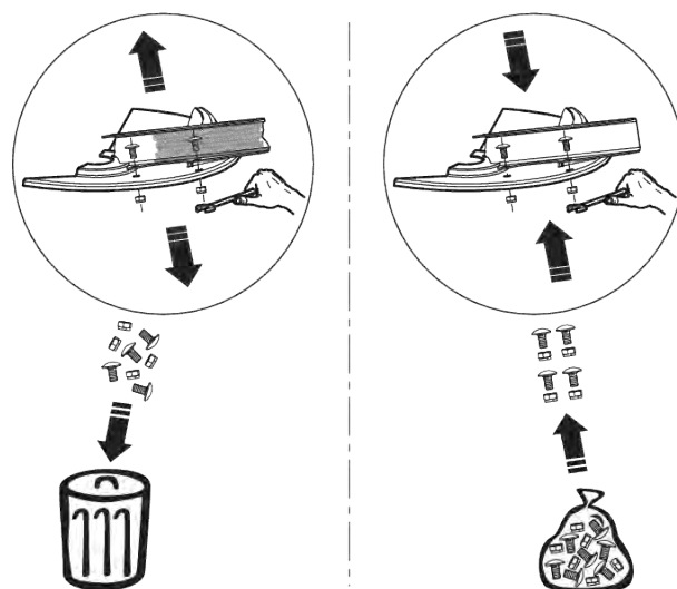
Fig. 64: Utiliser de nouveaux écrous autobloquants
