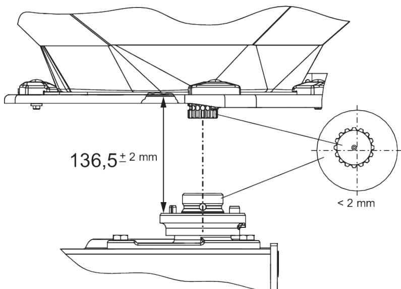
Abb. 59: Lage der Wurfscheibennabe prüfen
