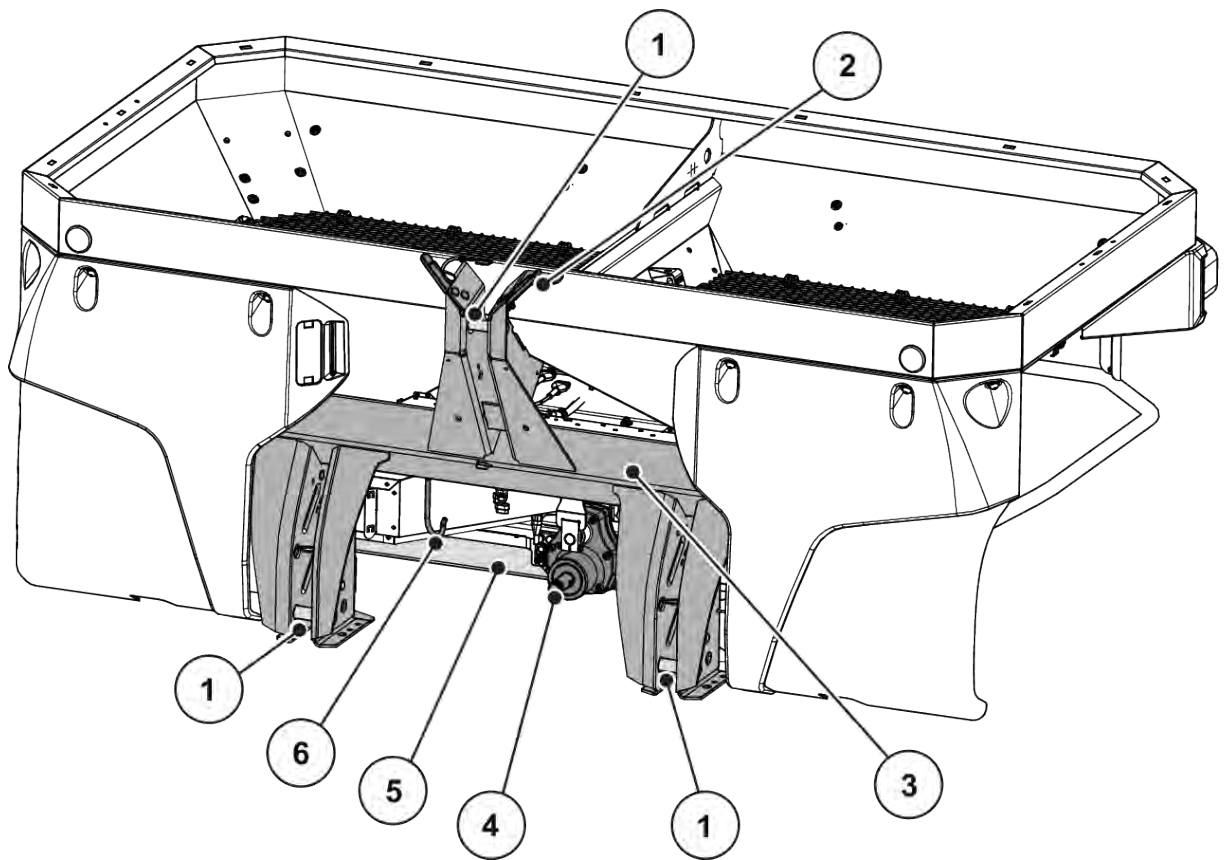
Abb. 5: Baugruppenübersicht: Vorderseite
