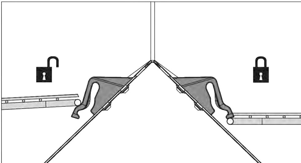
Abb. 55: Schutzgitterverriegelung offen/geschlossen
