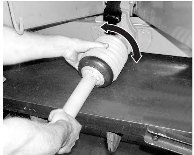
Abb. 19: Gelenkwellenschutz anlegen
