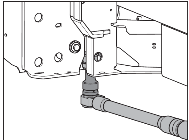
Abb. 52: Befestigung der Wiegezeile (in Fahrtrichtung links)
