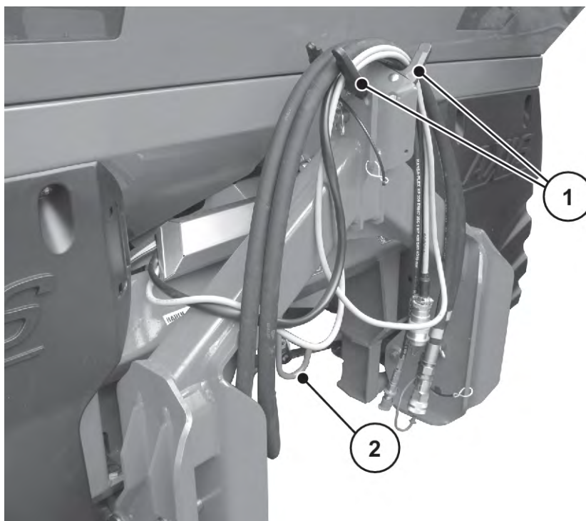
Abb. 51: Ablage der Kabel und Hydraulikschläuche
