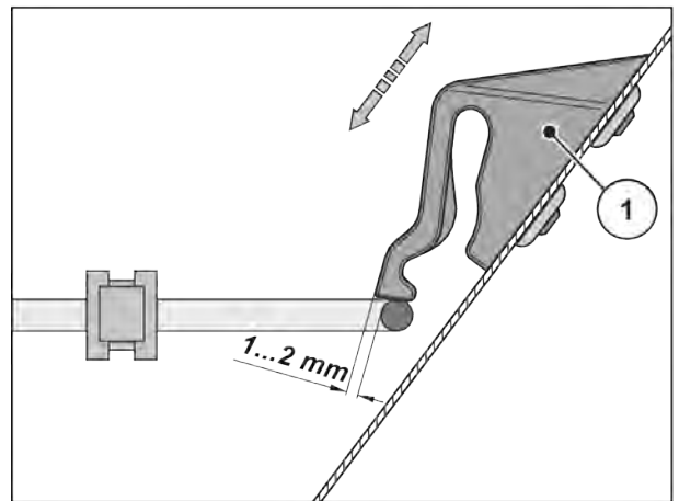
Abb. 57: Prüfmaß zur Funktionskontrolle der Schutzgitterverriegelung
