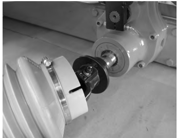
Abb. 12: Gelenkwelle auf Getriebezapfen aufstecken
