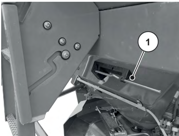
Abb. 36: Lage des Einstellhebels AXIS xx.2
