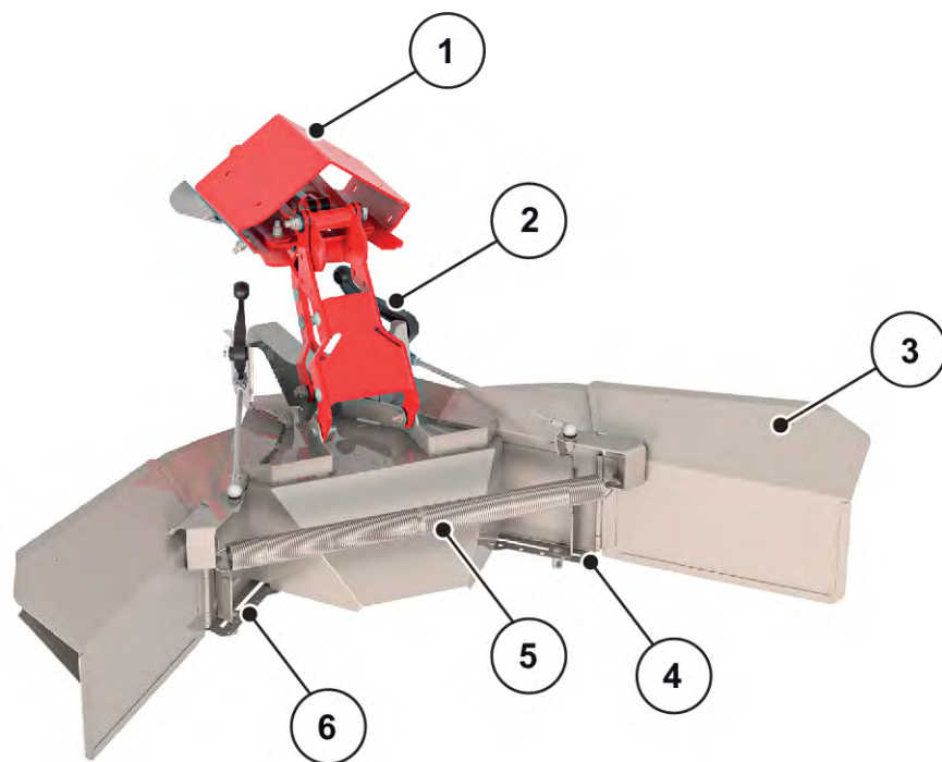
Abb. 33: Einstellung der Grenzstreueinrichtung
