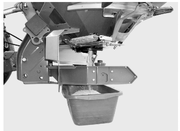
Abb. 49: Abdrehprobe durchführen
