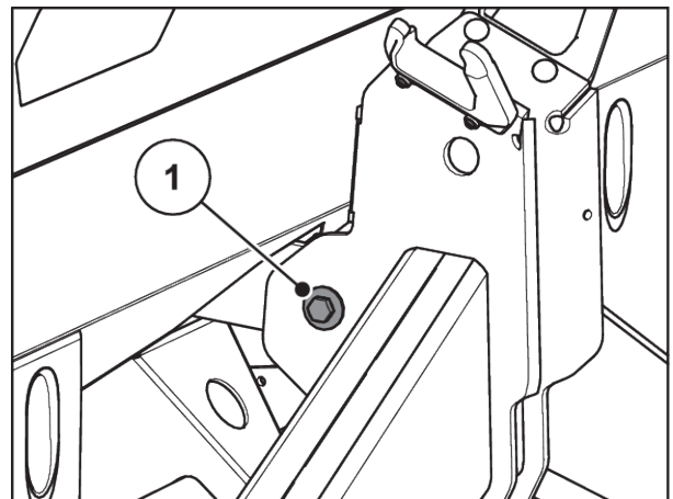
Abb. 53: Befestigung des Zugstabes am Wiegerahmen
