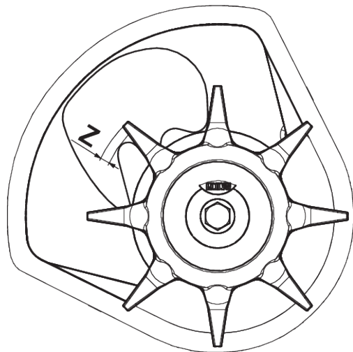
Abb. 61: Verschleißbereich des Rührkopfs
