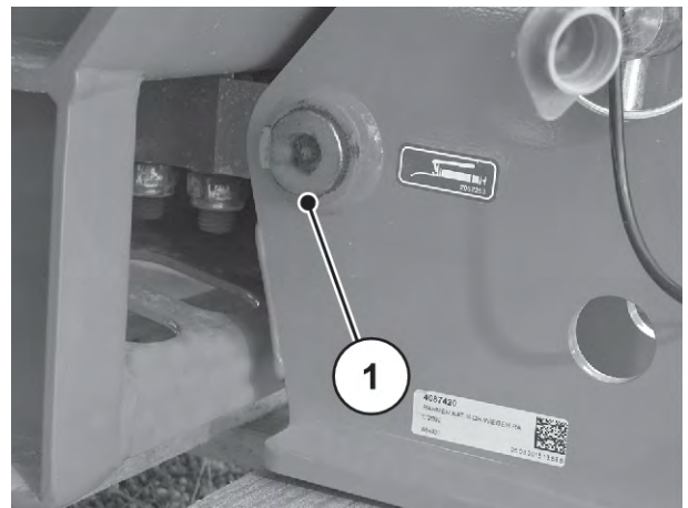
Abb. 72: Schmierstelle Wiegestreuer
