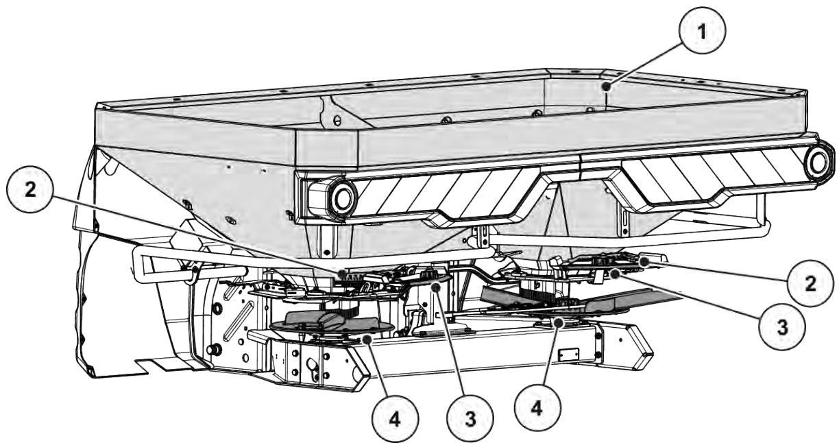
Abb. 6: Baugruppenübersicht: Rückseite
