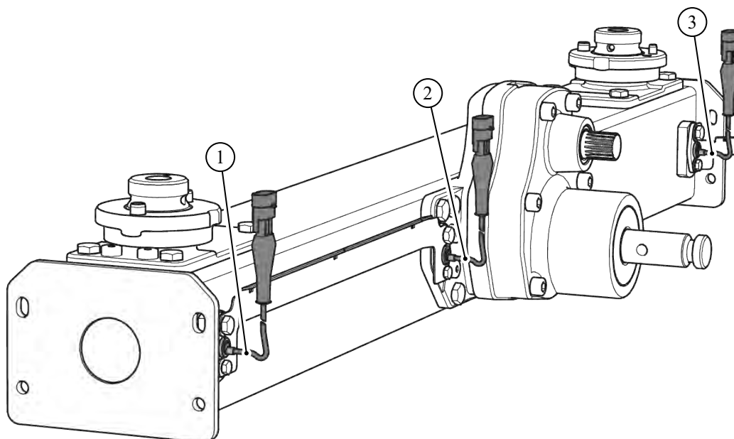
Abb. 7: Massenstromregelung durch Messung des Drehmoments der Wurfscheiben
