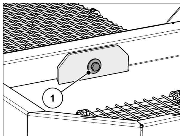
Рис. 47: Кріплення натяжної штанги на бункері
