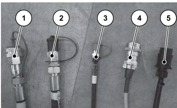
Sl. 13: Priključne napeljave iz metalnega trosilnika mineralnega gnojila
