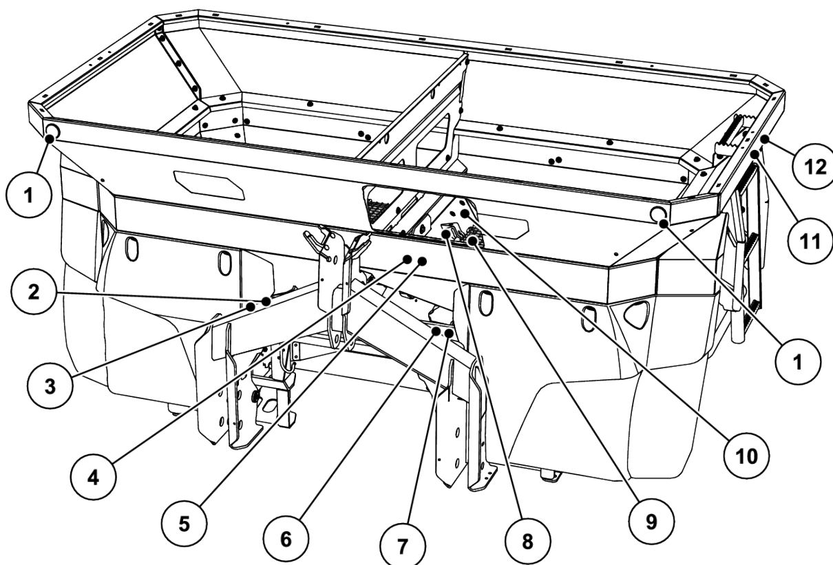
Jn. 2: Kaitseeadised, hoiatus- ja instruksioonijuhiste kleebsed, esikülg
