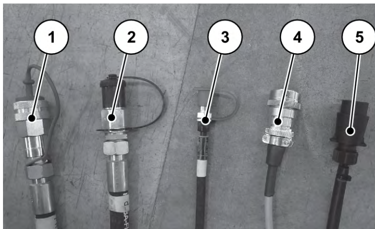
Att. 13: Centrbēdzes minerālmēslu izkļiedēja pieslēgšanas caurules
