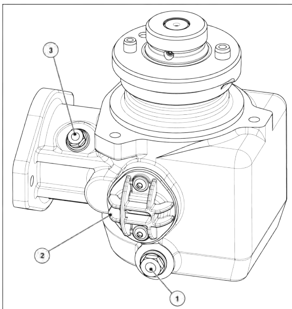
Att. 67: Transmisijas eļļas iepildīšanas un iztecināšanas vietas
