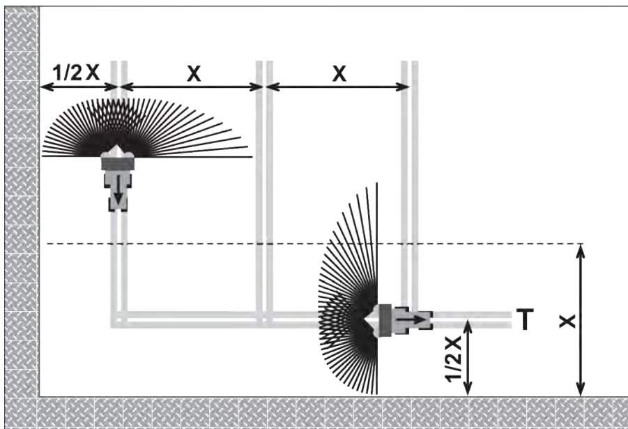
Att. 30: Izkliešana gar robežu
