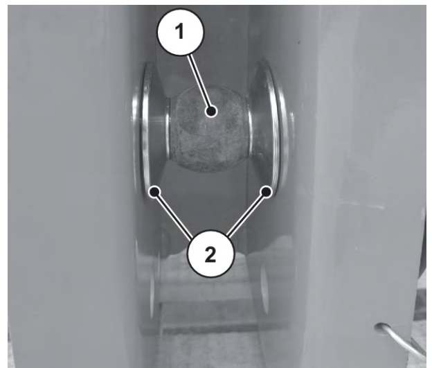
Att. 11: Distances starpliku pozīcija, uzkabīnot mašīnu
