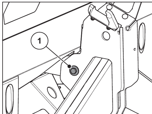
Att. 46: Spriegošanas stieņa stiprinājums pie svēršanas rāmja
