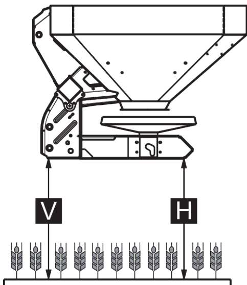
Att. 14: Maksimālais pieļaujamais uzkabināšanas augstums normālai un vēlī mēslošanai
