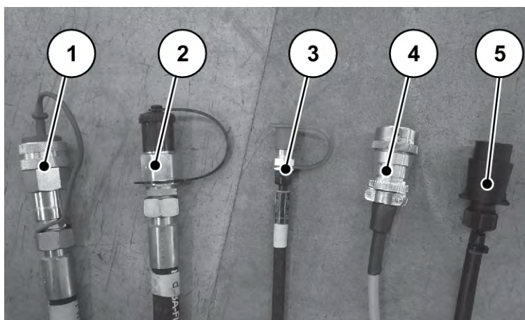
Att. 13: Centrālās minerālmēslu izkliedētāja pieslēgšanas caurules
