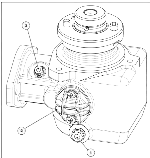
Att. 67: Transmisijas eļļas iepildīšanas un iztecinašanas vietas
