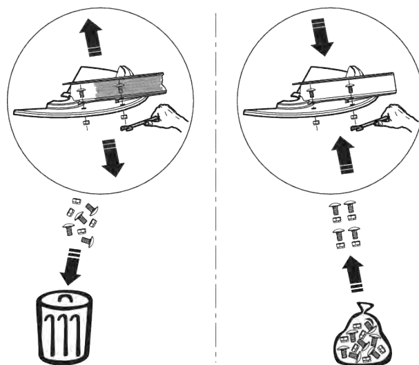
Att. 57: Izmantojiet jaunus pašfiksējošos uzgriežņus
