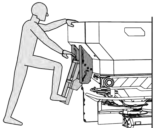
Pav. 41: Kopėčios be rezervuaro dengiamojo tento
