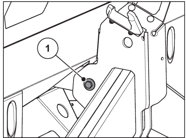
Pav. 46: Tempiamojo strypo tvirtinimas prie svėrimo sistemos rémo
