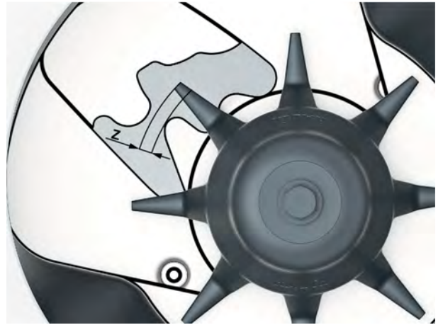
Pav. 54: Maišymo galvutės nudilimo riba
