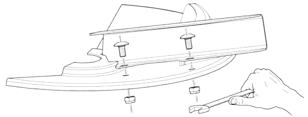
Фиг. 56: Разхлабете винтовете на разпръскващите лопатки
