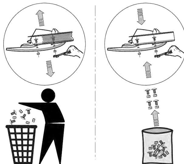
Фиг. 57: Използвайте нови самозаконтящи се гайки
