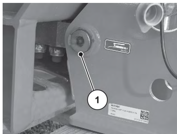
Фиг. 64: Точка на смазване Разпръсквачка с претегляща система
